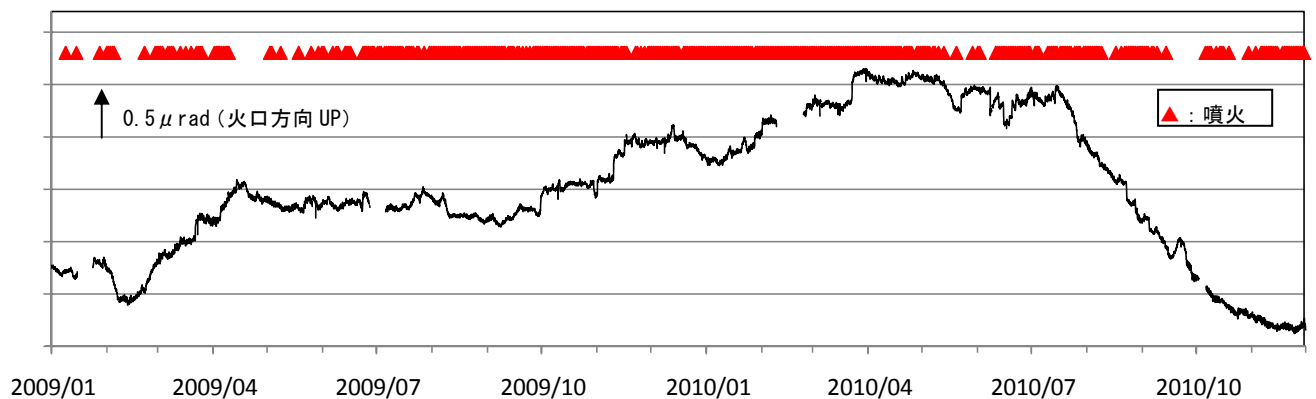
図 6 ※ 桜島 有村観測坑道の水管傾斜計の変化（2009 年 1 月～2010 年 11 月）
