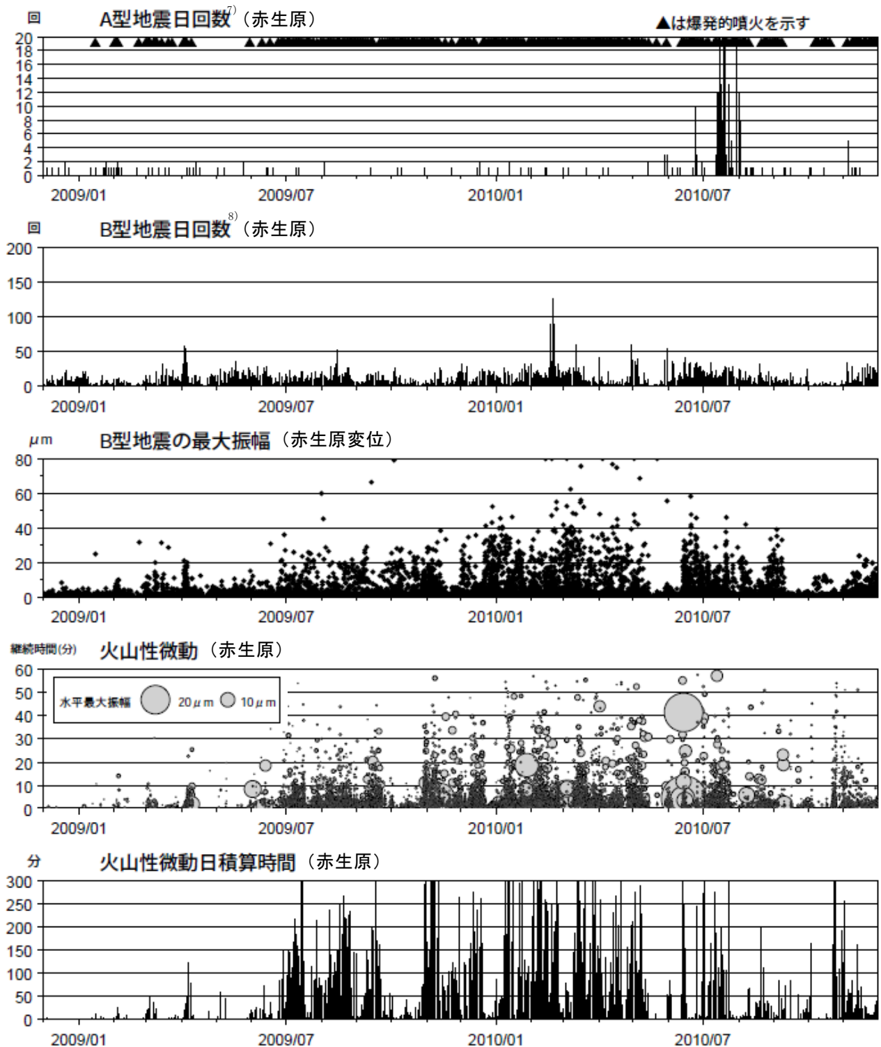
図 4 桜島 最近 2 年間の火山性地震、火山性微動（2008 年 12 月～2010 年 11 月） ＜11 月の状況＞
