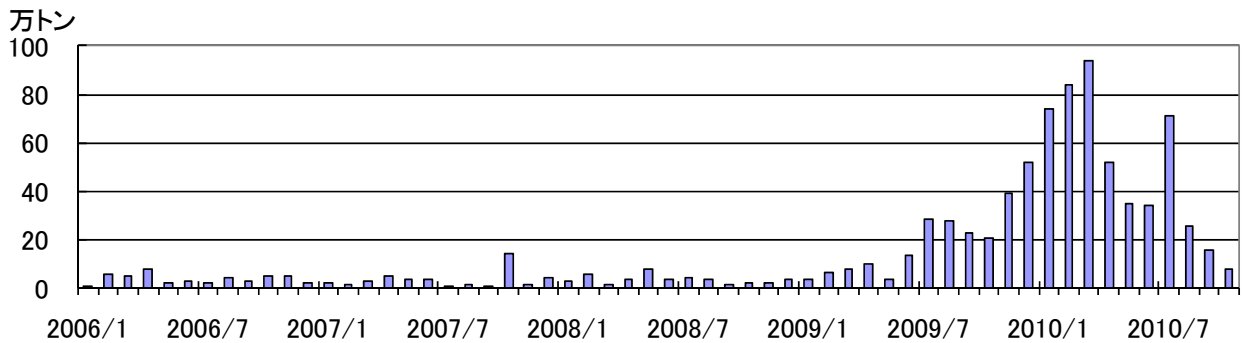
図 9※ 桜島 鹿児島県が実施している降灰量観測による月別降灰量 (2006 年 1 月～2010 年 10 月)
