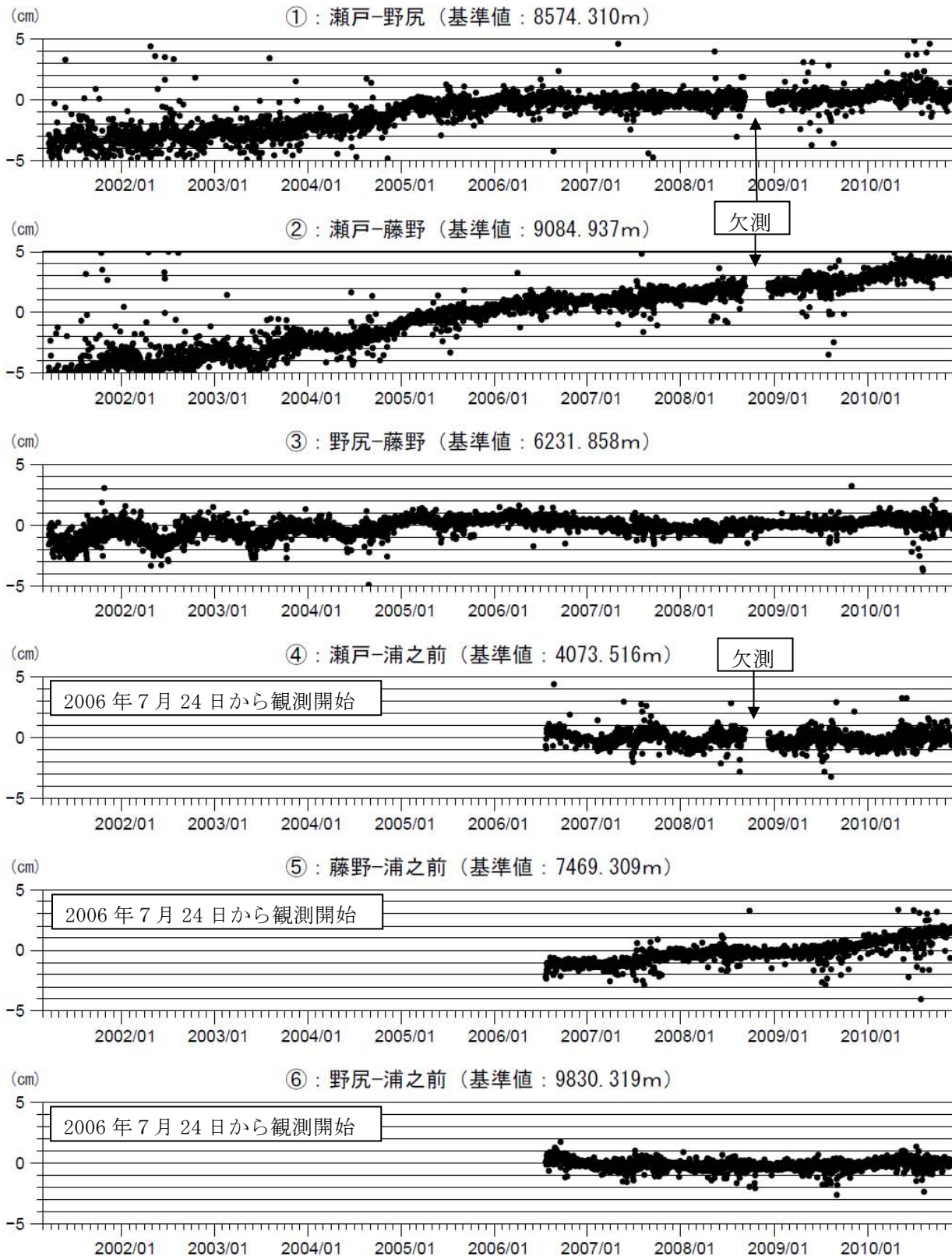
図 7 桜島 GPS 連続観測による長期の基線長変化（2001 年 3 月～2010 年 11 月）
