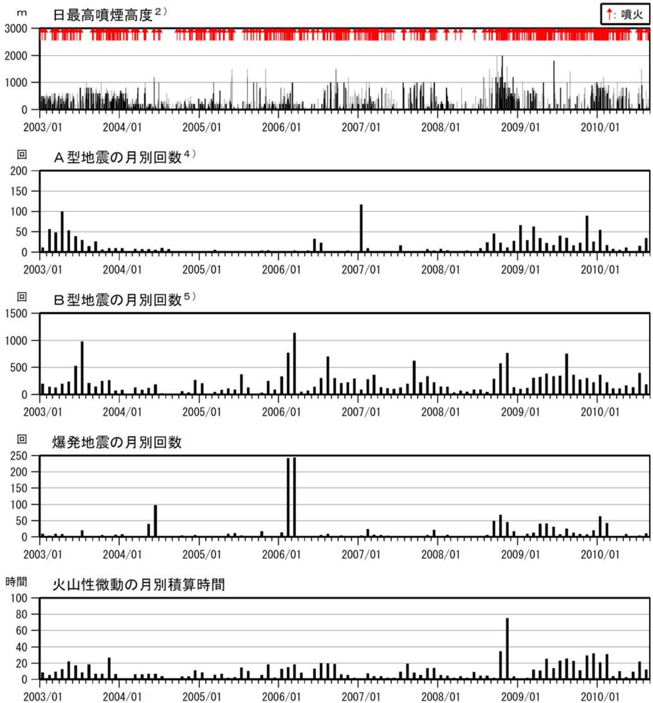
図 1 諏訪之瀬島 火山活動経過図（2003 年 1 月～2010 年 8 月）
