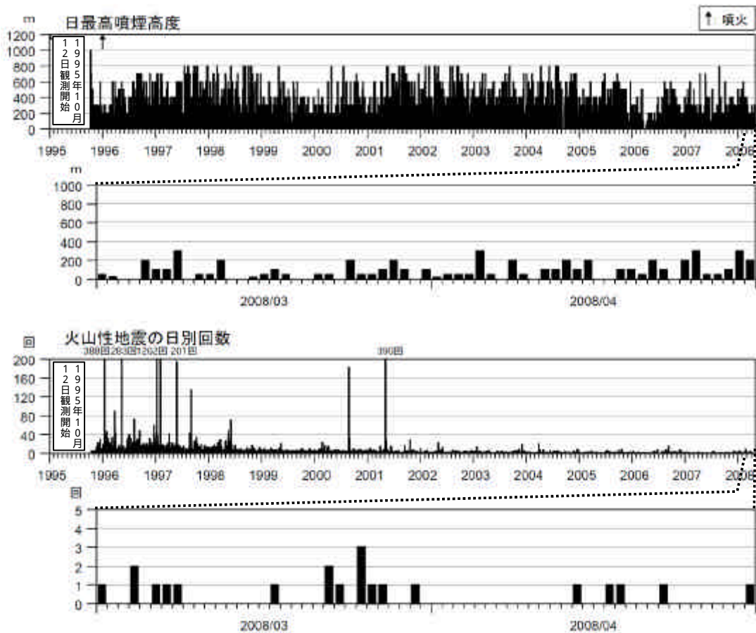
図 2 九重山 火山活動経過図(1995 年 10 月 12 日～2008 年 4 月 30 日)
