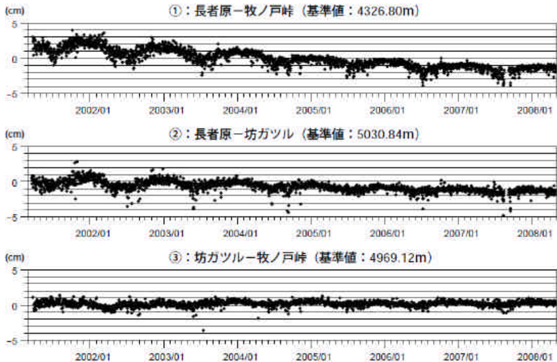
図 3 九重山 GPS 連続観測による基線長変化(2001 年 3 月～2008 年 4 月)
