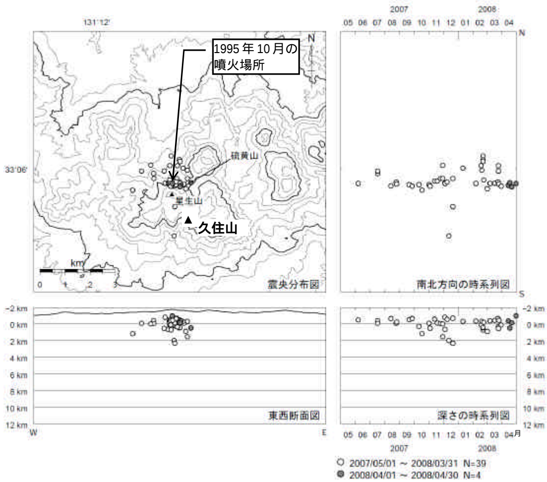
図 4 九重山 震源分布図(2007 年 5 月～2008 年 4 月) 2008 年 4 月は 4 個の震源が求まり、山体付近の浅い所に分布しました。
