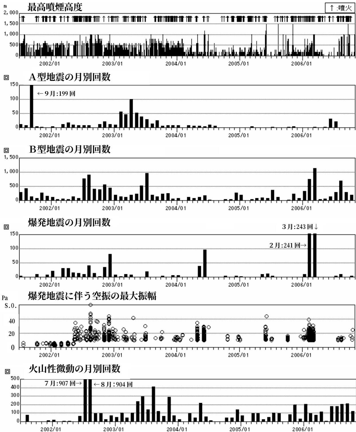
図2 火山活動経過図(2001年7月～2006年10月)
