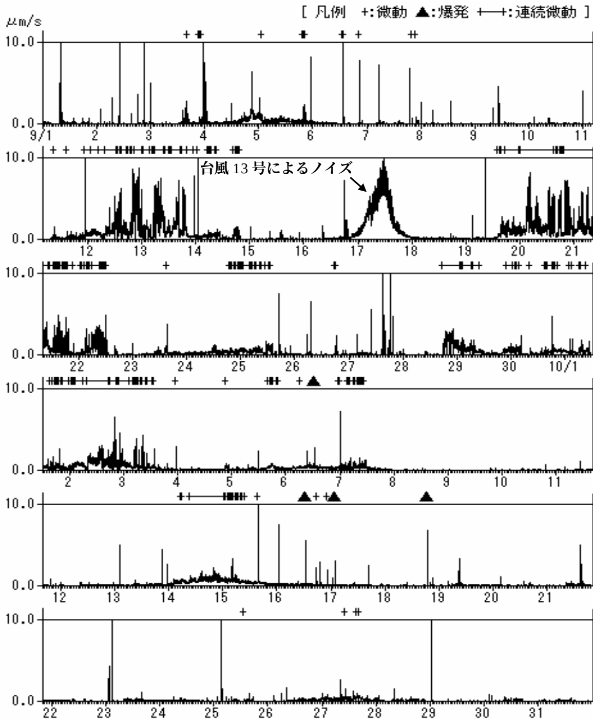
図3 1分間平均振幅の時間変化（SWA1 上下成分） （2006年9月1日～10月31日）
