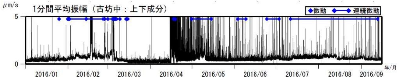
図3 阿蘇山 古坊中観測点上下成分の1分間平均振幅（2016年1月1日～2016年9月15日）
