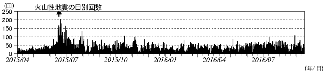
図2 浅間山 火山性地震の日別回数（2015年4月1日～2016年9月15日）（矢印はごく小規模な噴火を示す）
