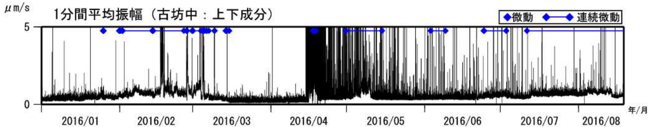
図3 阿蘇山 古坊中観測点上下成分の1分間平均振幅(2016年1月1日～2016年8月18日)
