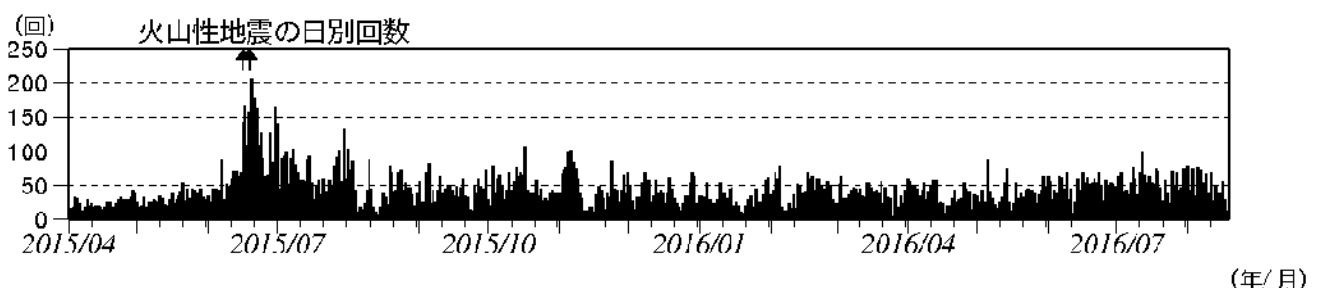
図2 浅間山 火山性地震の日別回数（2015年4月1日～2016年8月18日）（矢印はごく小規模な噴火を示す）
