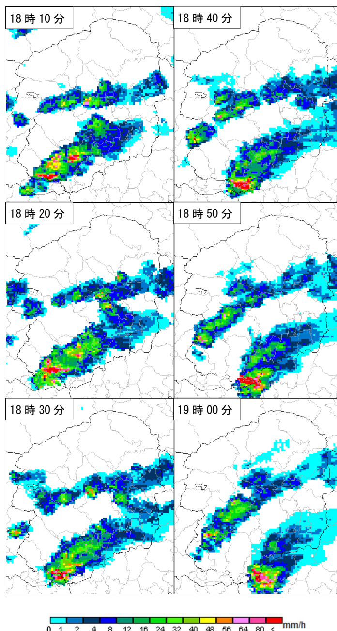
7月10日18時10分から10分毎のレーダー画像
