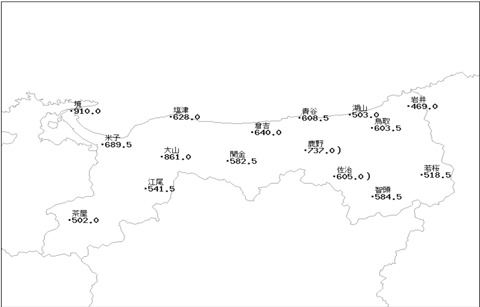
図1 鳥取県内の降水量実況値
