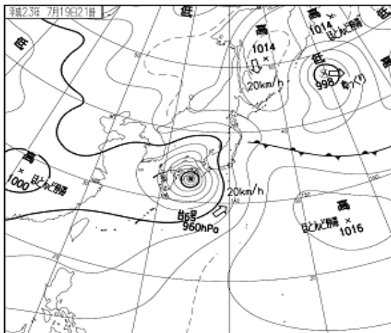
19 日 21 時（日本時間）の地上天気図（左）と気象衛星赤外画像（右）
