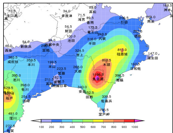
台風第 6 号の台風経路図（左）と 7 月 17 日 18 時～20 日 18 時のアメダス降水量積算図（右）
