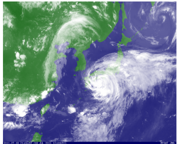
19 日 21 時（日本時間）の地上天気図（左）と気象衛星赤外画像（右）
