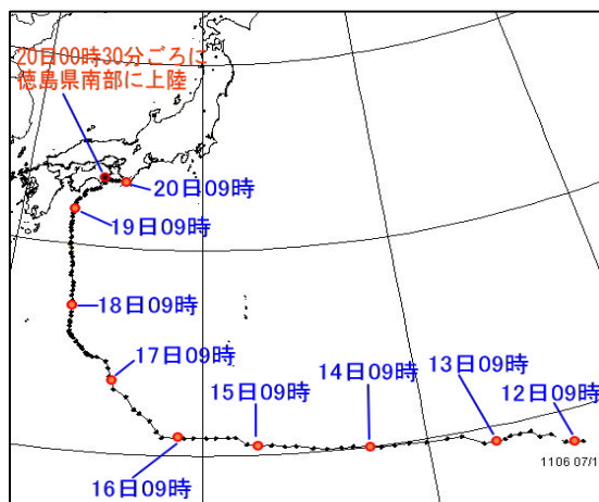
台風第 6 号の台風経路図（左）と 7 月 17 日 18 時～20 日 18 時のアメダス降水量積算図（右）
