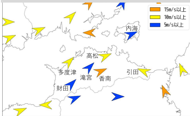
風の状況(日最大風速)(期間:8月9日)
