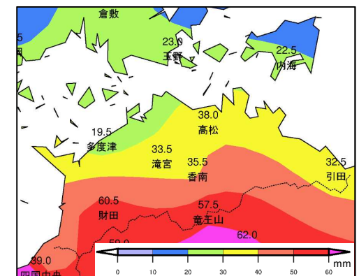
雨量分布図 (期間:8月8日14時~8月9日19時)
