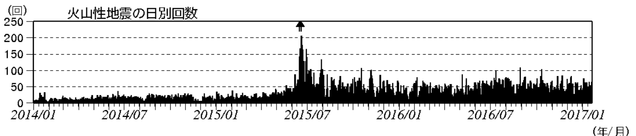
図2 浅間山 火山性地震の日別回数（2014年1月1日～2017年1月19日） （矢印はごく小規模な噴火を示す）
