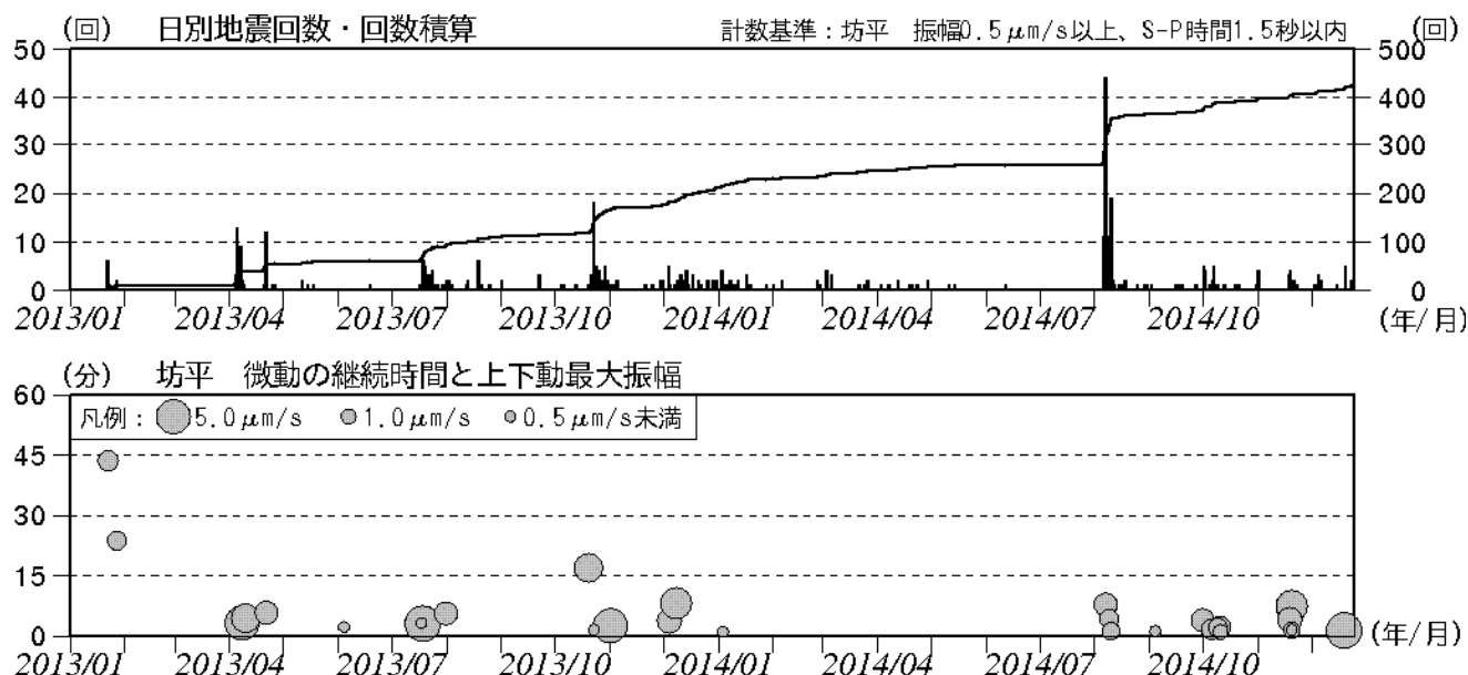
図6 蔵王山 火山性地震の日別回数、火山性微動の発生状況（2013年1月～2014年12月25日24時）
