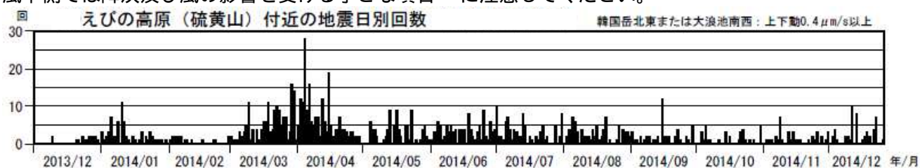
図5 霧島山（えびの高原（硫黄山）周辺） 火山性地震の日別回数 （2013年12月1日～2014年12月25日）
