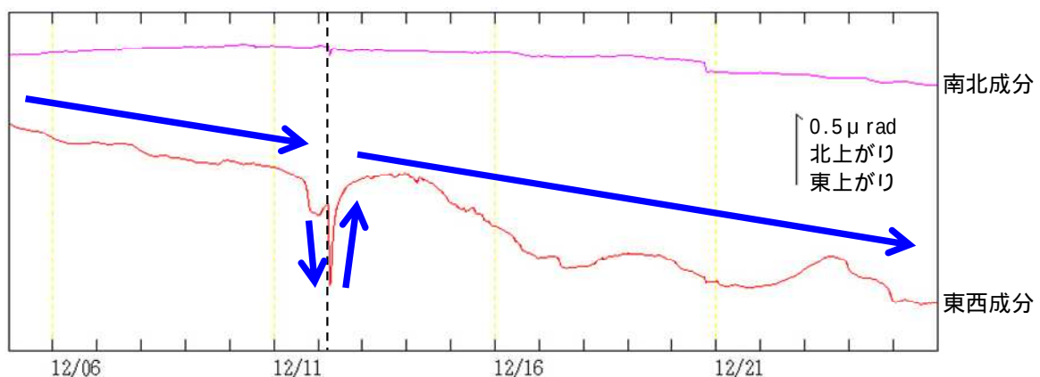
図3 吾妻山 浄土平観測点の傾斜変動（2014年12月5日00時～12月25日15時）
