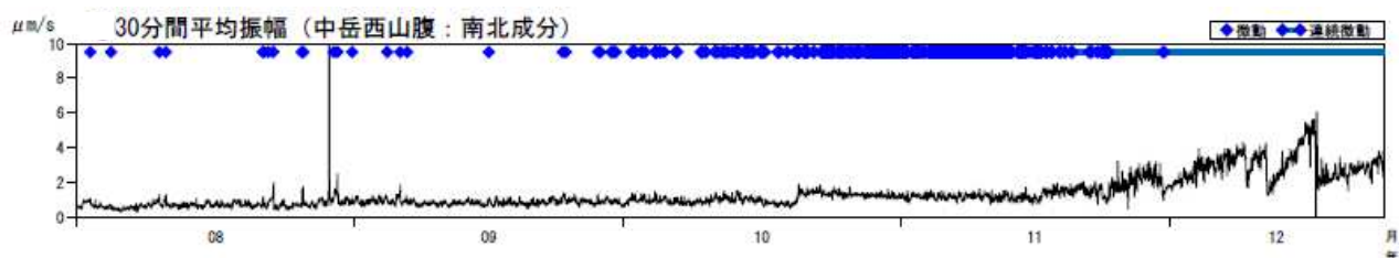
図4 阿蘇山 火山性微動の30分間平均振幅（2014年8月1日～2014年12月25日）
