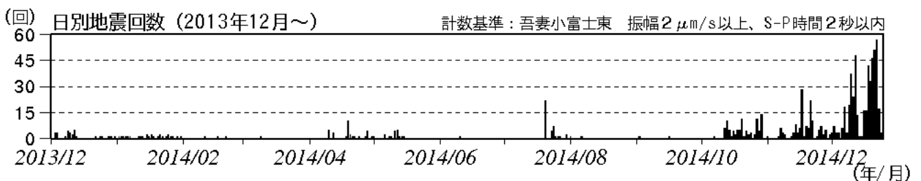
図2 吾妻山 火山性地震の日別回数（2013年12月1日～12月25日）
