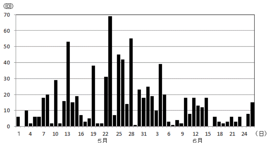
図2 草津白根山 日別地震回数（5月1日～6月26日）
