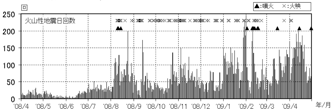
図2 浅間山 火山性地震の日別回数（2008年4月1日～2009年4月30日）
