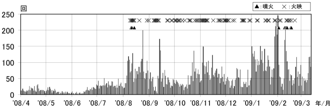
図2 浅間山 火山性地震の日別回数（2008年4月1日～2009年3月12日）
