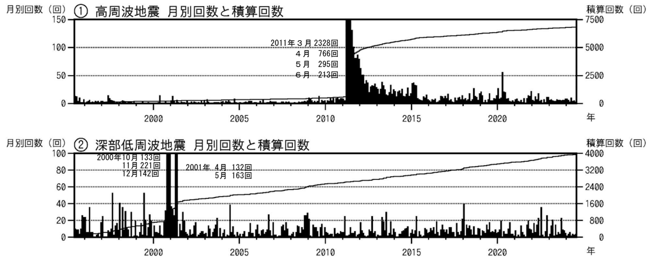
図2 富士山 月別地震回数（1995年6月1日～2024年7月31日）
