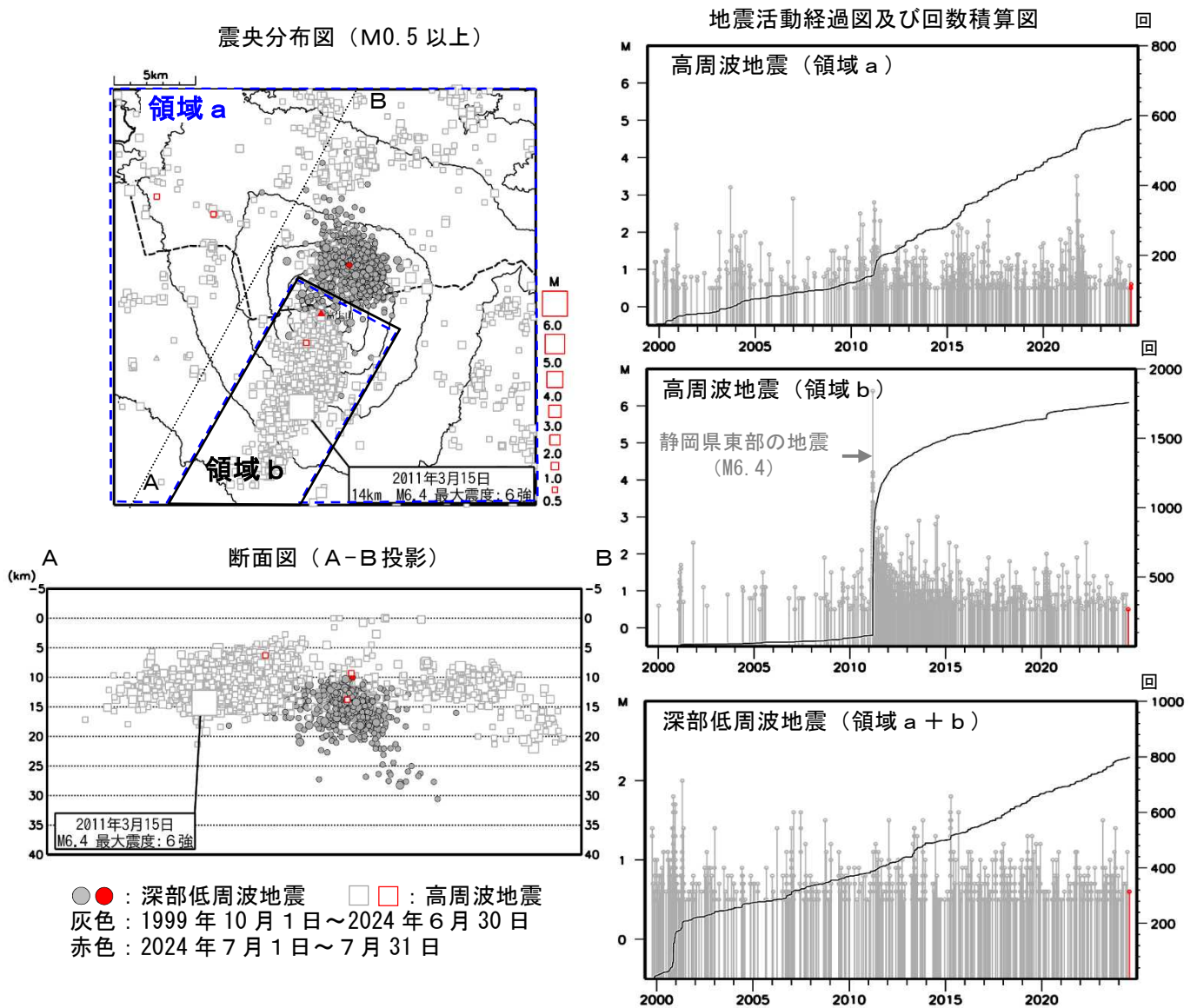
図3 富士山 広域地震観測網による山体及び周辺の地震活動(1999年10月1日～2024年7月31日)
