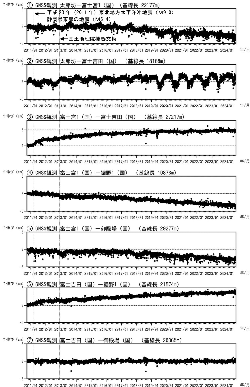
図4 富士山 GNSS 連続観測による基線長変化 (2010 年 10 月 1 日～2024 年 7 月 31 日) (国): 国土地理院 「平成 23 年 (2011 年) 東北地方太平洋沖地震」及び 2011 年 3 月 15 日に発生した静岡県東部の地震 (M 6.4) によるステップ状の変化を補正しています。 ①～⑦は図5の GNSS 基線①～⑦に対応しています。
