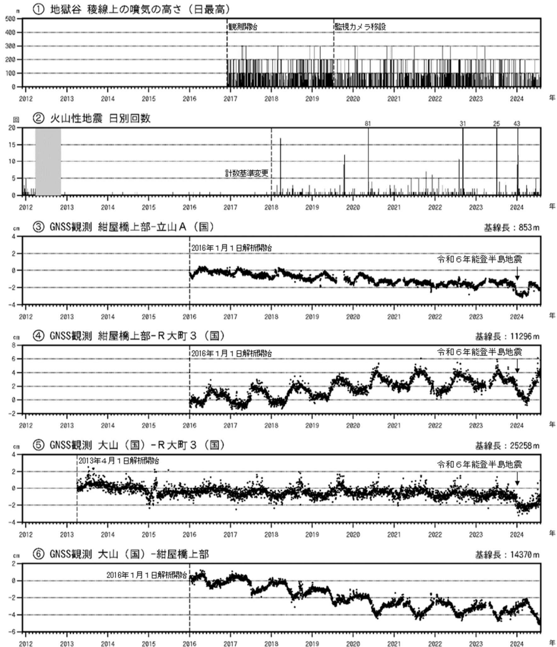
図3 弥陀ヶ原 火山活動経過図（2011年12月1日～2024年7月31日）
