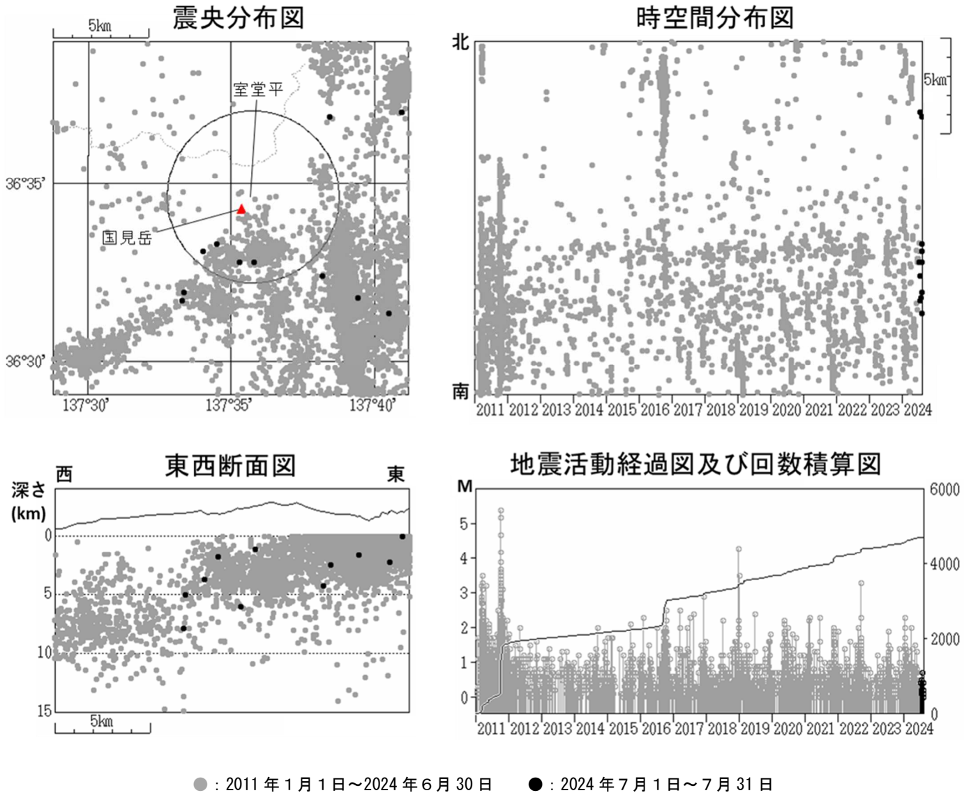
図2 弥陀ヶ原 広域地震観測網による山体・周辺の地震活動（2011 年 1 月 1 日～2024 年 7 月 31 日） 震央分布図中の円は弥陀ヶ原の計数対象地震（室堂平で S-P 時間 1 秒以内）のおよその範囲を示しています。 広域地震観測網により震源決定したもので、深さは全て海面以下として決定しています。 図中の震源要素は一部暫定値が含まれており、後日変更することがあります。 この図では、関係機関の地震波形を一元的に処理し、地震観測点の標高を考慮する等した手法で得られた震源を用いています（ただし、2020 年 8 月以前の地震については火山活動評価のための参考震源です）。
