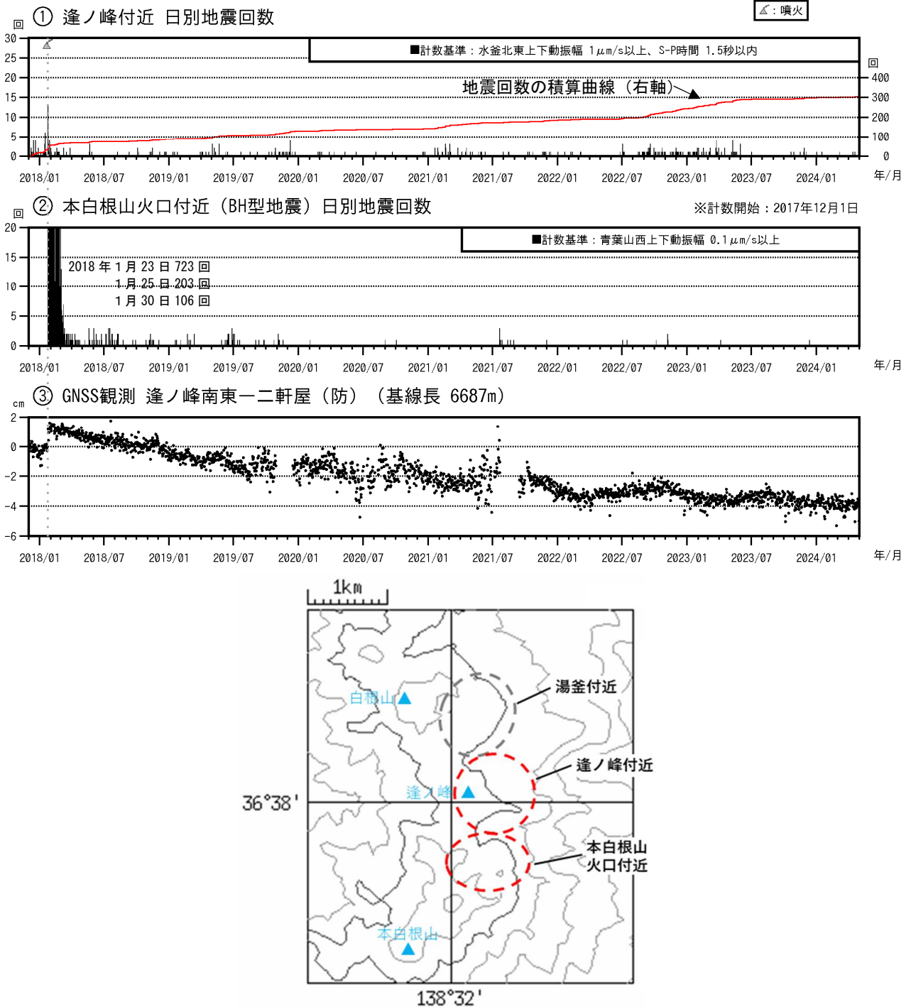
図13 草津白根山（本白根山） 火山活動経過図（2017年12月1日～2024年4月30日）
