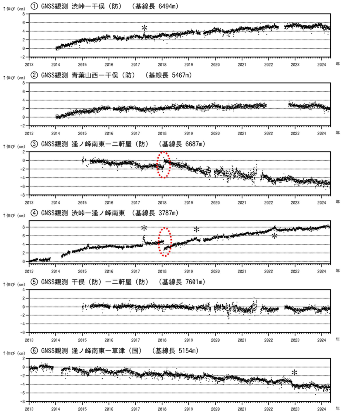
図6 草津白根山 GNSS 連続観測の結果（2013年1月1日～2024年4月30日）
