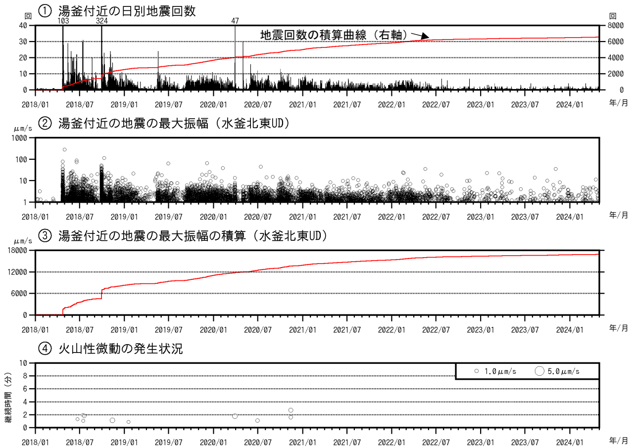
図1 草津白根山（白根山（湯釜付近）） 湯釜付近の地震活動及び火山性微動の発生状況 （2018年1月1日～2024年4月30日）
