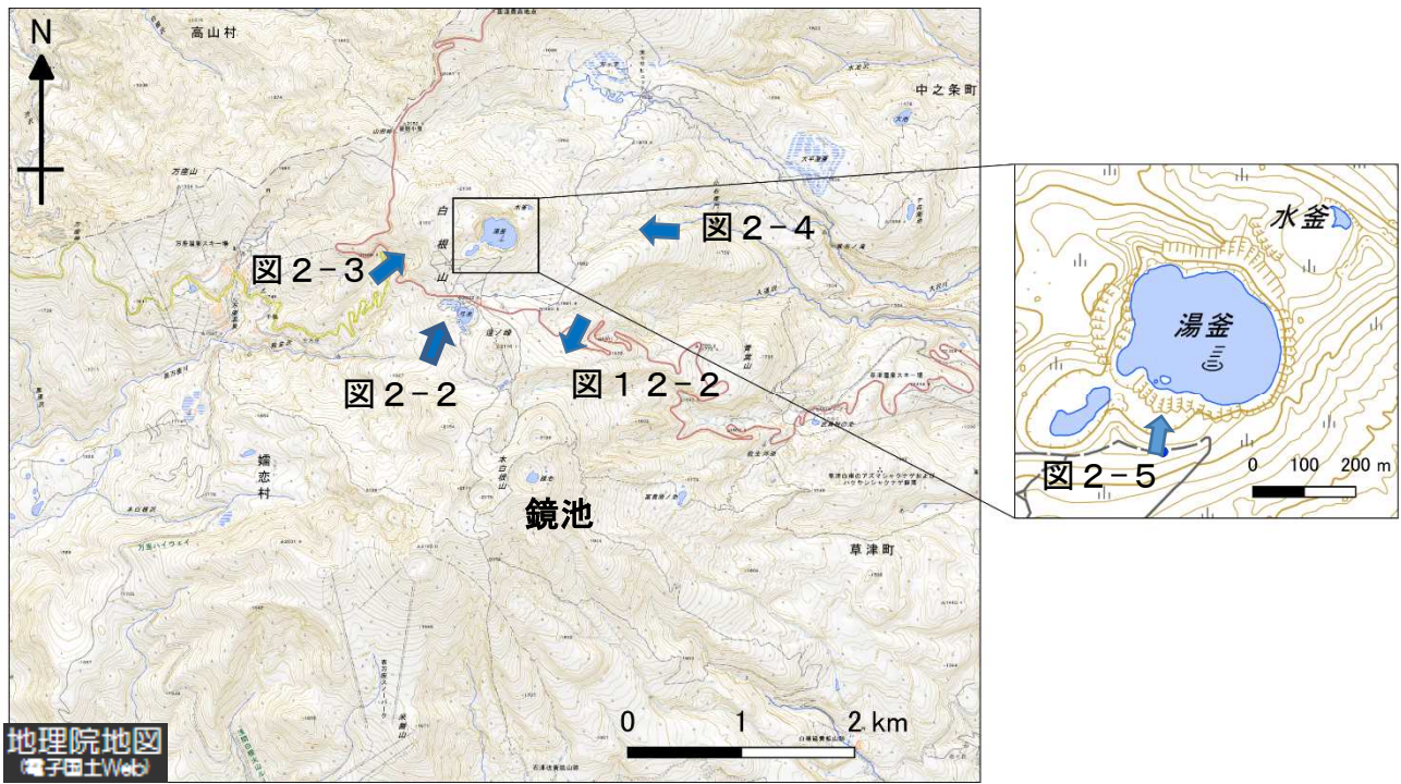
図 2-6 草津白根山 写真撮影位置及び撮影方向 ・ 矢印は図 2-2～2-5 及び図 12-2 の撮影位置及び撮影方向を示します。
