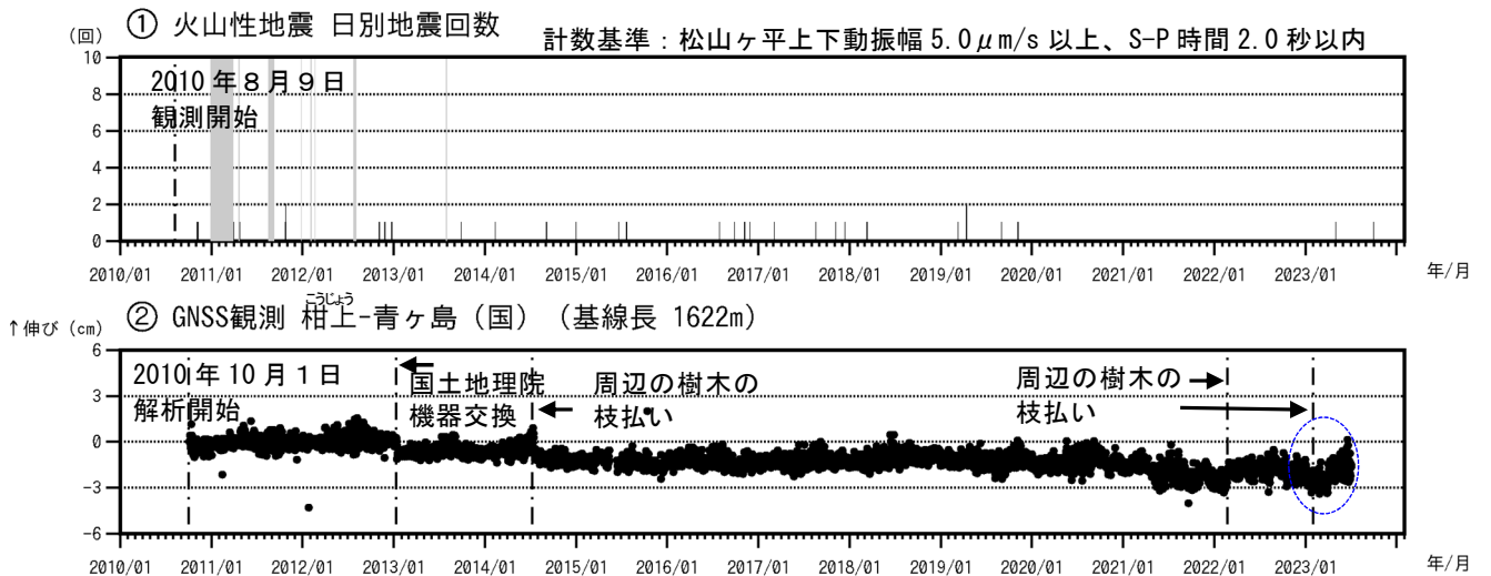
図3 青ヶ島 火山活動経過図（2010年8月9日～2024年1月31日） ① グラフの灰色部分は機器障害による欠測を示す。 ② (国)：国土地理院、図4のGNSS基線②に対応。グラフの空白部分は柑上の障害による欠測を示す。 ・青破線で囲んだ変化は原因不明の変化ですが、火山活動によるものではないと考えています。
