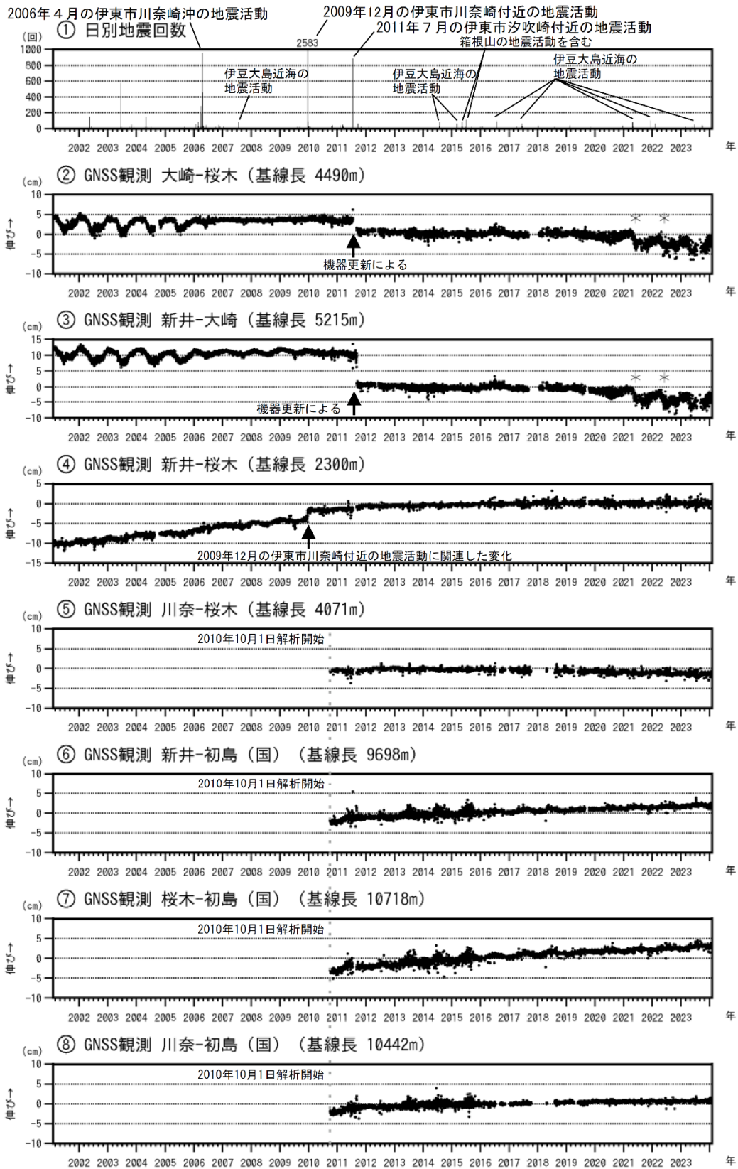
図3 伊豆東部火山群 火山活動経過図（2001年2月1日～2024年1月31日）
