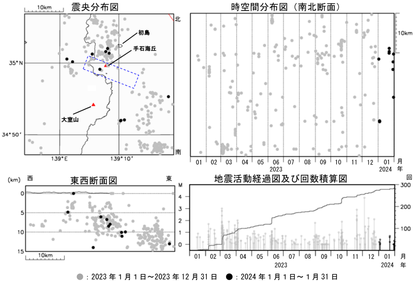
図2 伊豆東部火山群 広域地震観測網による震源分布図（2023年1月1日～2024年1月31日） □の領域は群発地震活動の発生する可能性がある範囲（火口が出現する可能性がある範囲）を示しています。 ( https://www.data.jma.go.jp/vois/data/tokyo/STOCK/level/PDF/level_316.pdf ) 広域地震観測網により震源決定したもので、深さは全て海面以下として決定しています。 M（マグニチュード）は地震の規模を表し、M0.0以上を表示しています。 図中の震源要素は一部暫定値が含まれており、後日変更することがあります。 この図では、関係機関の地震波形を一元的に処理し、地震観測点の標高を考慮する等した手法で得られた震源を用いています。
