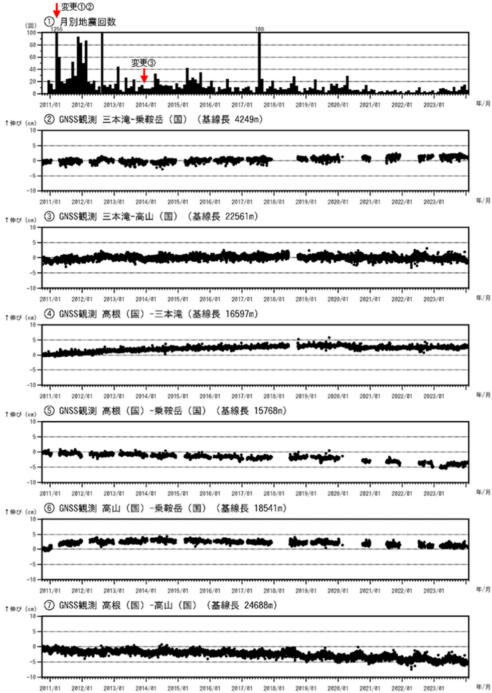
図2 乗鞍岳 火山活動経過図（2010年10月1日～2024年1月31日）
