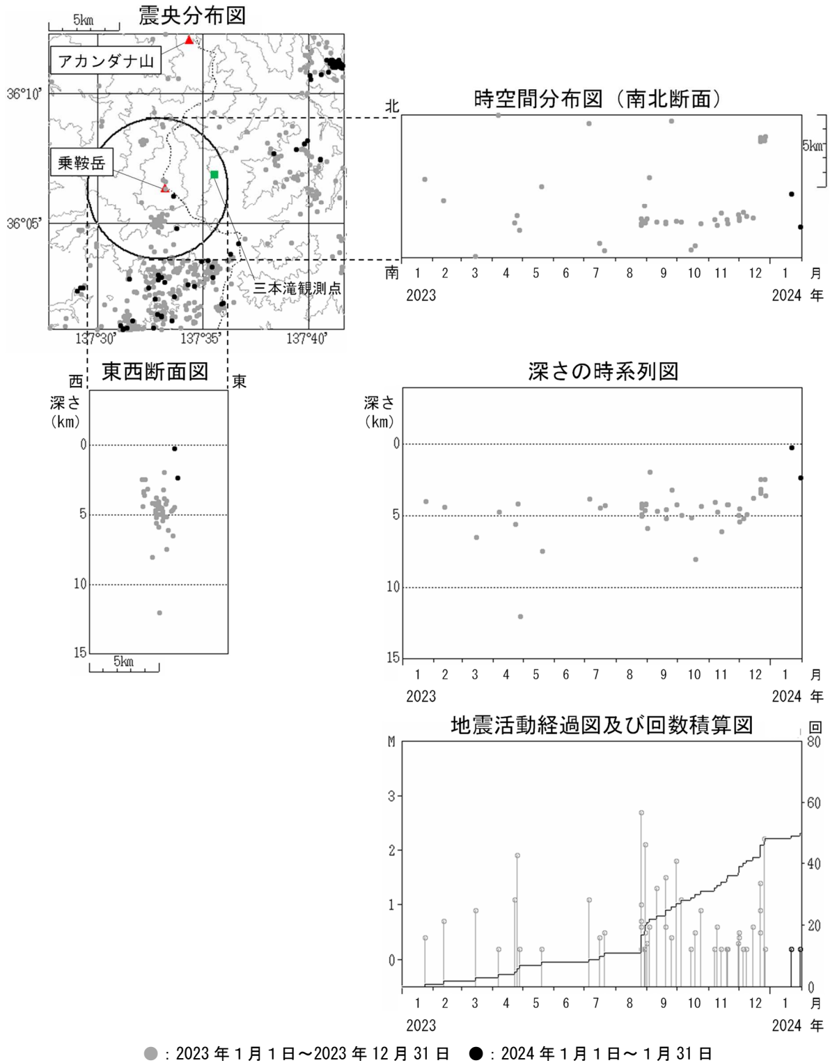
図3 乗鞍岳 広域地震観測網による山体・周辺の地震活動(2023年1月1日～2024年1月31日) M(マグニチュード)は地震の規模を表し、M0.2以上の地震を表示しています。 広域地震観測網により震源決定したもので、深さは全て海面以下として決定しています。図中の震源要素は一部暫定値が含まれており、後日変更することがあります。 この図では、関係機関の地震波形を一元的に処理し、地震観測点の標高を考慮する等した手法で得られた震源を用いています。 東西断面図、時空間分布図及び深さの時系列図には、乗鞍岳付近(震央分布図中の黒線円の範囲)の地震を示しています。 ・乗鞍岳付近の地震活動は、低調に経過しています。
