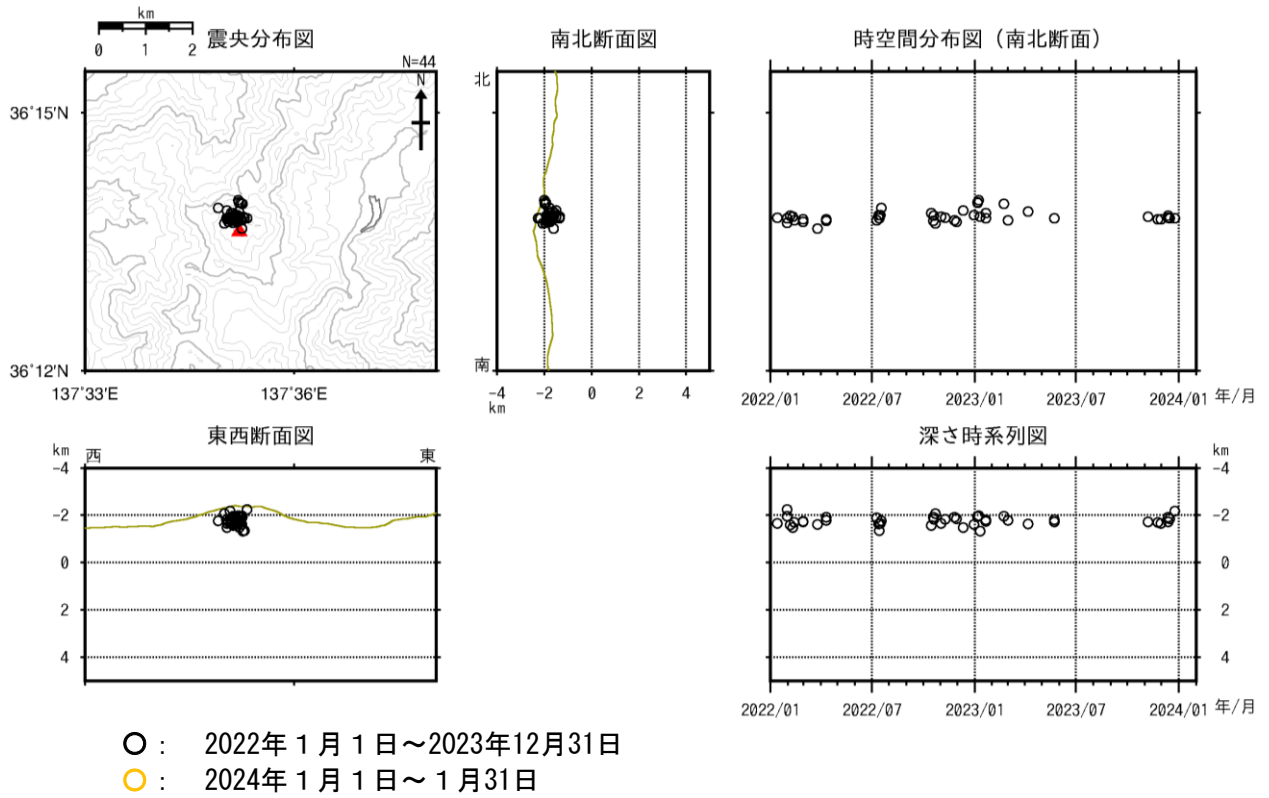
図2 焼岳 山頂付近の地震の震源分布図（2022年1月1日～2024年1月31日）
