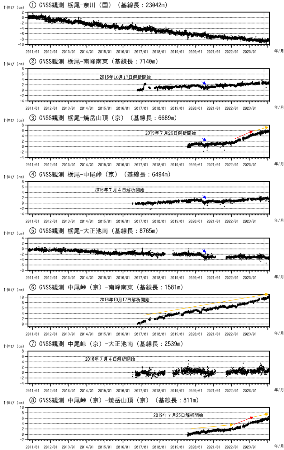
図6 焼岳 GNSS 連続観測による基線長変化（2010年10月1日～2024年1月31日）
