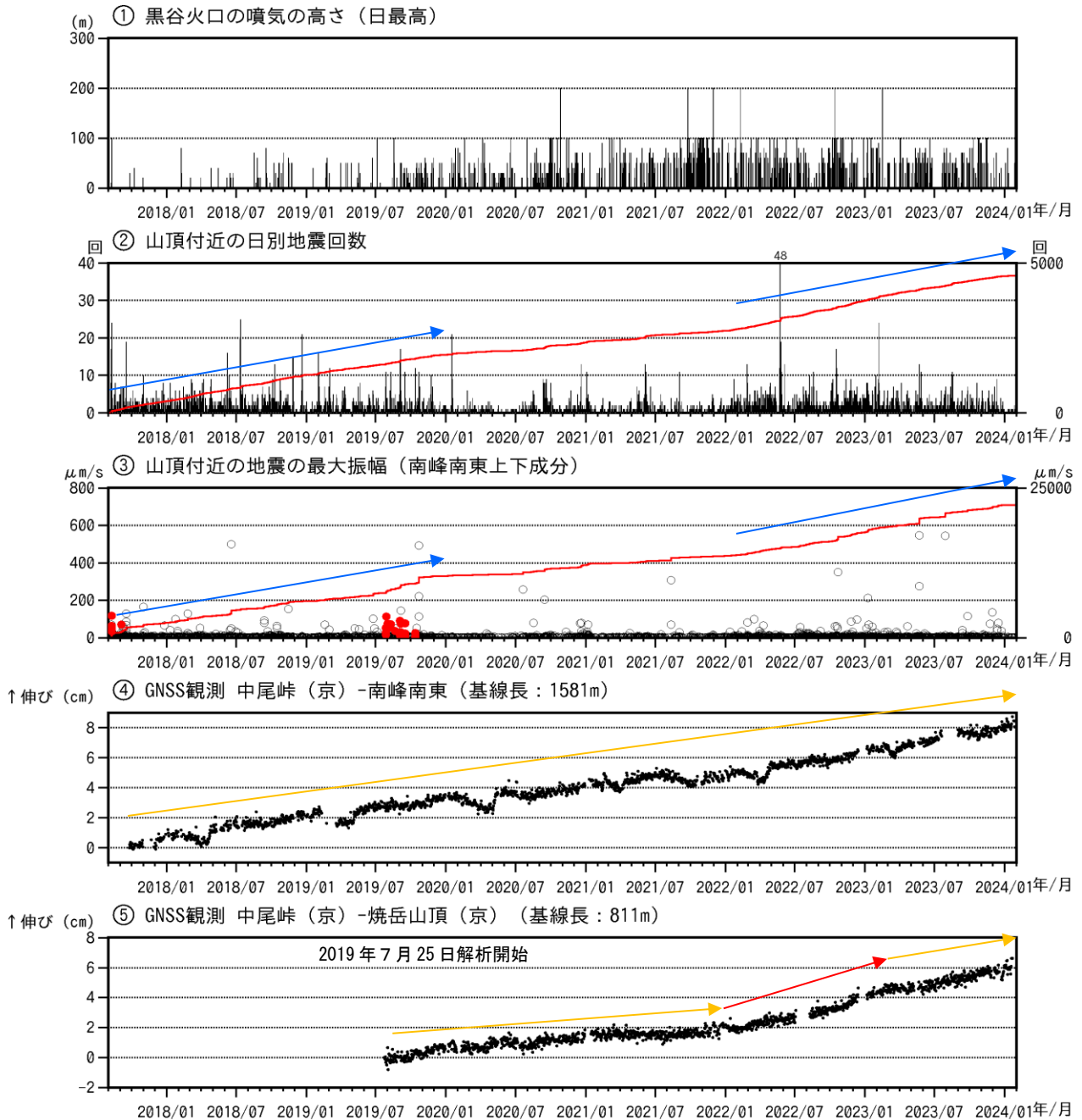
図1 焼岳 火山活動経過図（2017年8月1日～2024年1月31日）
