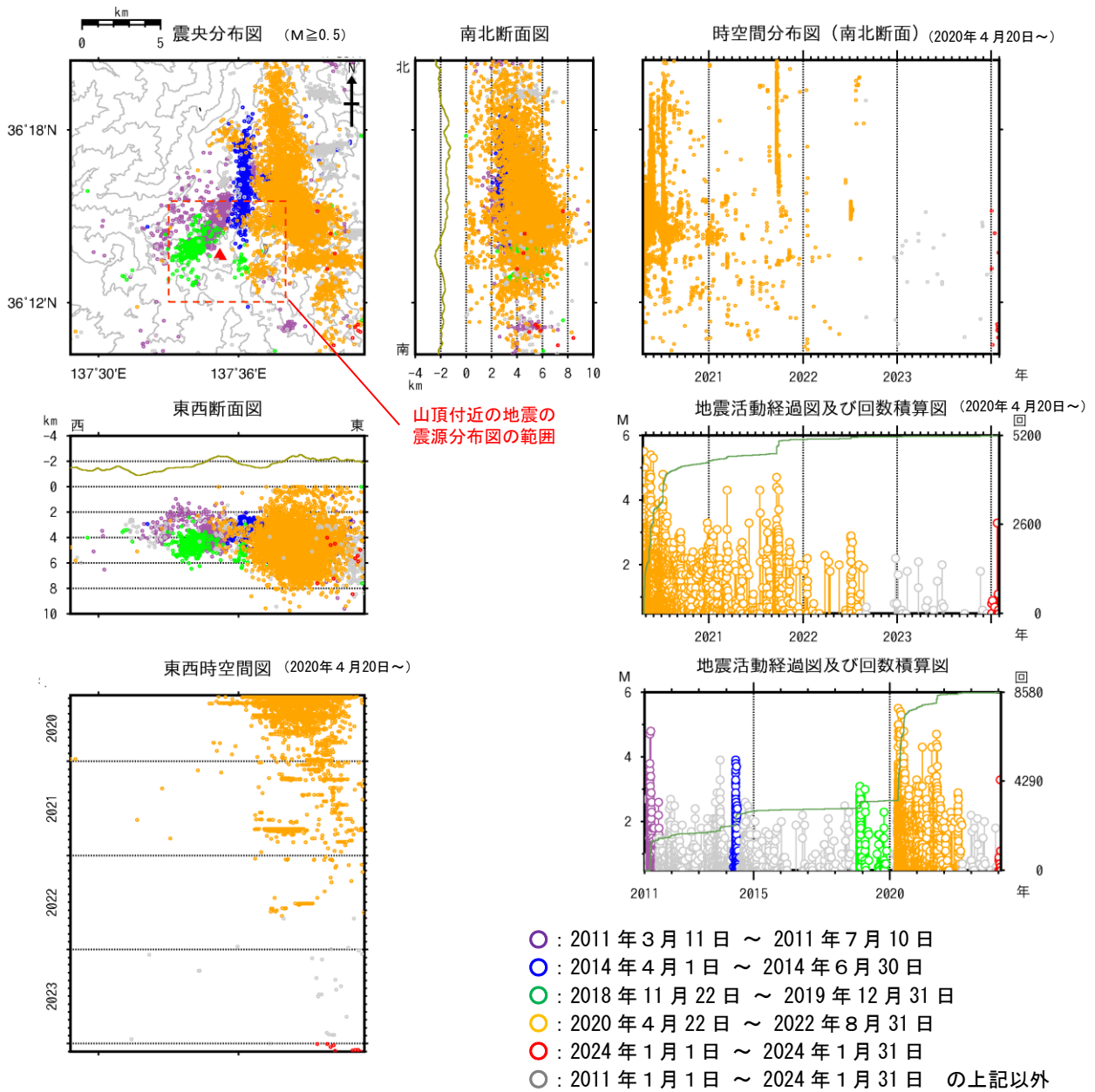
図9 焼岳 広域地震観測網による山体及び周辺の地震活動(2011年1月1日~2024年1月31日)
