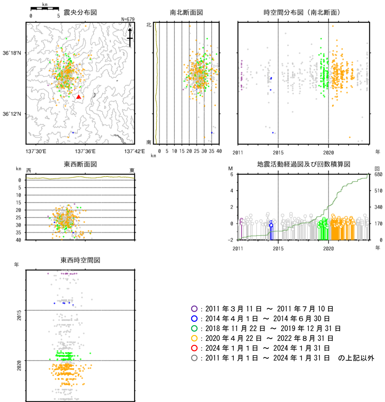
図10 焼岳 広域地震観測網による深部低周波地震の震源分布図（2011年1月1日～2024年1月31日） 広域地震観測網により震源決定したもので、深さは全て海面以下として決定しています。そのため、山頂付近の浅い地震の震源も海面下に決定されています。 M（マグニチュード）は地震の規模を表します。 図中の震源要素は一部暫定値が含まれており、後日変更することがあります。 ・焼岳の北西側の深い所を震源とする低周波地震の発生状況に特段の変化はみられません。 ・過去には、図9に示したような焼岳周辺の地震活動の活発化がみられた期間付近で、深部低周波地震が増加したことがあります。
