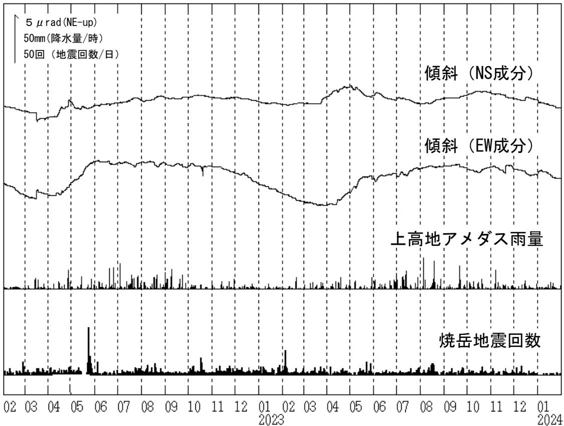
図8 焼岳 南峰南東観測点における傾斜データ（2022年1月1日～2024年1月31日）
