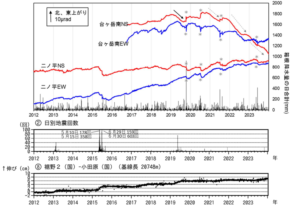
図5 箱根山 傾斜観測及び地震回数・GNSS観測（2012年1月1日～2023年12月31日） *印は降水による影響と考えられる変動を示します。(国)：国土地理院 ⑧は図3-2 基線⑧に対応します。
