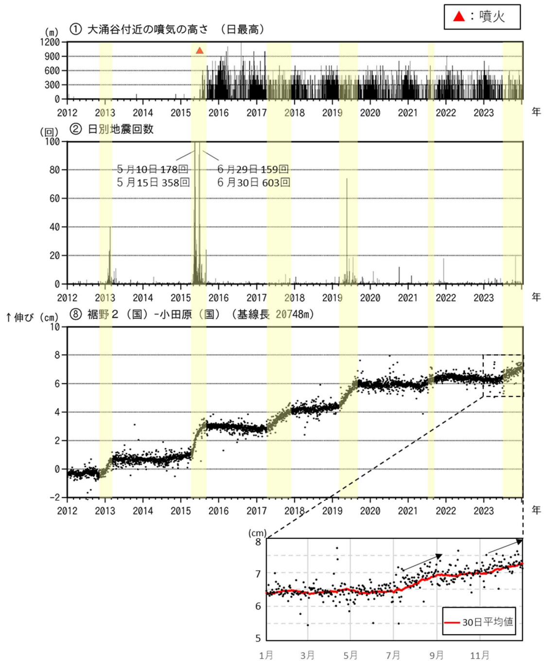
図3-1 箱根山 火山活動経過図（2012年1月1日～2023年12月31日）
