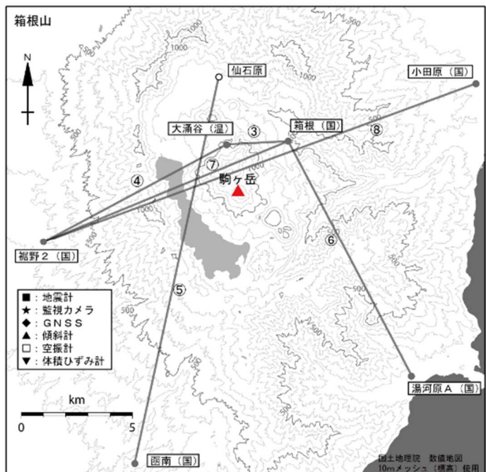
図3-2 箱根山 GNSS 連続観測による基線長変化及び観測点配置図 (2012年1月1日~2023年12月31日) (国): 国土地理院 (温): 神奈川県温泉地学研究所 空白部分は欠測を示します。
