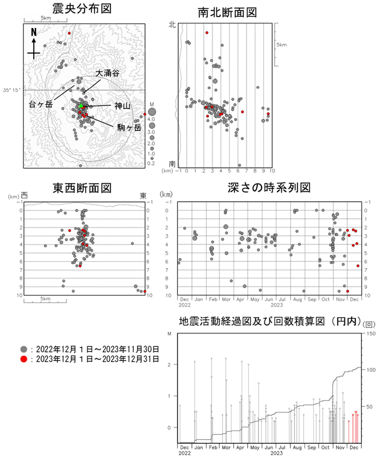
図4 箱根山 広域地震観測網による山体周辺の震源分布図（2022年12月1日～2023年12月31日）
