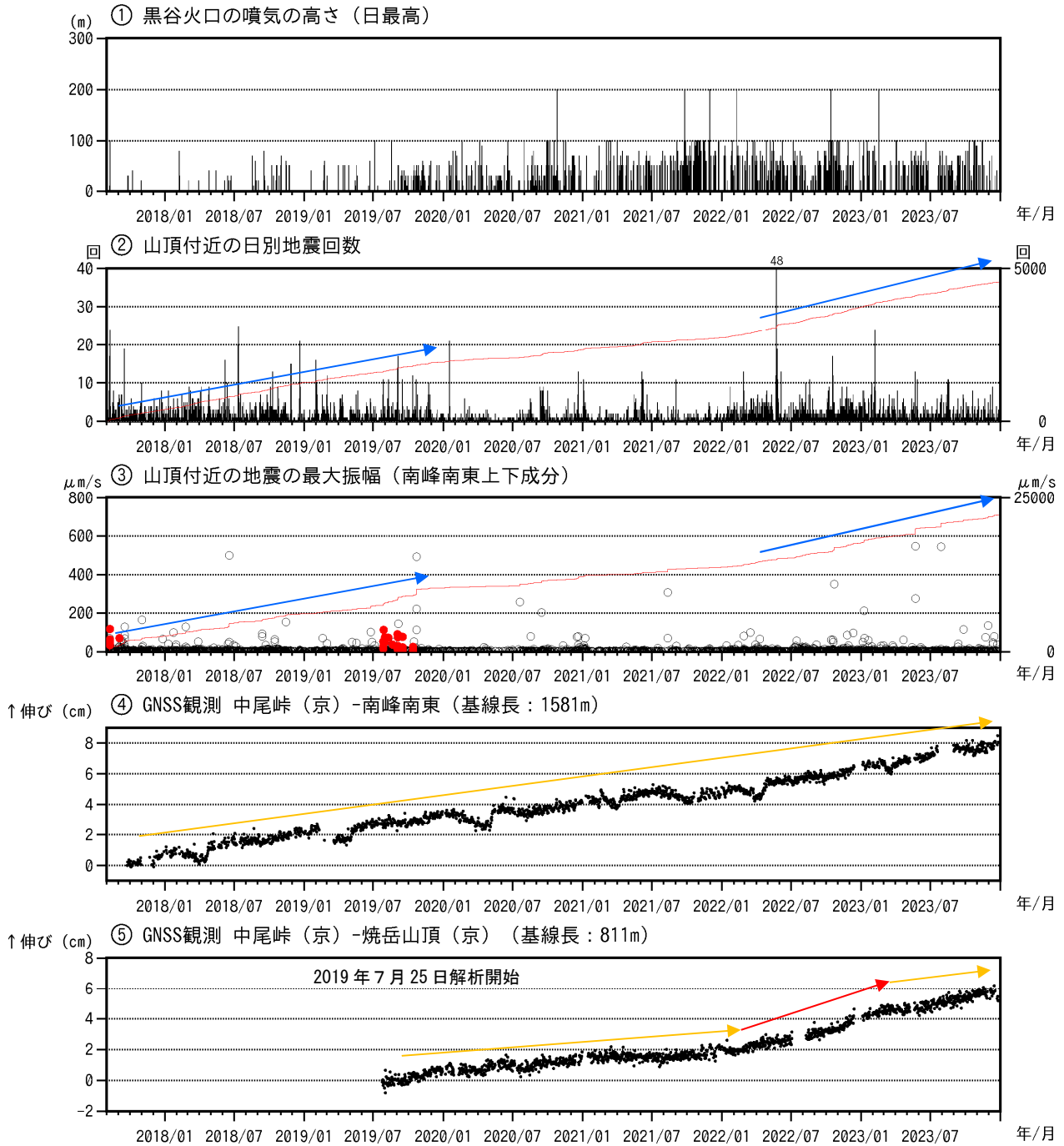
図1 焼岳 火山活動経過図（2017年8月1日～2023年12月31日）
