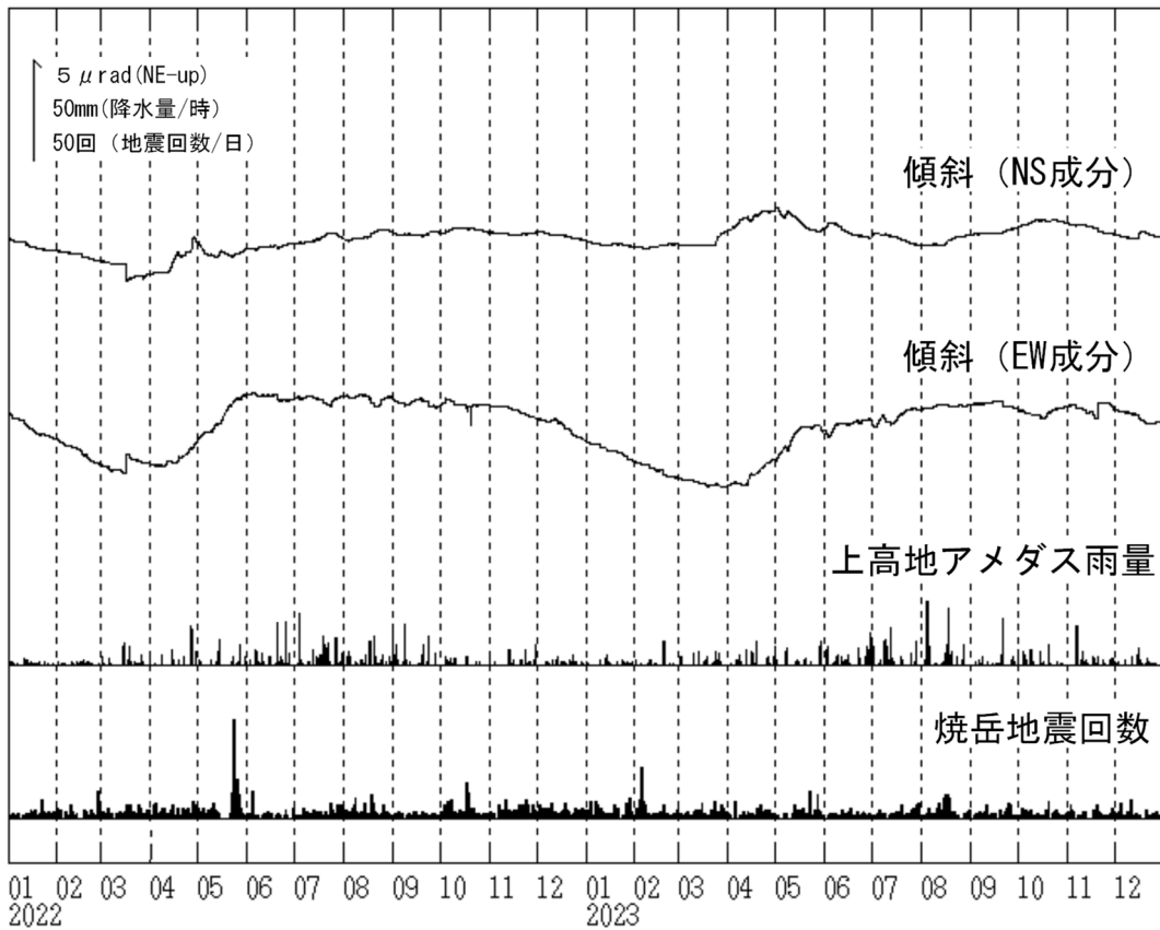
図8 焼岳 南峰南東観測点における傾斜データ (2022年1月1日～2023年12月31日)
