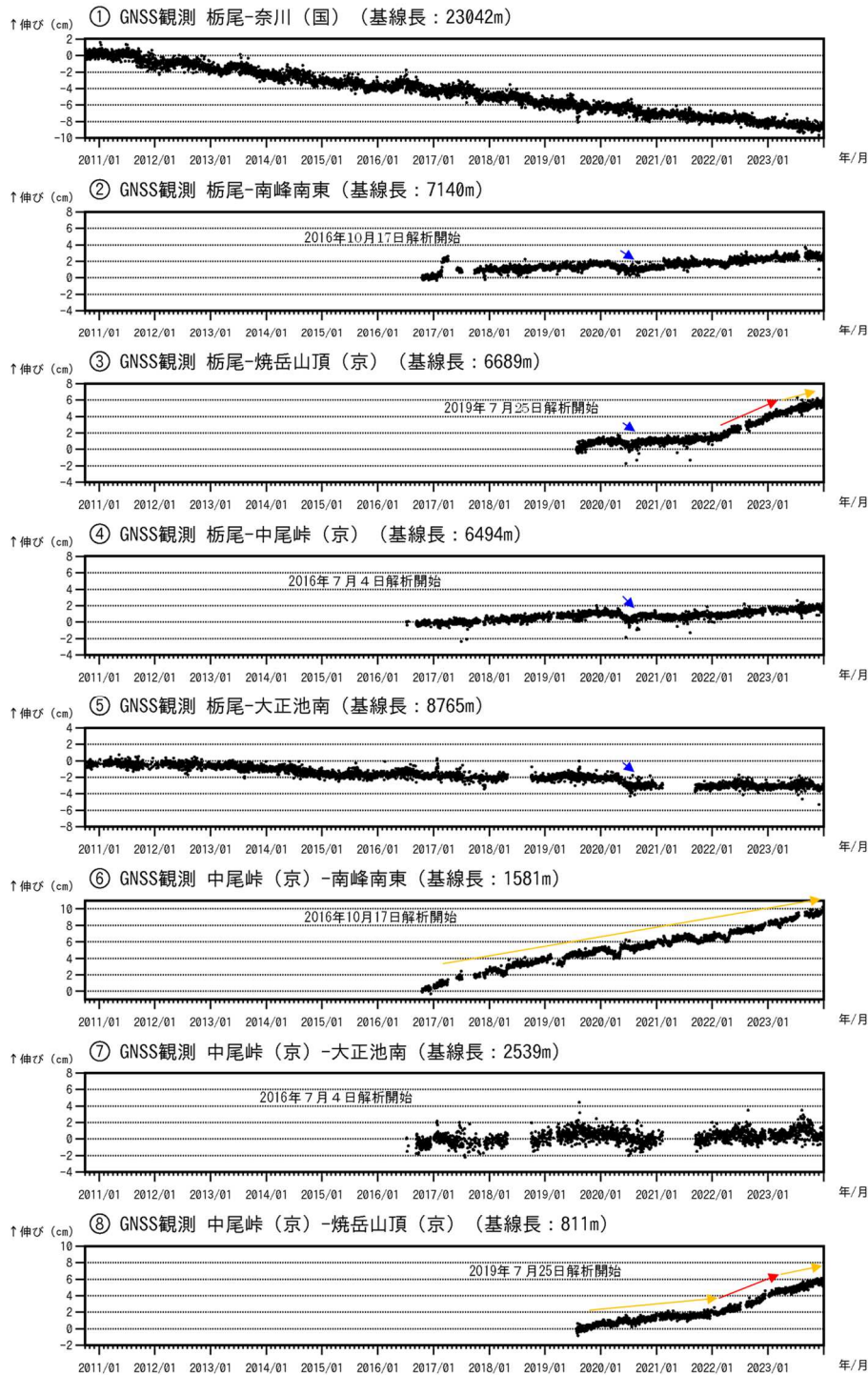
図6 焼岳 GNSS 連続観測による基線長変化 (2010 年 10 月 1 日～2023 年 12 月 31 日)
