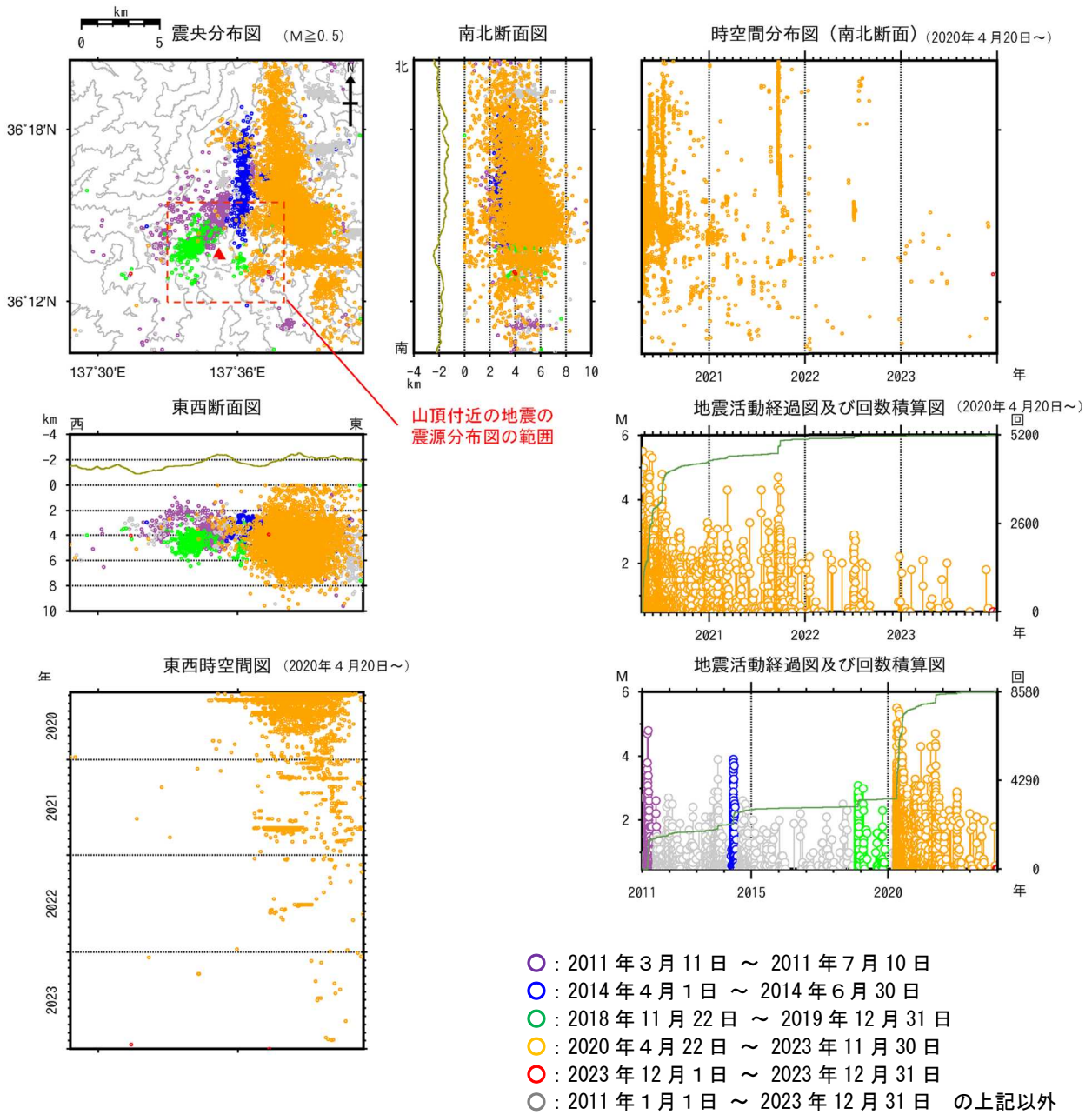
図9 焼岳 広域地震観測網による山体及び周辺の地震活動(2011年1月1日～2023年12月31日)
