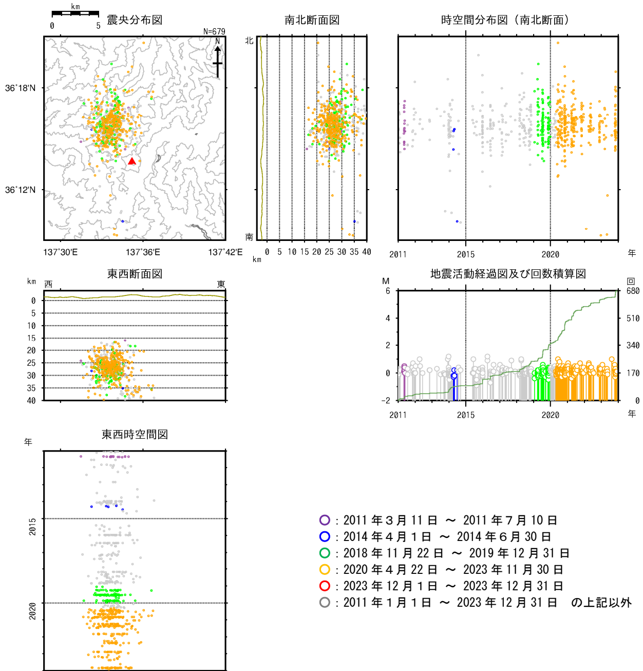
図10 焼岳 広域地震観測網による深部低周波地震の震源分布図（2011年1月1日～2023年12月31日） 広域地震観測網により震源決定したもので、深さは全て海面以下として決定しています。そのため、山頂付近の浅い地震の震源も海面下に決定されています。 M（マグニチュード）は地震の規模を表します。 図中の震源要素は一部暫定値が含まれており、後日変更することがあります。 ・ 焼岳の北西側の深い所を震源とする低周波地震の発生状況に特段の変化はみられません。 ・ 過去には、図9に示したような焼岳周辺の地震活動の活発化がみられた期間付近で、深部低周波地震が増加したことがあります。
