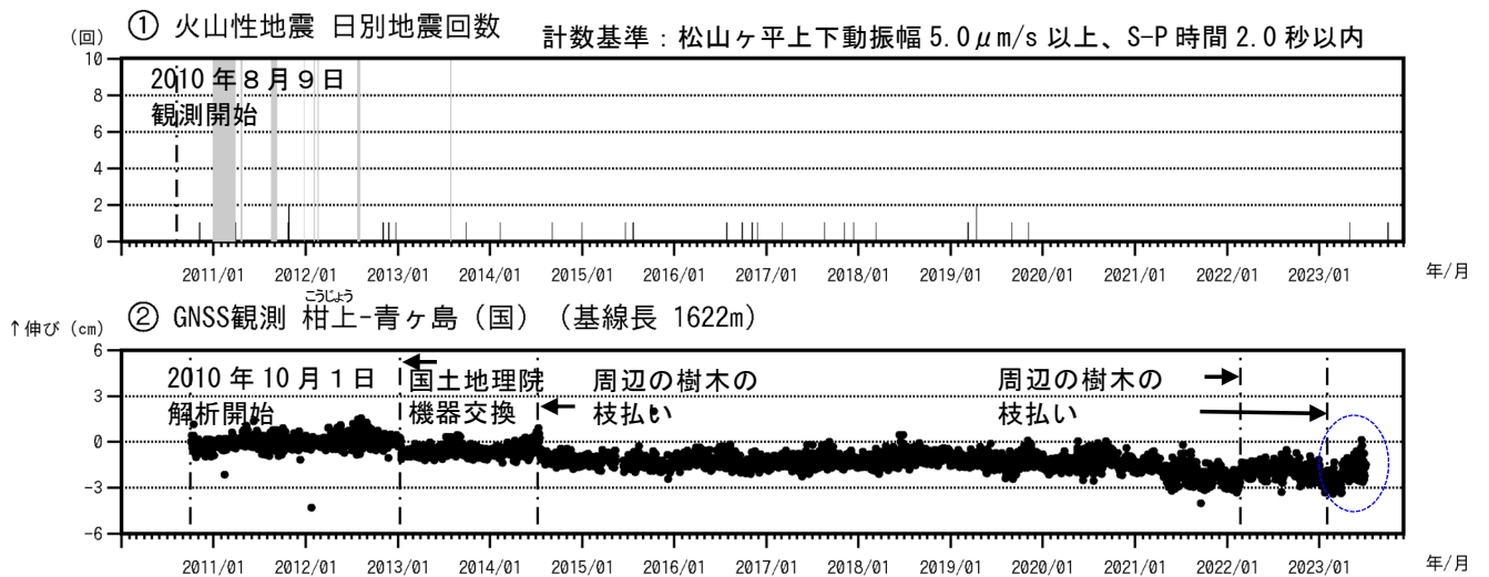
図3 青ヶ島 火山活動経過図（2010年8月9日～2023年11月30日）
