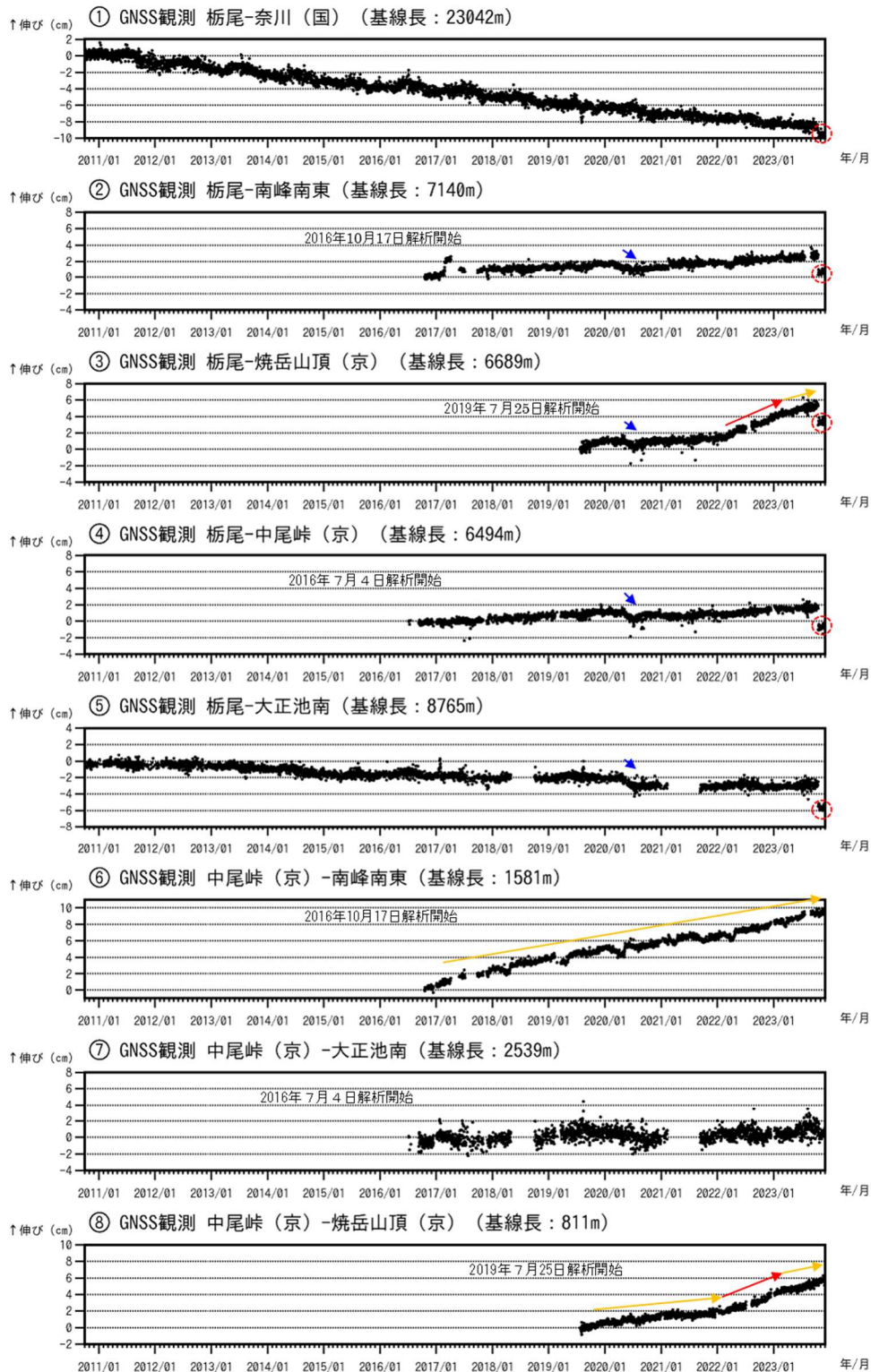
図6 焼岳 GNSS 連続観測による基線長変化 (2010年10月1日~2023年11月30日)
