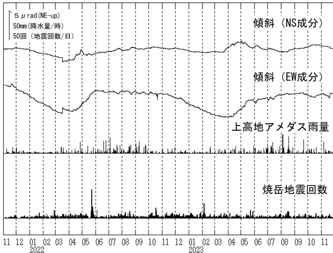
図8 焼岳 南峰南東観測点における傾斜データ (2021年11月1日～2023年11月30日)
