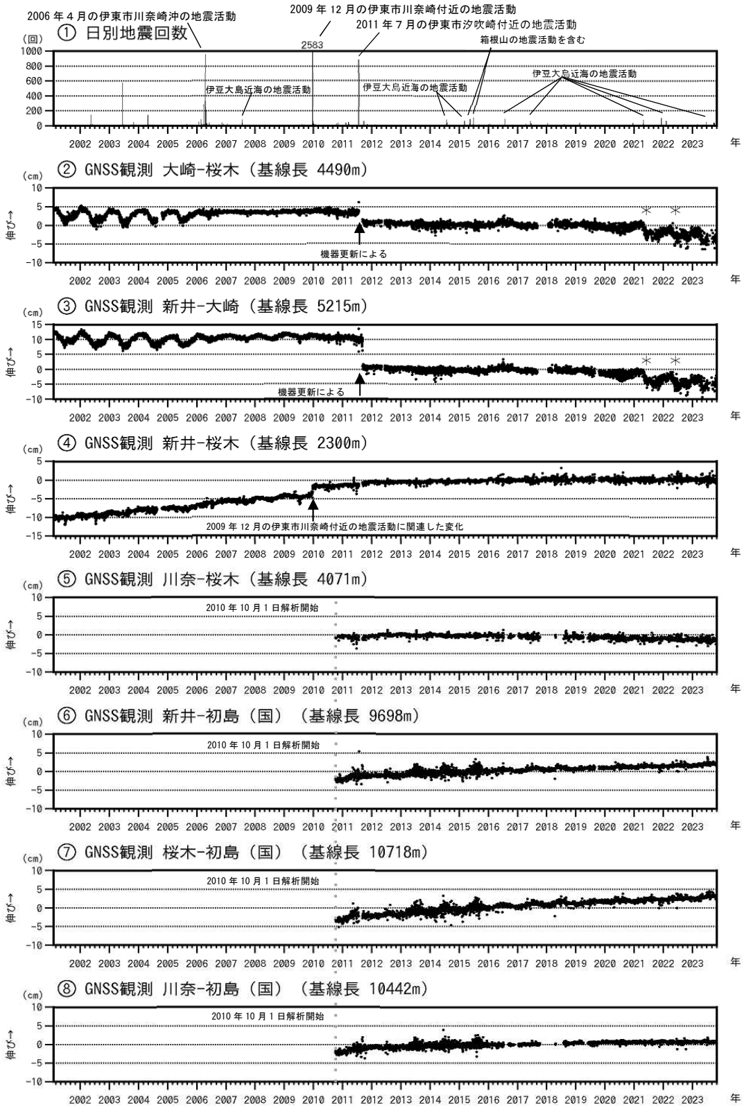
図3 伊豆東部火山群 火山活動経過図 (2001年2月1日~2023年10月31日)
