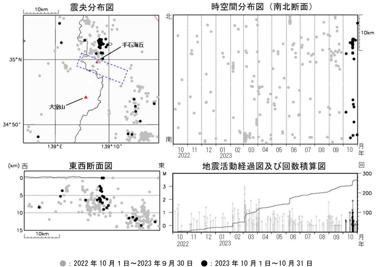
図2 伊豆東部火山群 広域地震観測網による震源分布図（2022年10月1日～2023年10月31日） □の領域は群発地震活動の発生する可能性がある範囲（火口が出現する可能性のある範囲）を示しています。 https://www.data.jma.go.jp/vois/data/tokyo/STOCK/level/PDF/level_316.pdf 広域地震観測網により震源決定したもので、深さは全て海面以下として決定しています。 M（マグニチュード）は地震の規模を表し、M0.0以上を表示しています。 図中の震源要素は一部暫定値が含まれており、後日変更することがあります。 この図では、関係機関の地震波形を一元的に処理し、地震観測点の標高を考慮する等した手法で得られた震源を用いています。
