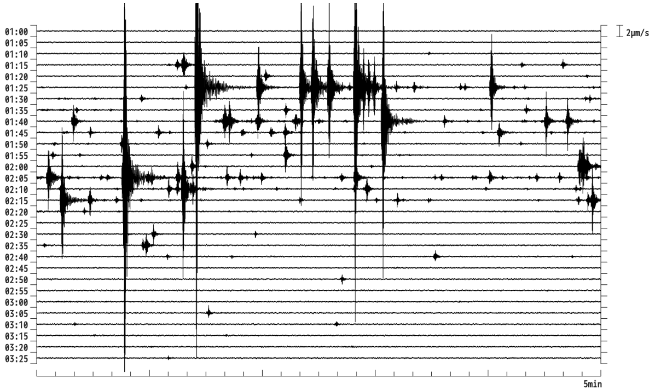
図5 箱根山 10月31日01時00分～03時30分の地震波形図（駒ヶ岳（温） 短周期 上下成分）
