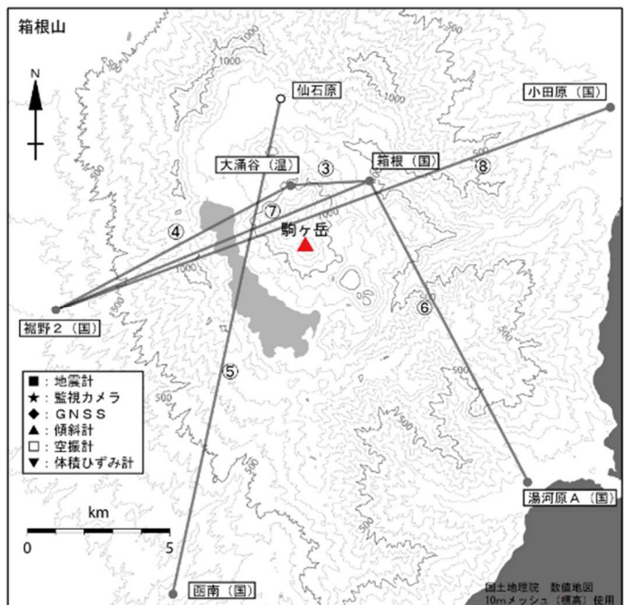
図3-2 箱根山 GNSS 連続観測による基線長変化及び観測点配置図 (2012年1月1日～2023年10月31日) (国)：国土地理院 (温)：神奈川県温泉地学研究所 空白部分は欠測を示します。
