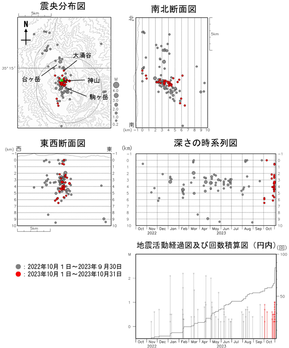
図4 箱根山 広域地震観測網による山体周辺の震源分布図（2022年10月1日～2023年10月31日）
