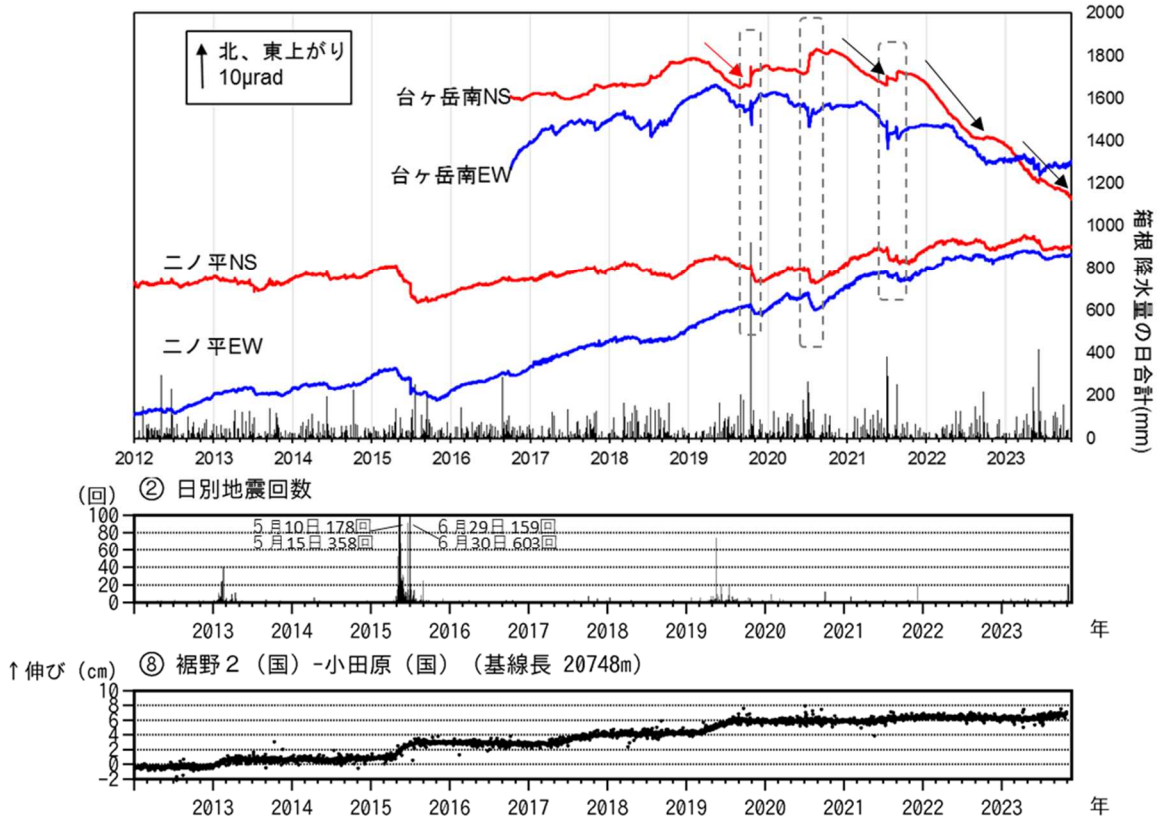
図6 箱根山 傾斜観測及び地震回数・GNSS観測（2012年1月1日～2023年10月31日）
