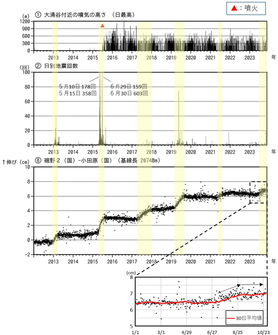
図3-1 箱根山 火山活動経過図（2012年1月1日～2023年10月31日）
