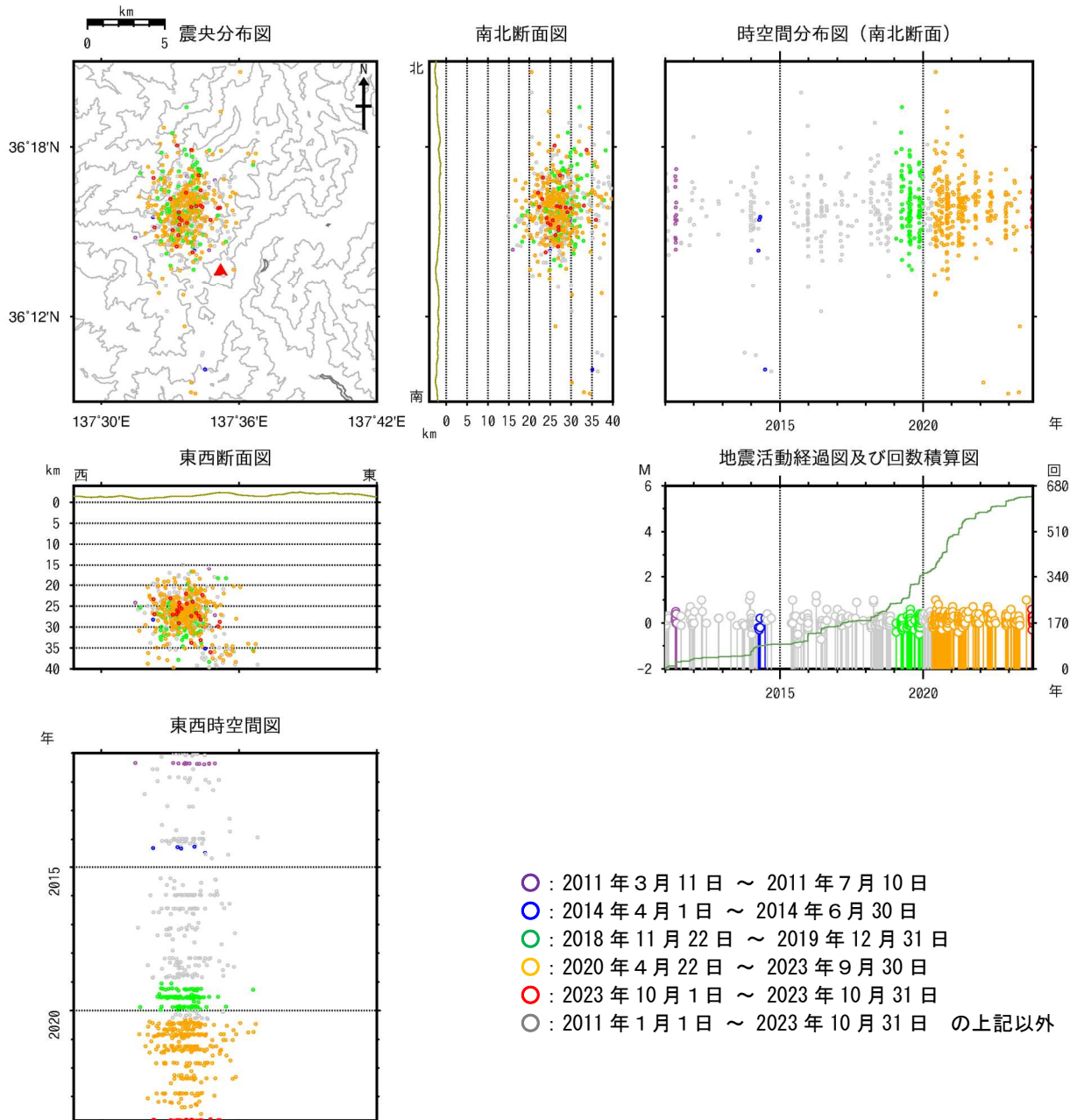
図10 焼岳 広域地震観測網による深部低周波地震の震源分布図（2011年1月1日～2023年10月31日） 広域地震観測網により震源決定したもので、深さは全て海面以下として決定しています。そのため、山頂付近の浅い地震の震源も海面下に決定されています。 M（マグニチュード）は地震の規模を表します。 図中の震源要素は一部暫定値が含まれており、後日変更することがあります。 ・焼岳の北西側の深い所を震源とする低周波地震の発生状況に特段の変化はみられません。 ・過去には、図9に示したような焼岳周辺の地震活動の活発化がみられた期間付近で、深部低周波地震が増加したことがあります。
