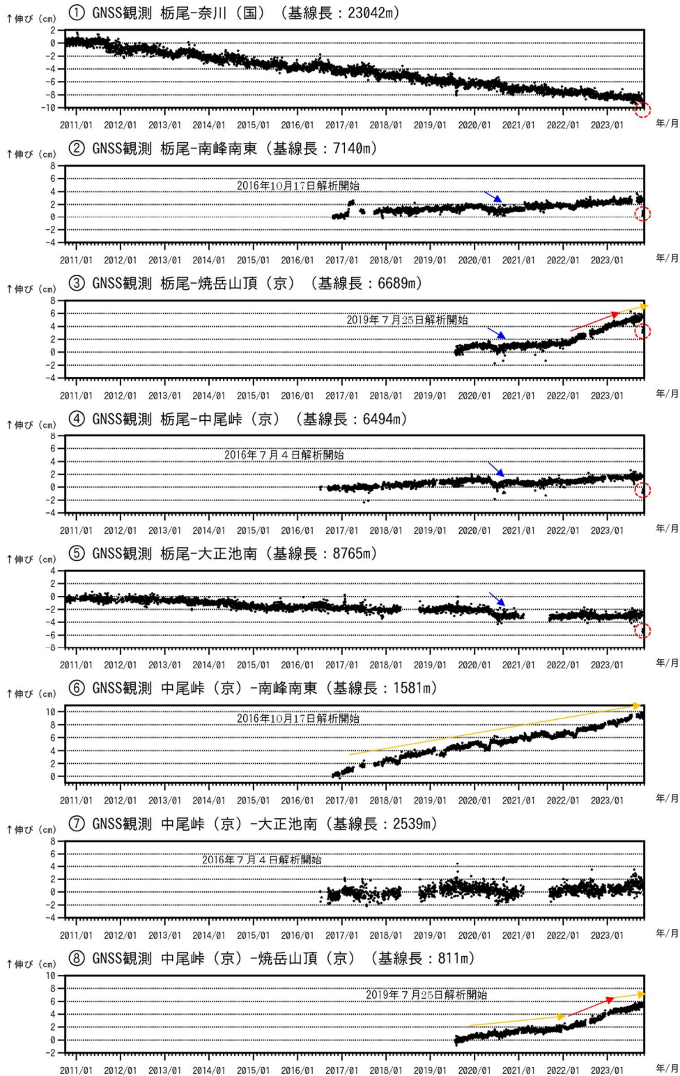
図6 焼岳 GNSS 連続観測による基線長変化 (2010年10月1日～2023年10月31日)
