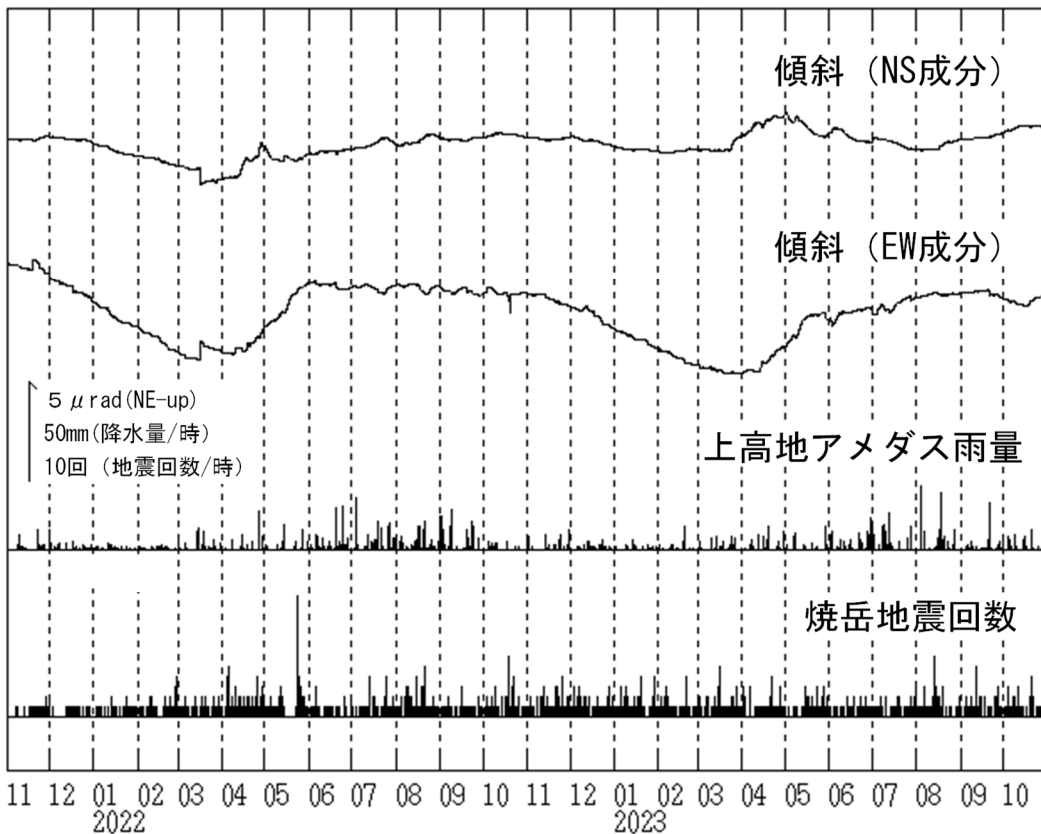
図8 焼岳 南峰南東観測点における傾斜データ（2021年11月1日～2023年10月31日）
