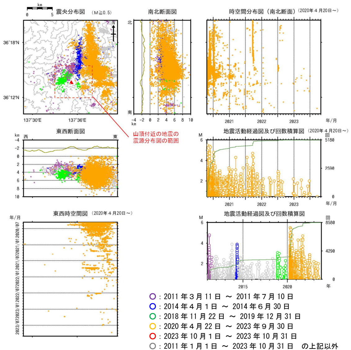
図9 焼岳 広域地震観測網による山体及び周辺の地震活動(2011年1月1日～2023年10月31日)
