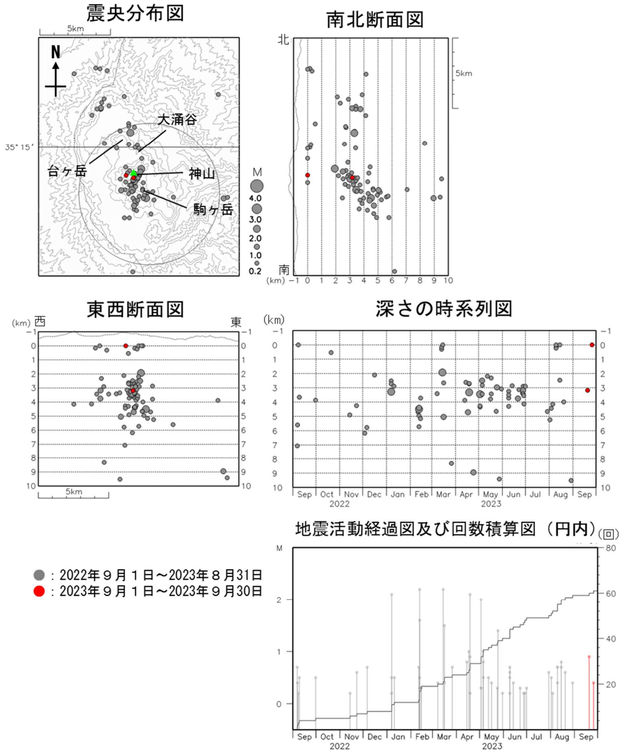
図4 箱根山 広域地震観測網による山体周辺の震源分布図（2022年9月1日～2023年9月30日）
