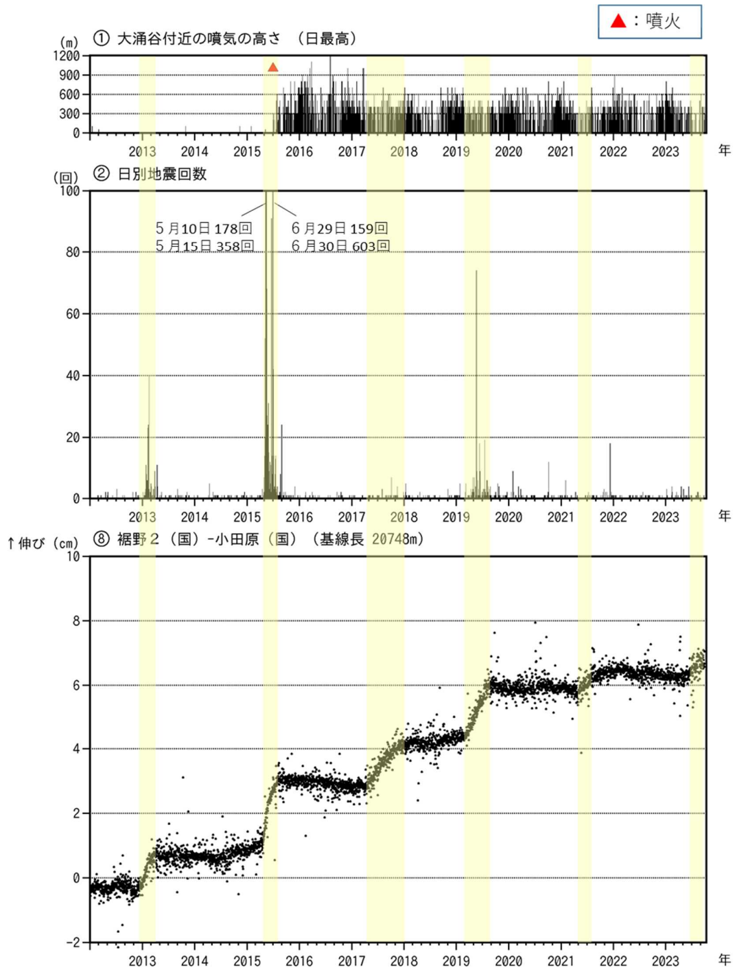
図3-1 箱根山 火山活動経過図（2012年1月1日～2023年9月30日）
