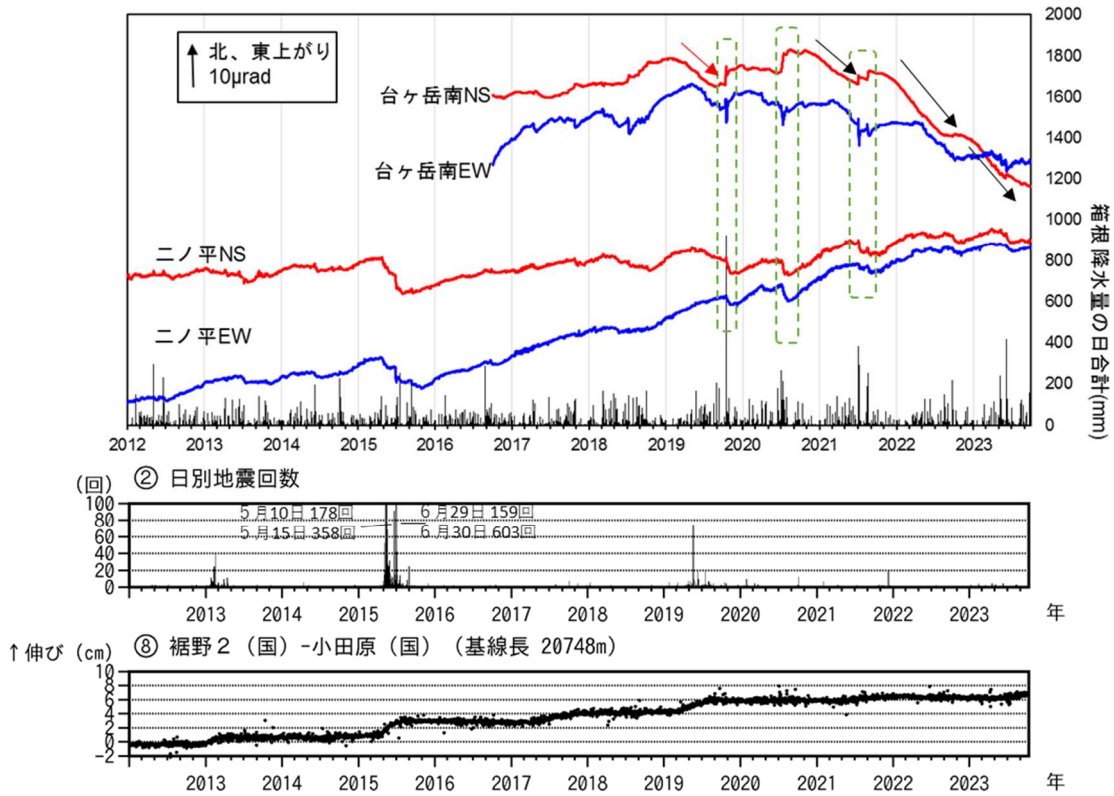
図5 箱根山 傾斜データ（2012年1月1日～2023年9月30日）
