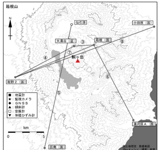
図3-2 箱根山 GNSS連続観測による基線長変化及び 観測点配置図(2012年1月1日~2023年9月30日) (国): 国土地理院 (温): 神奈川県温泉地学研究所 空白部分は欠測を示します。
