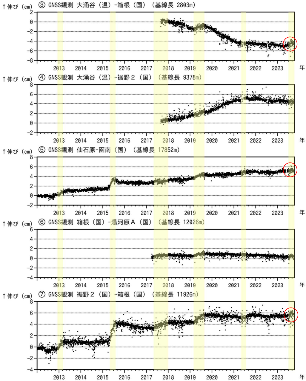
図3-2 箱根山 GNSS連続観測による基線長変化及び 観測点配置図(2012年1月1日~2023年9月30日) (国): 国土地理院 (温): 神奈川県温泉地学研究所 空白部分は欠測を示します。
