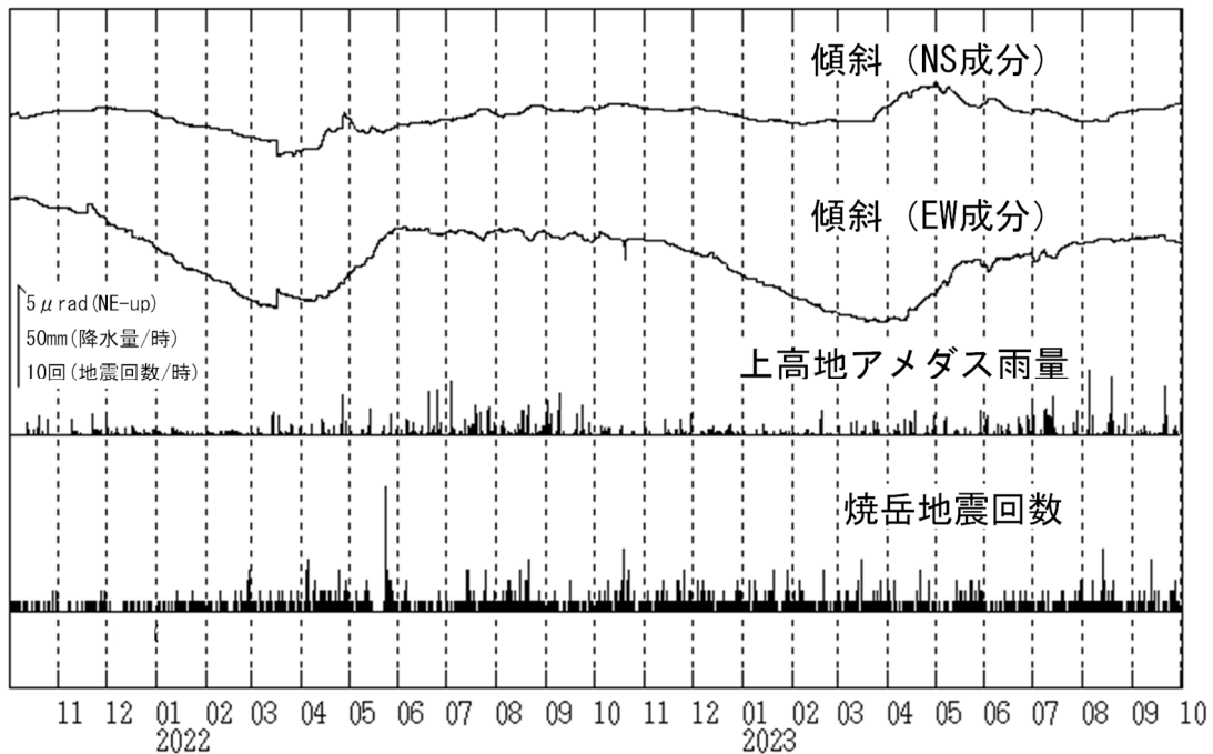
図8 焼岳 南峰南東観測点における傾斜データ (2021年10月1日～9月30日)
