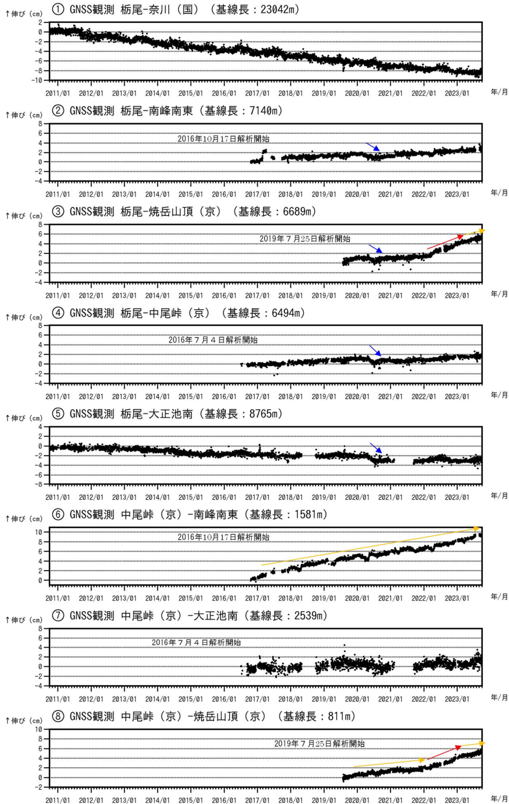
図6 焼岳 GNSS 連続観測による基線長変化（2010年10月1日～2023年9月30日）
