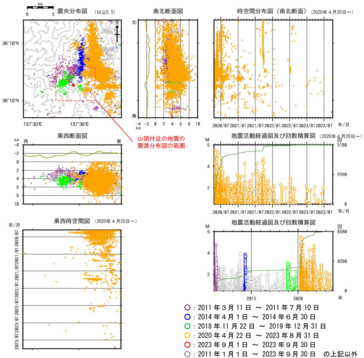
図9 焼岳 広域地震観測網による山体及び周辺の地震活動(2011年1月1日～2023年9月30日)
