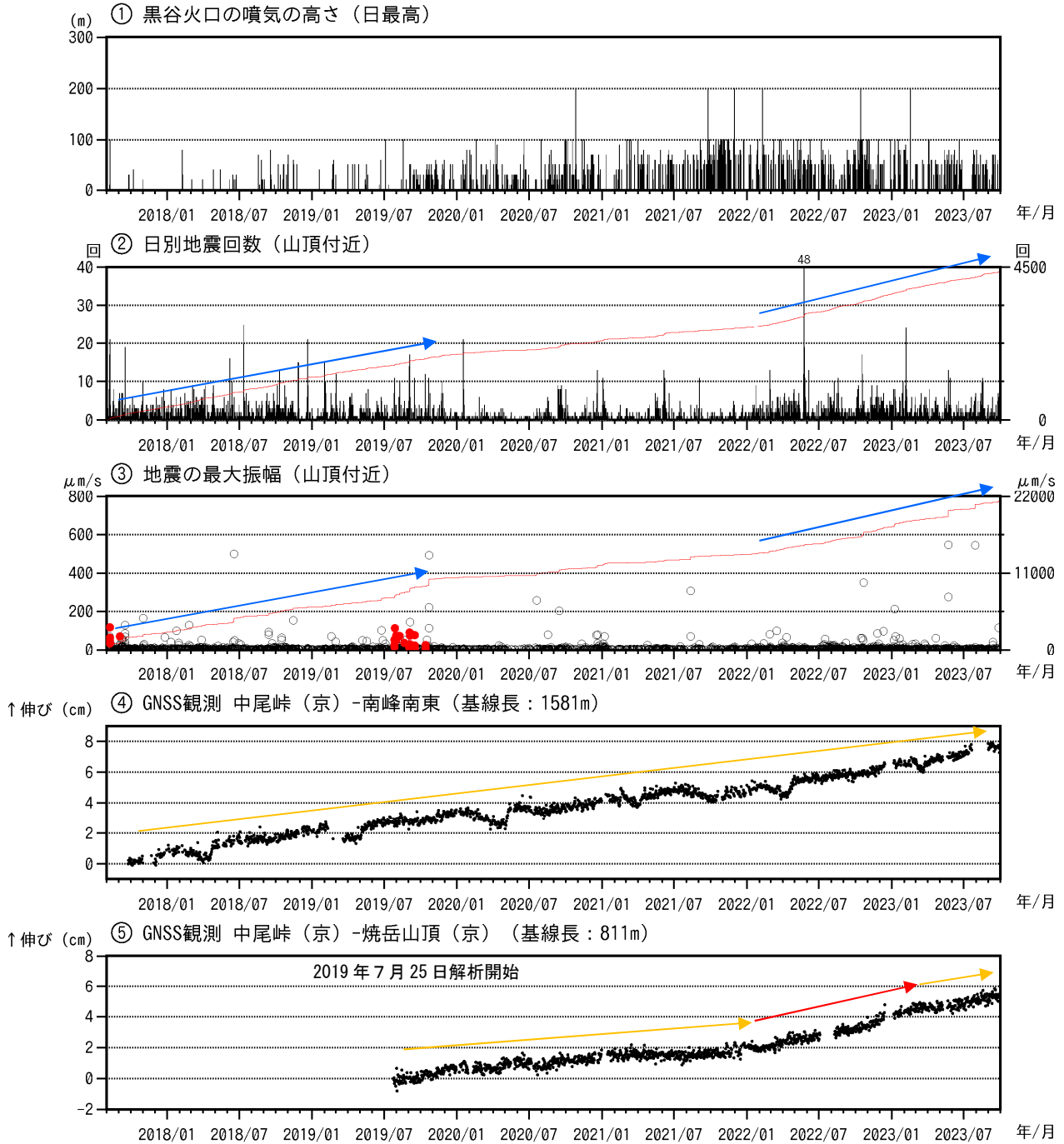
図1 焼岳 火山活動経過図（2017年9月1日～2023年9月30日）
