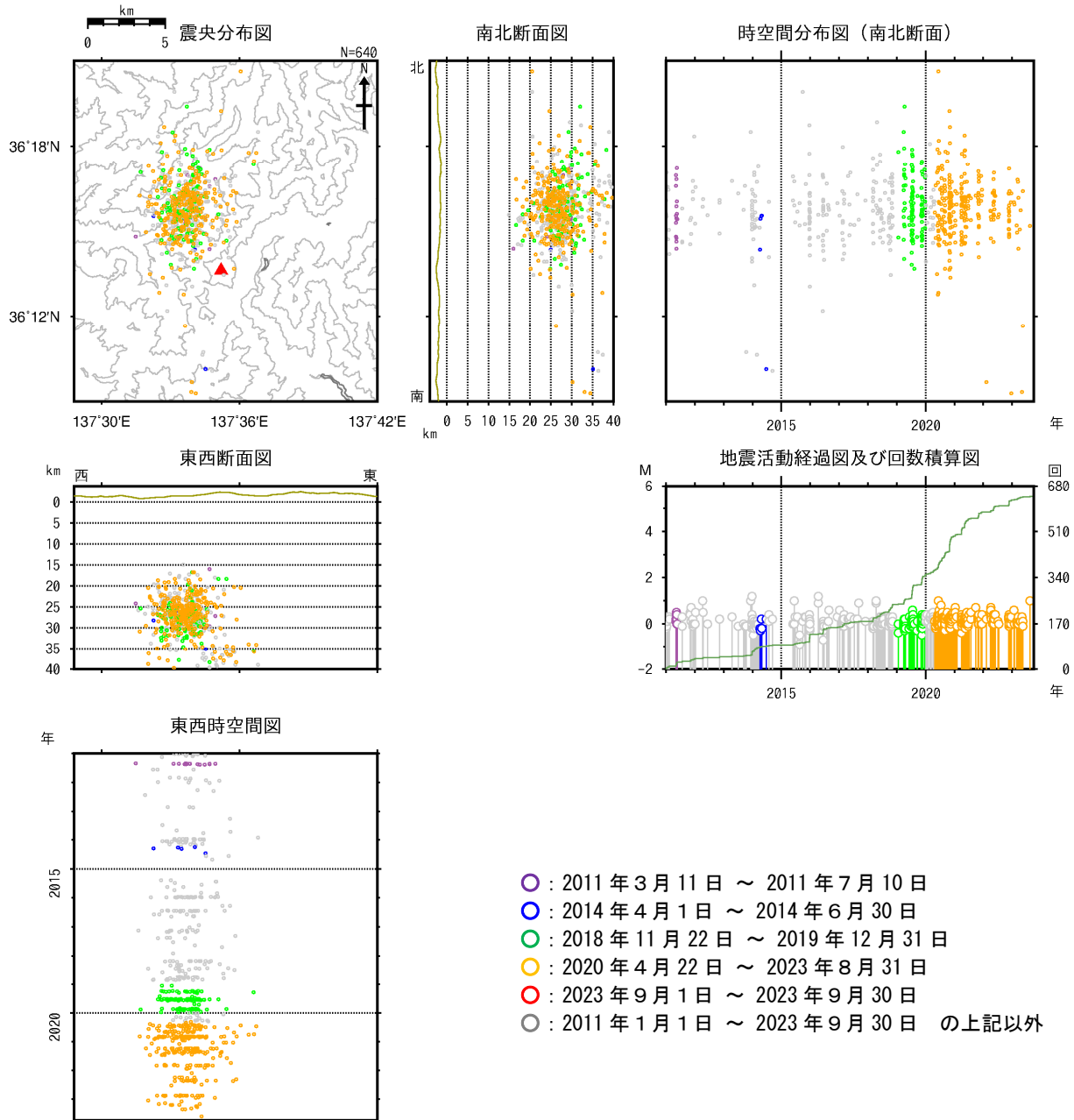
図10 焼岳 広域地震観測網による深部低周波地震の震源分布図（2011年1月1日～2023年9月30日） 広域地震観測網により震源決定したもので、深さは全て海面以下として決定しています。そのため、山頂付近の浅い地震の震源も海面下に決定されています。 M（マグニチュード）は地震の規模を表します。 図中の震源要素は一部暫定値が含まれており、後日変更することがあります。 ・焼岳の北西側の深い所を震源とする低周波地震の発生状況に特段の変化はみられません。 ・過去には、図9に示したような焼岳周辺の地震活動の活発化がみられた期間付近で、深部低周波地震が増加したことがあります。
