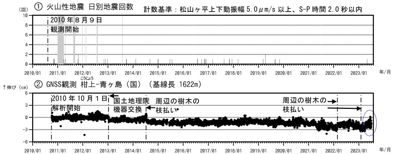
図3 青ヶ島 火山活動経過図（2010年8月9日～2023年7月31日）
