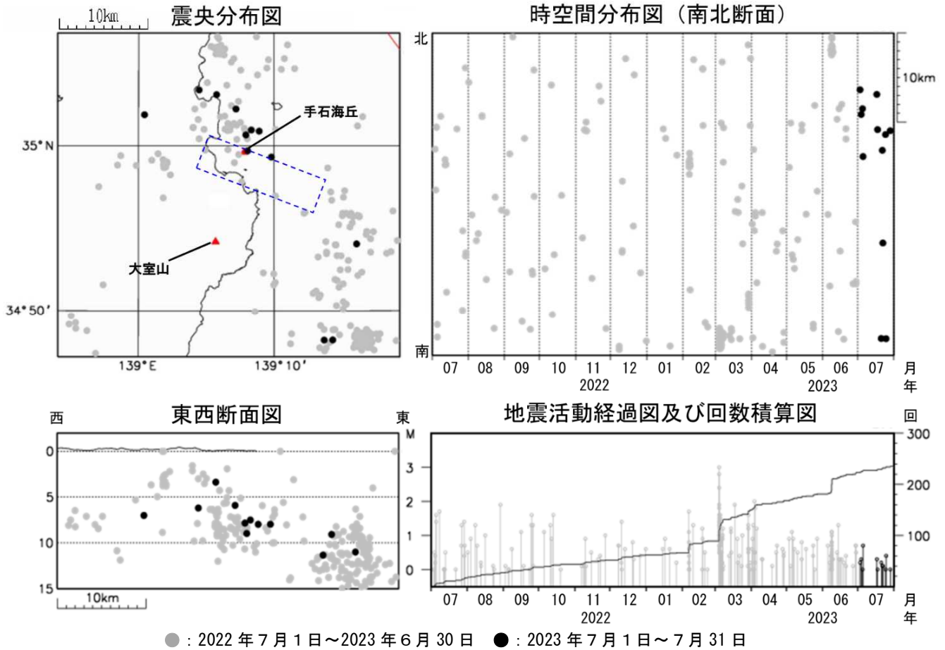
図5 伊豆東部火山群 広域地震観測網による震源分布図（2022年7月1日～2023年7月31日） □の領域は群発地震活動の発生する可能性がある範囲（火口が出現する可能性のある範囲）を示しています。 ( https://www.data.jma.go.jp/vois/data/tokyo/STOCK/level/PDF/level_316.pdf ) 広域地震観測網により震源決定したもので、深さは全て海面以下として決定しています。 M（マグニチュード）は地震の規模を表し、M0.0以上を表示しています。 図中の震源要素は一部暫定値が含まれており、後日変更することがあります。 この図では、関係機関の地震波形を一元的に処理し、地震観測点の標高を考慮する等した手法で得られた震源を用いています。
