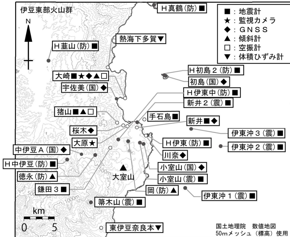
図7 伊豆東部火山群 GNSS 連続観測点配置図 図中の GNSS 基線②～⑧は図6の②～⑧に対応しています。
