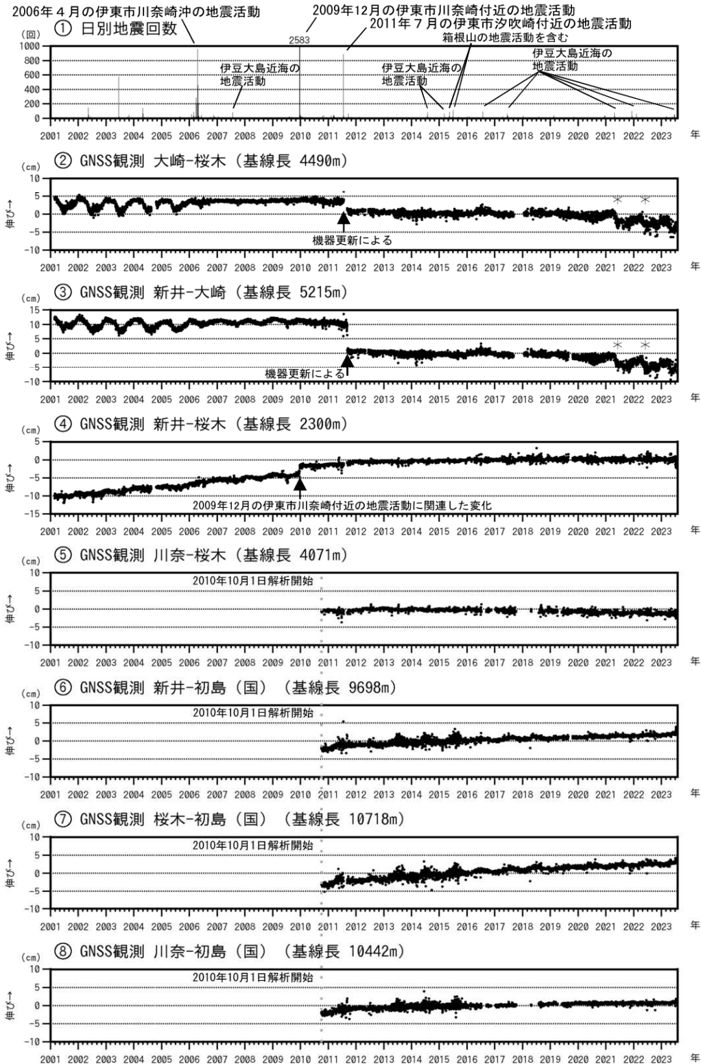
図6 伊豆東部火山群 火山活動経過図 (2001年2月1日~2023年7月31日)
