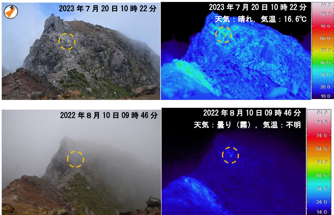
図6 焼岳 北峰東斜面の地表面温度分布
