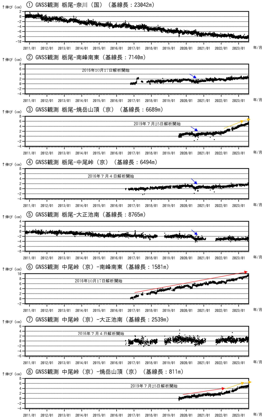
図10 焼岳 GNSS連続観測による基線長変化 (2010年10月1日~2023年7月31日)
