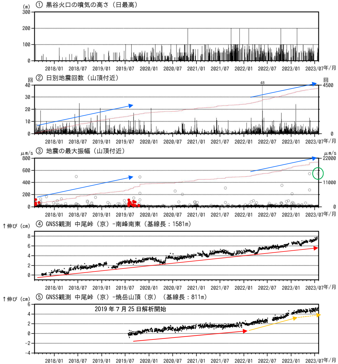
図1 焼岳 火山活動経過図（2017年8月1日～2023年7月31日）
