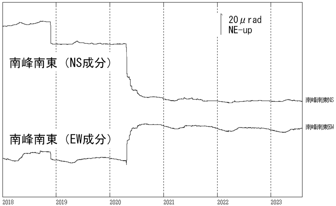
図 12 焼岳 南峰南東観測点における傾斜データ (2018年1月1日～2023年7月31日)
