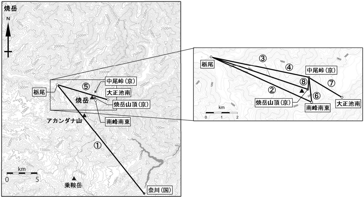
図 11 焼岳 GNSS 連続観測点配置
