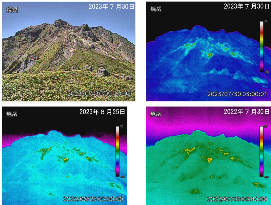
図4 焼岳 中尾峠赤外熱映像カメラによる焼岳の北側斜面の地表面温度分布と可視画像 撮影場所と撮影方向は図15を参照下さい。 ・前月（左下図）及び前年（右下図）と比較して、噴気の状態や地表面温度分布に特段の変化はありません。
