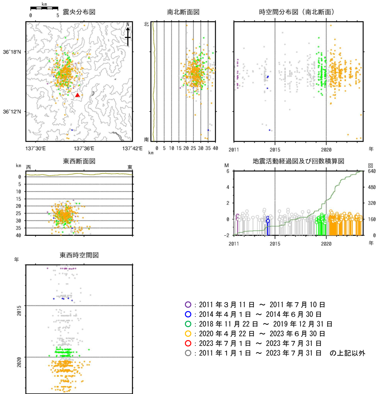
図14 焼岳 広域地震観測網による深部低周波地震の震源分布図（2011年1月1日～2023年7月31日） 広域地震観測網により震源決定したもので、深さは全て海面以下として決定しています。そのため、山頂付近の浅い地震の震源も海面下に決定されています。 M（マグニチュード）は地震の規模を表します。 図中の震源要素は一部暫定値が含まれており、後日変更することがあります。 ・ 焼岳の北西側の深い所を震源とする低周波地震の発生状況に特段の変化はみられません。 ・ 過去には、図13に示したような焼岳周辺の地震活動の活発化がみられた期間付近で、深部低周波地震が増加したことがあります。
