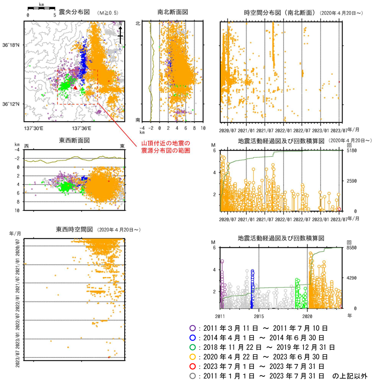
図13 焼岳 広域地震観測網による山体及び周辺の地震活動(2011年1月1日～2023年7月31日)
