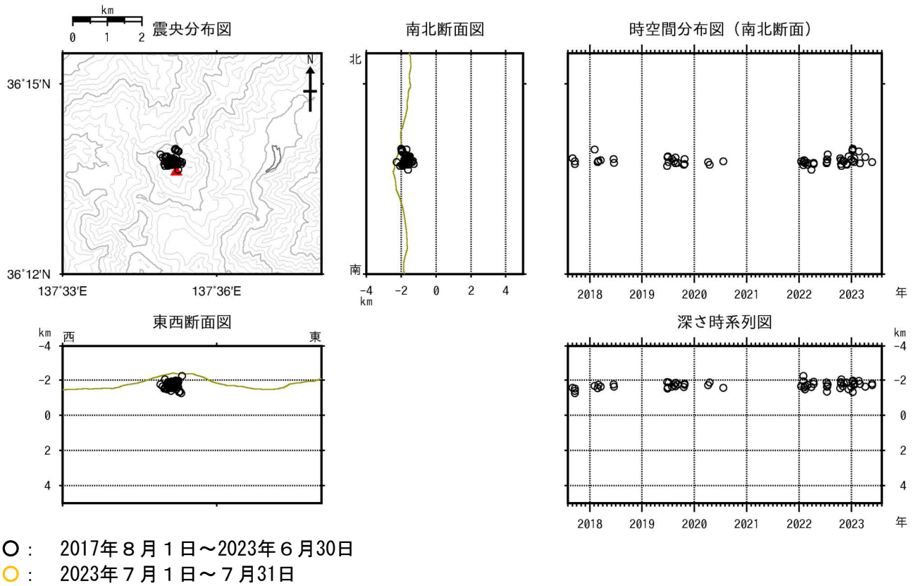
図2 焼岳 山頂付近の地震の震源分布図（2017年8月1日～2023年7月31日）
