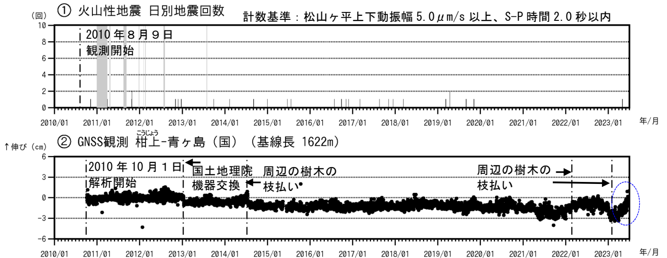
図3 青ヶ島 火山活動経過図（2010年8月9日～2023年6月30日）
