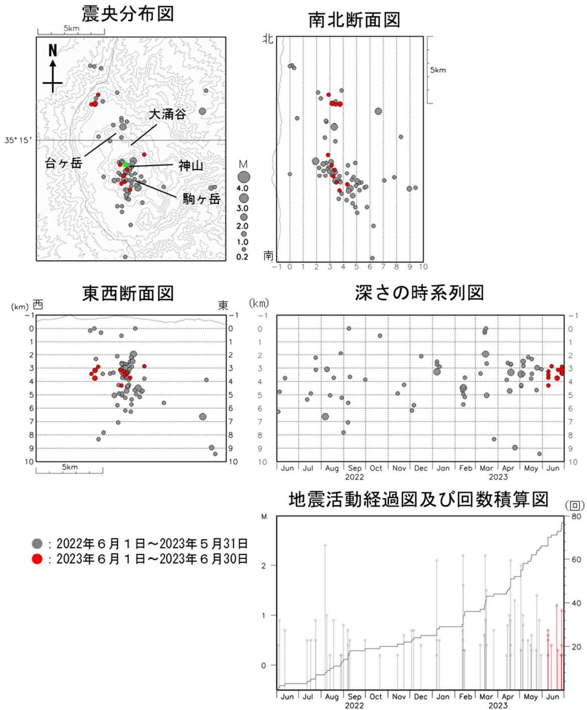
図4 箱根山 広域地震観測網による山体周辺の震源分布図（2022年6月1日～2023年6月30日） M（マグニチュード）は地震の規模を表し、M0.2以上の地震を表示しています。 広域地震観測網により震源決定したもので、深さは全て海面以下として決定しています。 図中の震源要素は一部暫定値が含まれており、後日変更することがあります。 この図では、関係機関の地震波形を一元的に処理し、地震観測点の標高を考慮する等した手法で得られた震源を用いています。 火山性地震は少なく地震活動は低調に経過しました。 震源は主に神山から駒ヶ岳にかけての深さ3～4km及び大涌谷の北西4km付近の深さ3～4kmに決まりました。
