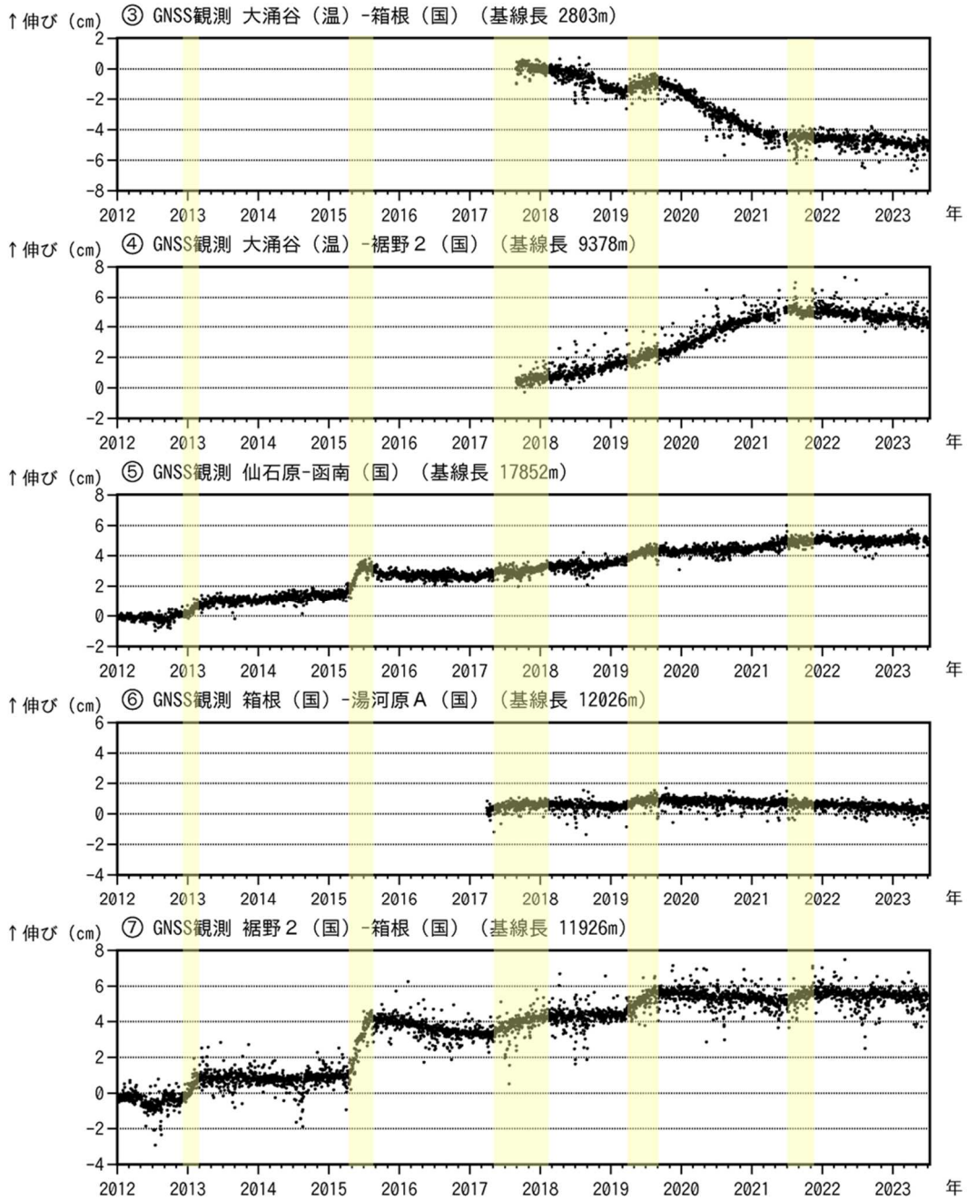
図3-2 箱根山 GNSS連続観測による基線長変化及び
