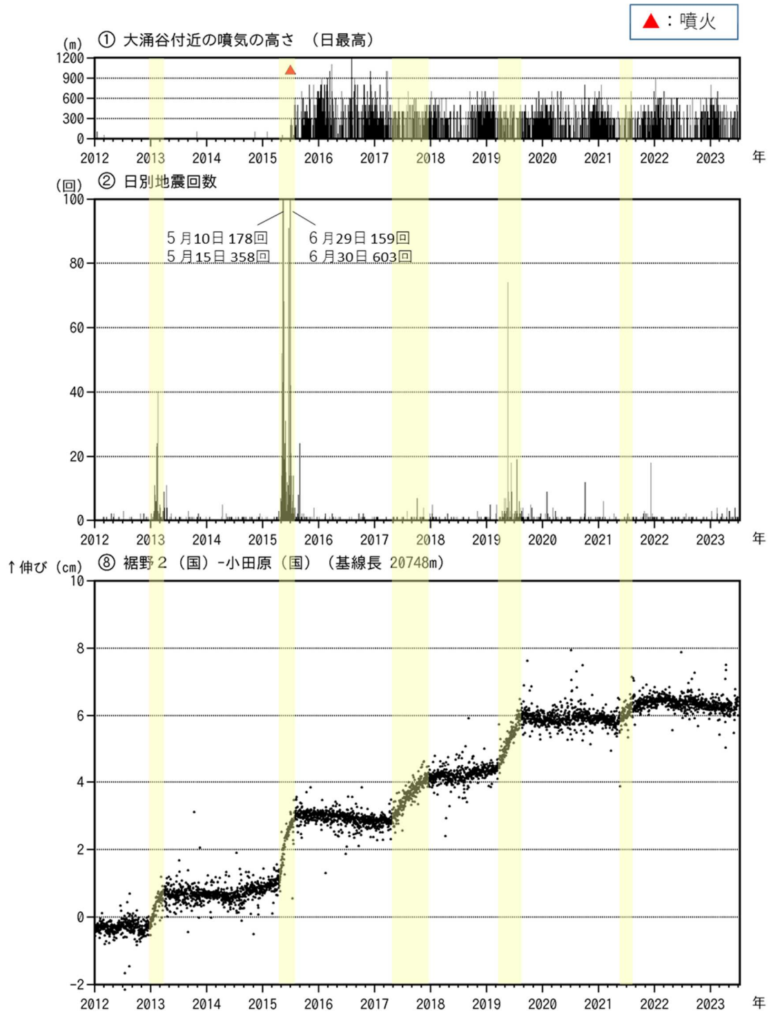
図3-1 箱根山 火山活動経過図（2012年1月1日～2023年6月30日）
