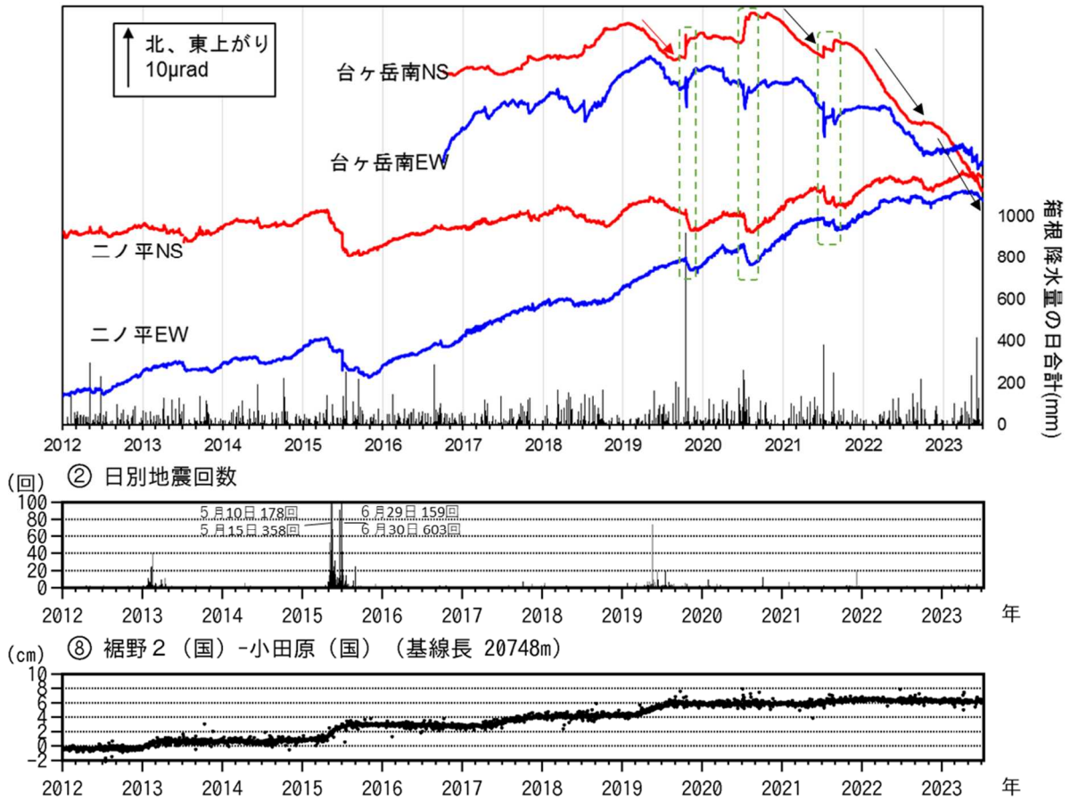
図5 箱根山 傾斜データ（2012年1月1日～2023年6月30日）
