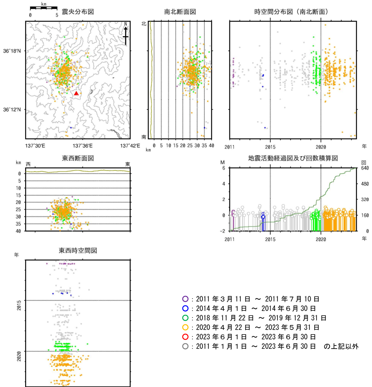
図10 焼岳 広域地震観測網による深部低周波地震の震源分布図（2011年1月1日～2023年6月30日）
