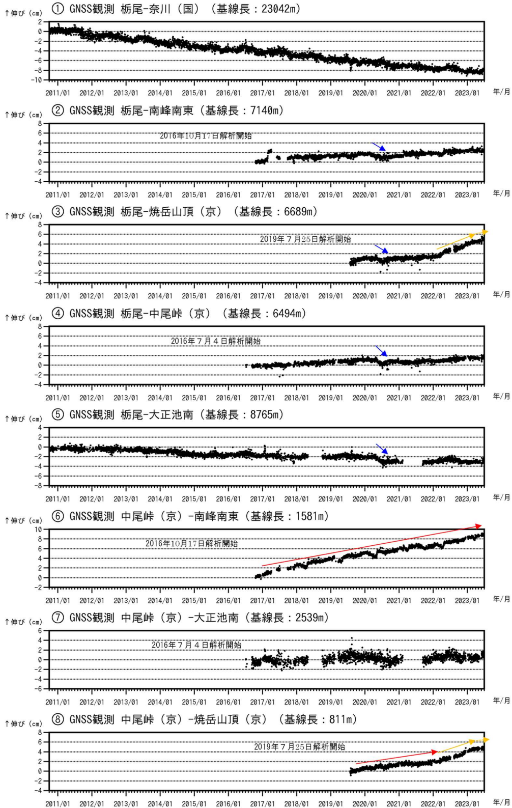
図6 焼岳 GNSS 連続観測による基線長変化 (2010年10月1日~2023年6月30日)
