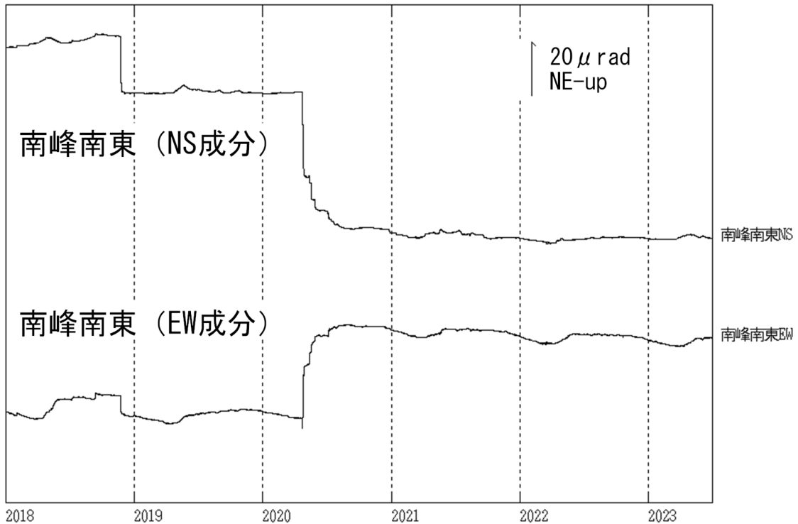
図8 焼岳 南峰南東観測点における傾斜データ（2018年1月1日～2023年6月30日）
