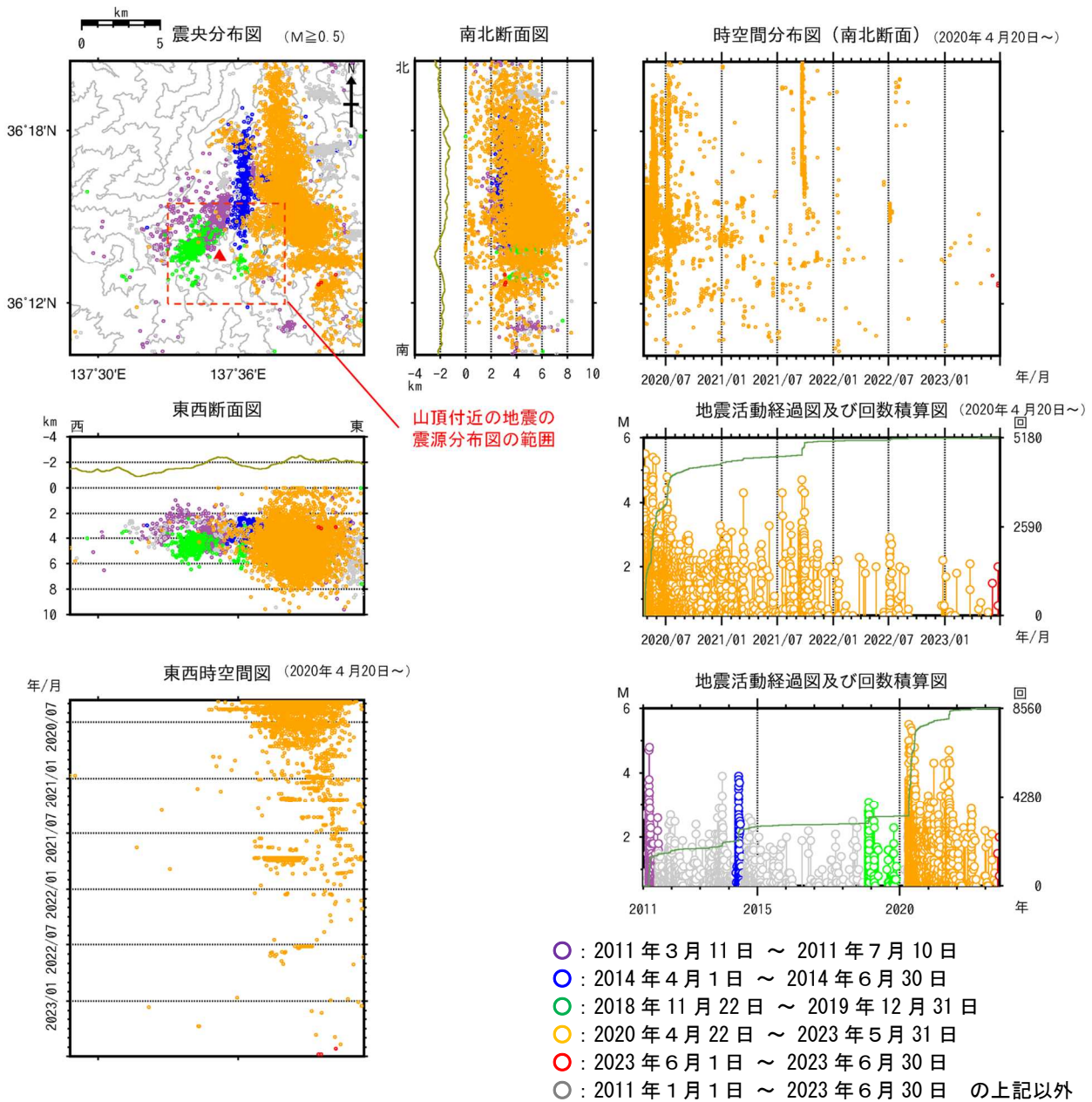
図9 焼岳 広域地震観測網による山体及び周辺の地震活動(2011年1月1日～2023年6月30日)
