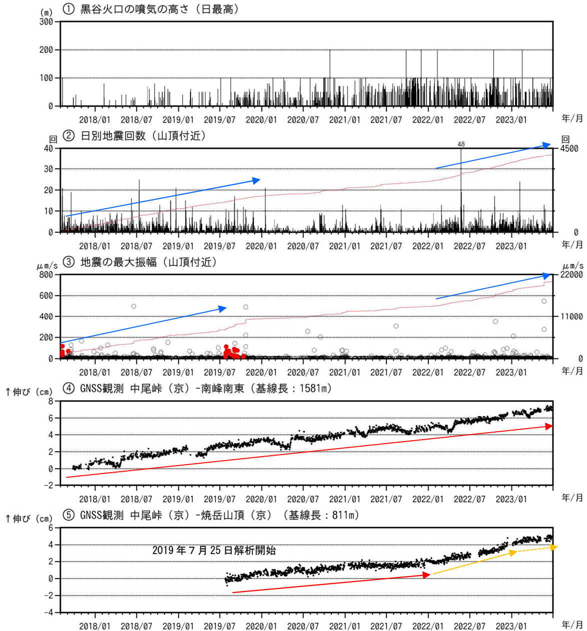
図1 焼岳 火山活動経過図（2017年8月1日～2023年6月30日）
