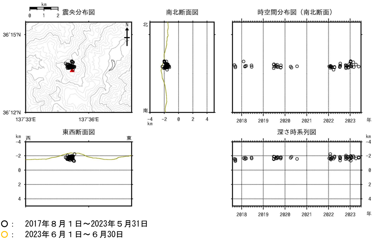
図2 焼岳 山頂付近の地震の震源分布図（2017年8月1日～2023年6月30日）
