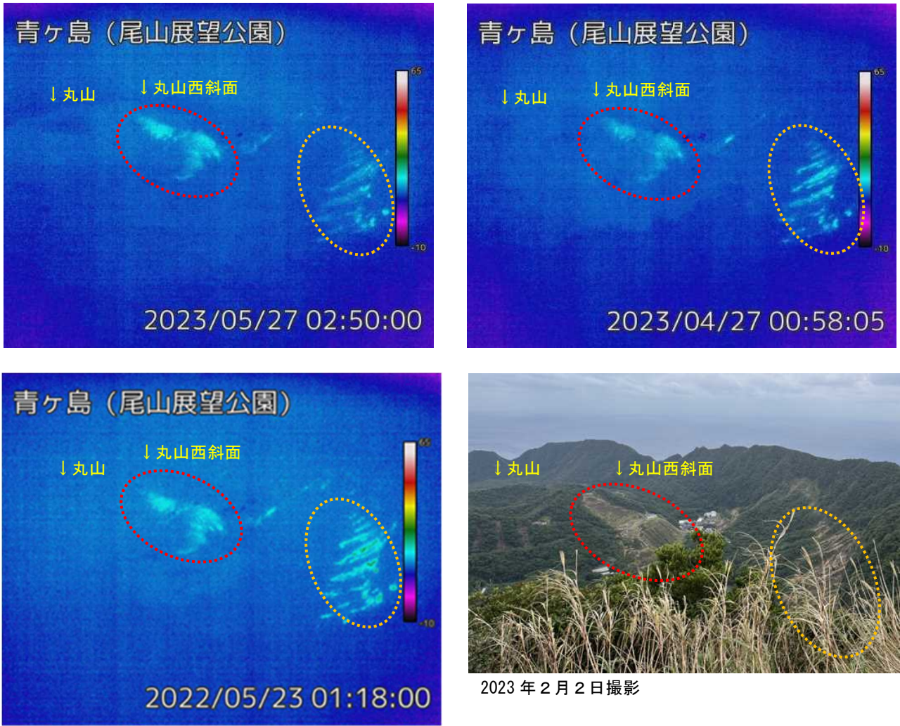
図2 青ヶ島 カルデラ内の地表面温度の状況（左上, 右上, 左下：尾山展望公園監視カメラによる、右下：2023年2月2日に撮影した同場所からの写真）
