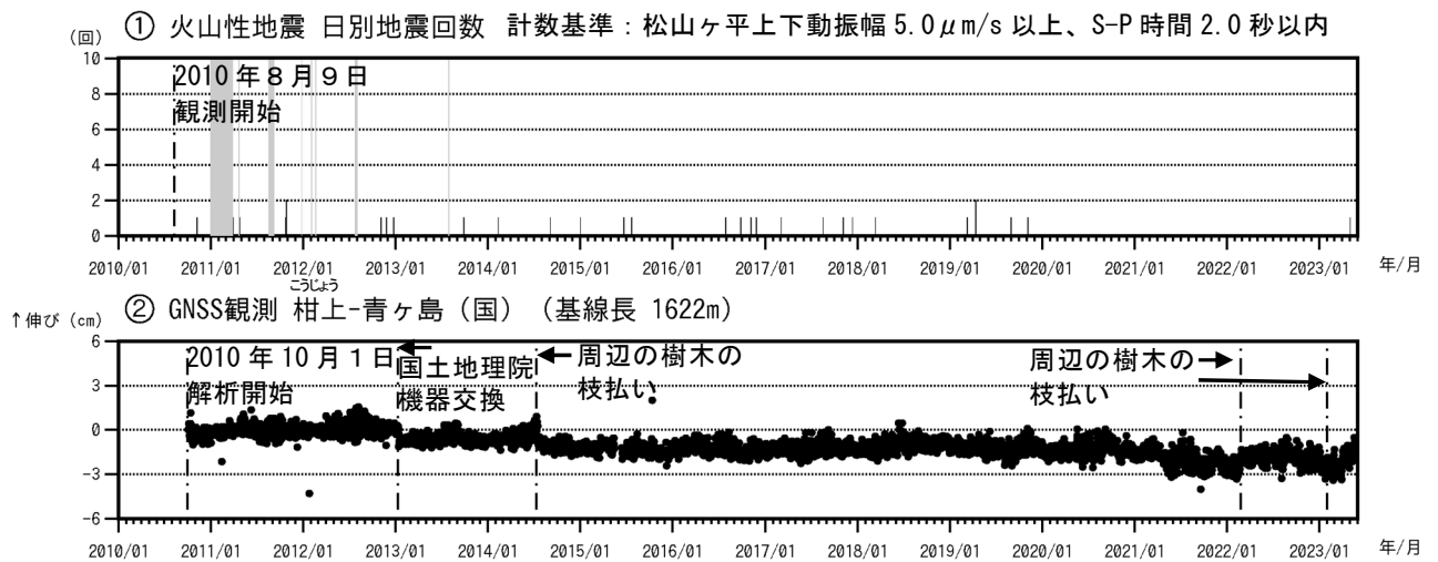
図3 青ヶ島 火山活動経過図（2010年8月9日～2023年5月31日）
