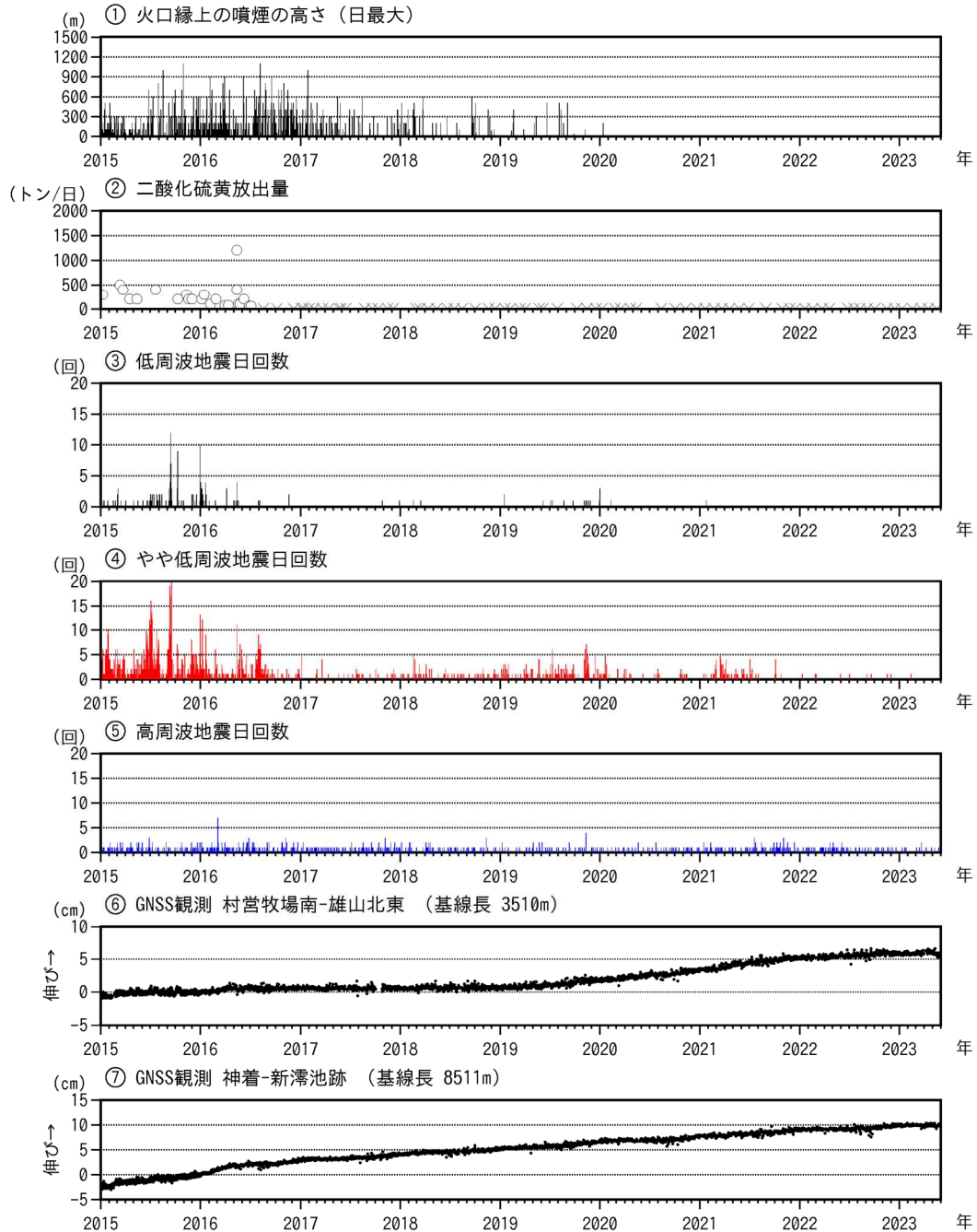
図6 三宅島 火山活動経過図（2015年1月1日～2023年5月31日）
