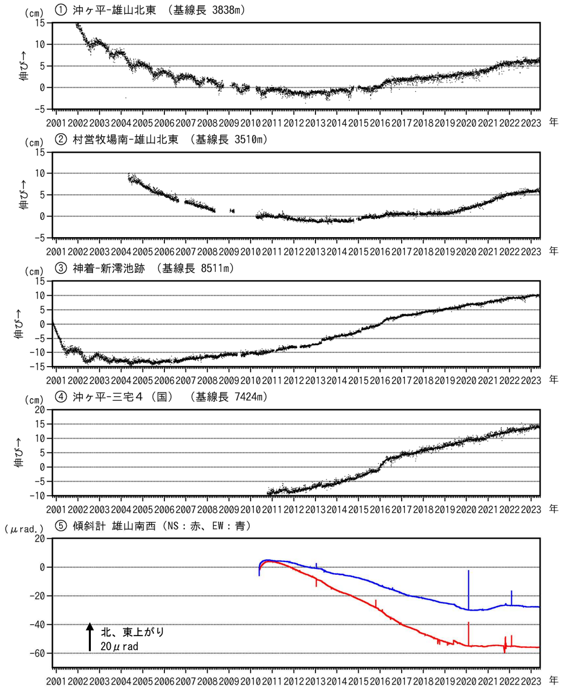
図8 三宅島 GNSS 連続観測及び傾斜計観測結果（2000年10月26日～2023年5月31日）
