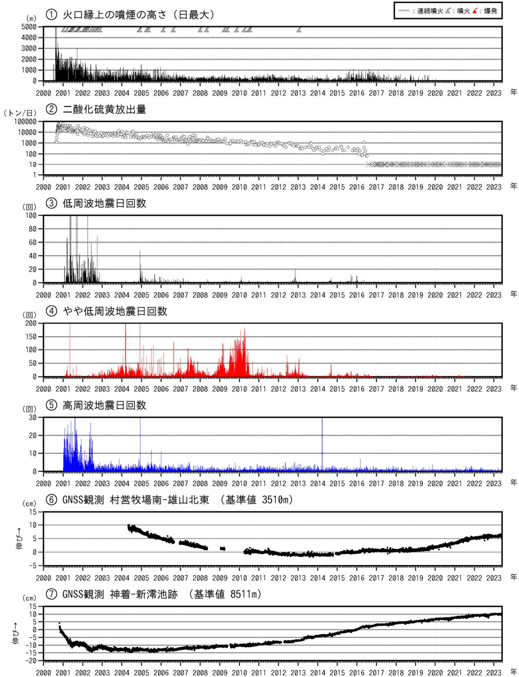
図7 三宅島 長期の火山活動経過図（2000年1月1日～2023年5月31日）
