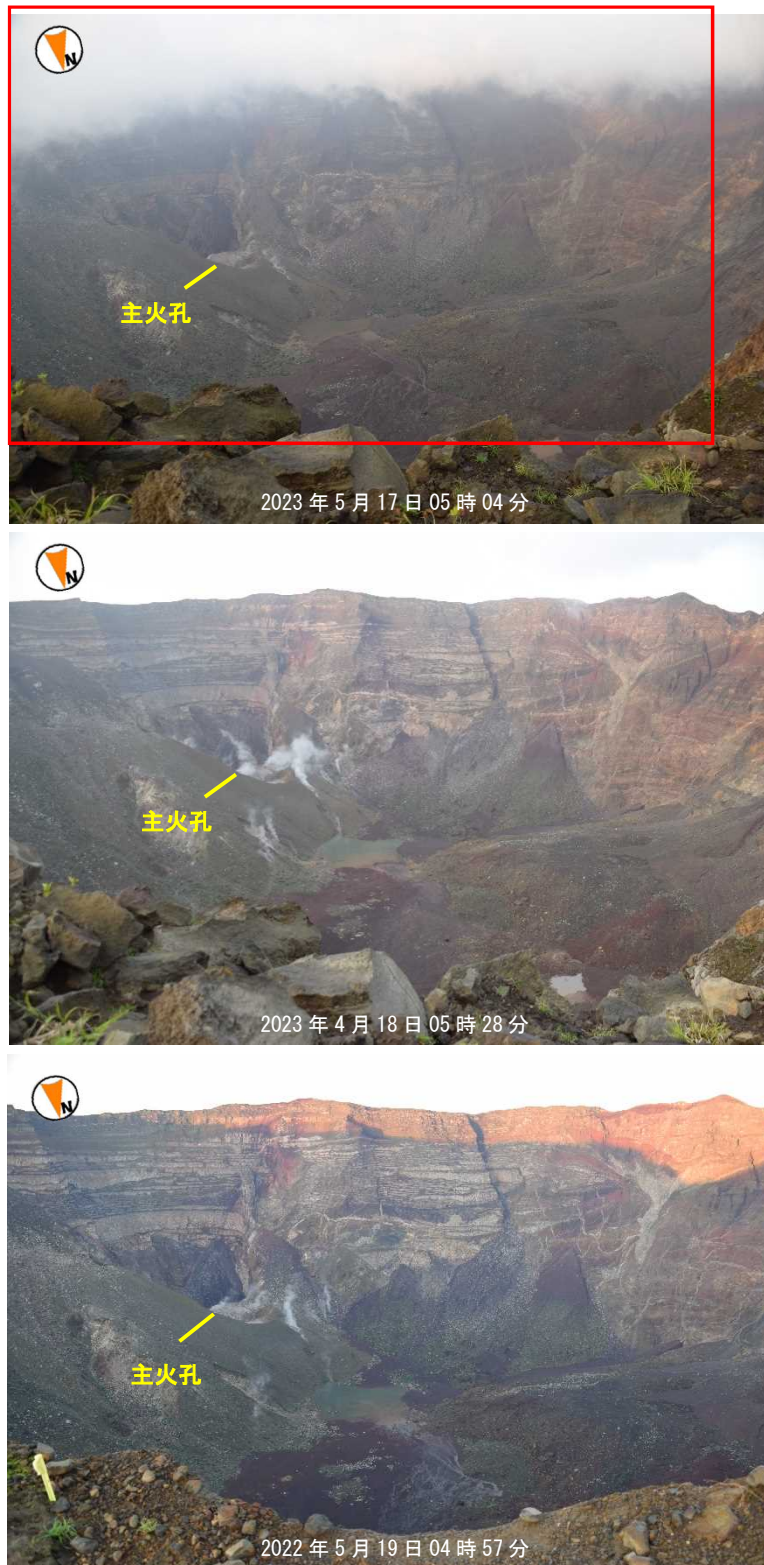
図4 三宅島 山頂火口内の状況（スオウ穴から撮影） ※図中の赤四角は図5の赤外熱映像の範囲を示しています。
