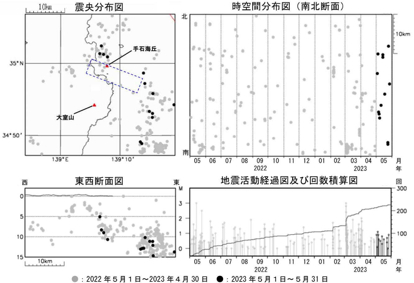
図2 伊豆東部火山群 広域地震観測網による震源分布図（2022年5月1日～2023年5月31日） □の領域は群発地震活動の発生する可能性がある範囲（火口が出現する可能性のある範囲）を示しています。 ( https://www.data.jma.go.jp/vois/data/tokyo/STOCK/level/PDF/level_316.pdf ) 広域地震観測網により震源決定したもので、深さは全て海面以下として決定しています。 M（マグニチュード）は地震の規模を表し、M0.0以上を表示しています。 図中の震源要素は一部暫定値が含まれており、後日変更することがあります。 この図では、関係機関の地震波形を一元的に処理し、地震観測点の標高を考慮する等した手法で得られた震源を用いています。
