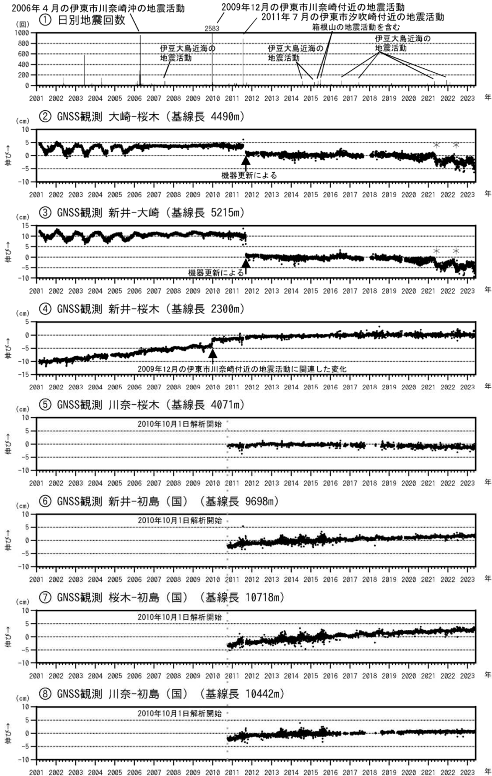
図3 伊豆東部火山群 火山活動経過図（2001年2月1日～2023年5月31日）
