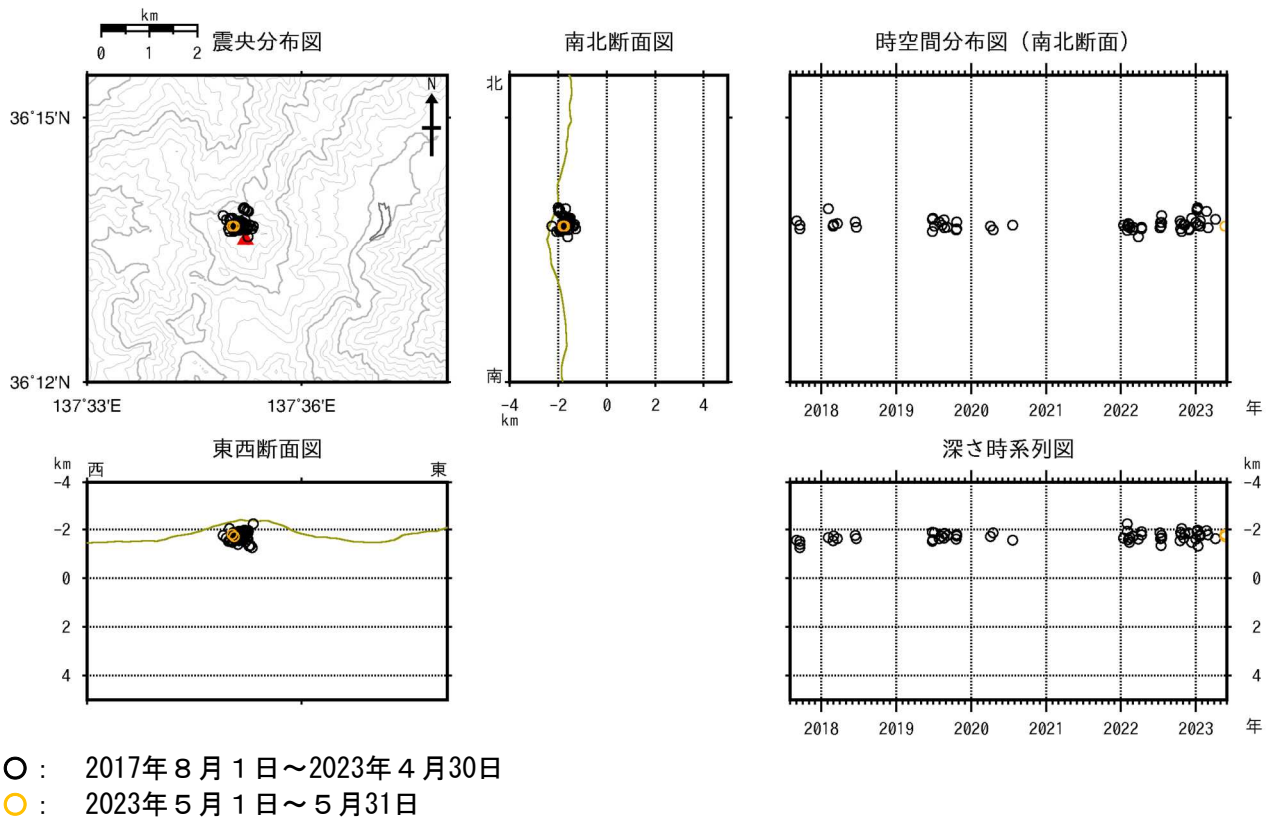
図2 焼岳 山頂付近の地震の震源分布図（2017年8月1日～2023年5月31日）
