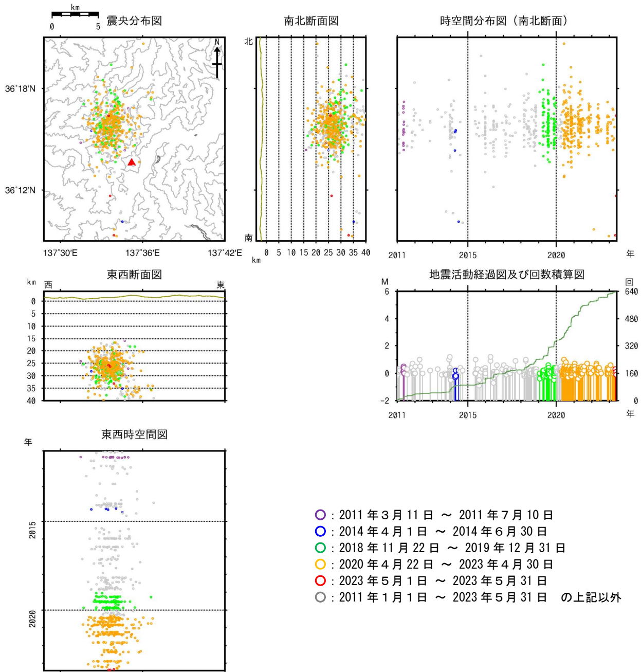
図10 焼岳 広域地震観測網による深部低周波地震の震源分布図（2011年1月1日～2023年5月31日）
