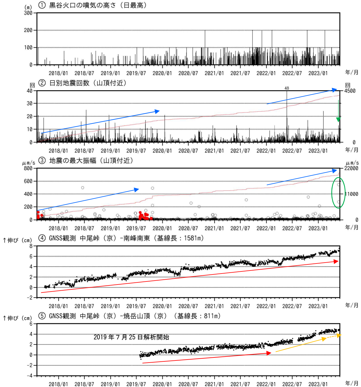
図1 焼岳 火山活動経過図（2017年8月1日～2023年5月31日）
