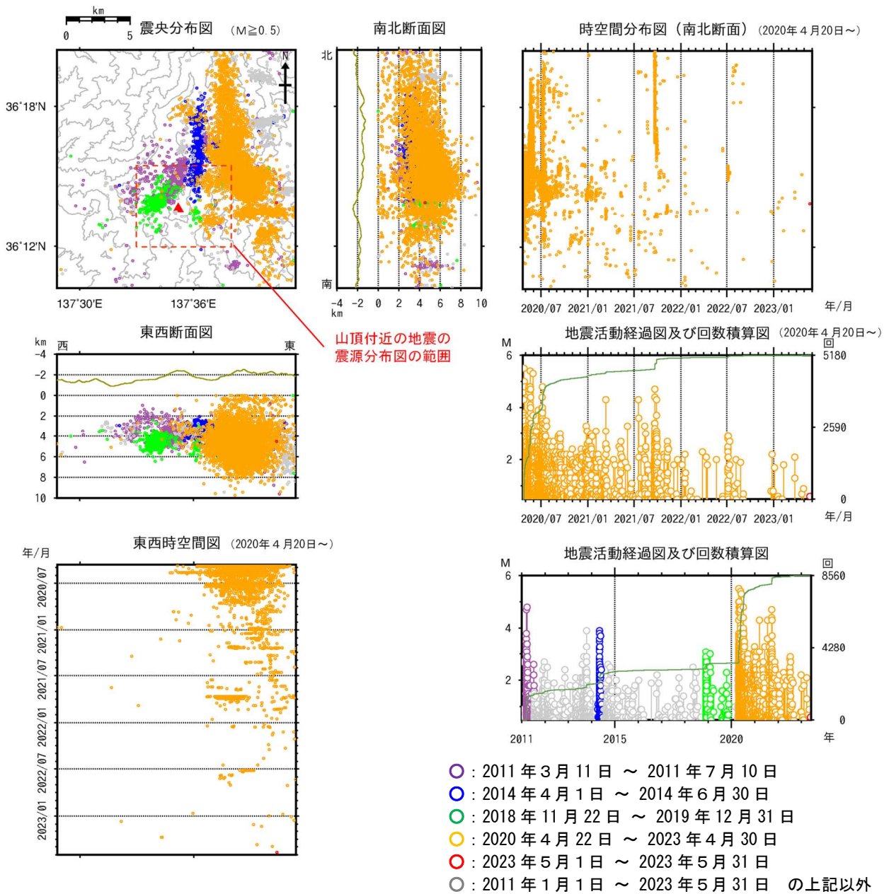
図9 焼岳 広域地震観測網による山体及び周辺の地震活動(2011年1月1日～2023年5月31日)
