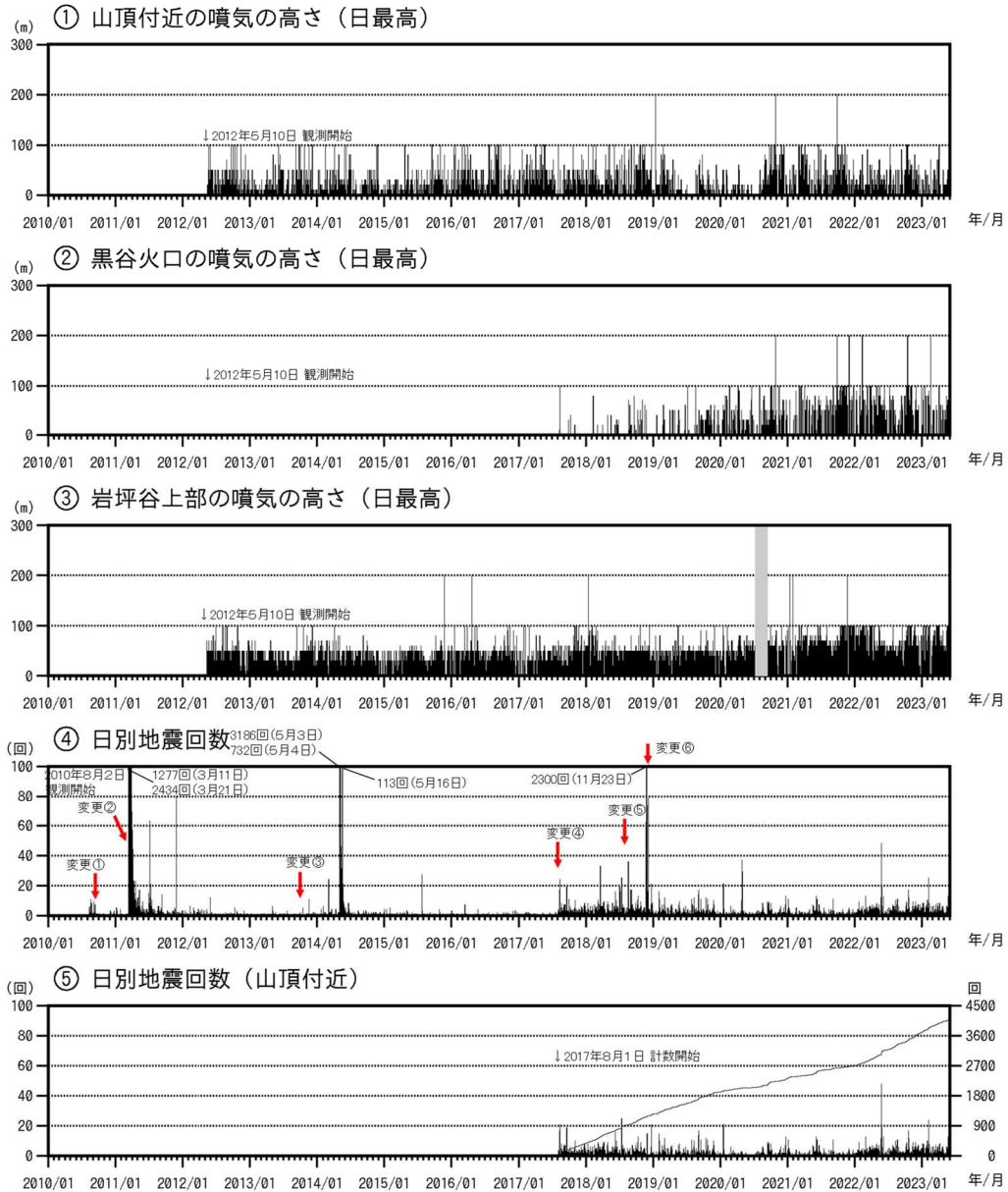
図5 焼岳 噴気の高さと地震回数の推移(2010年8月2日～2023年5月31日)
