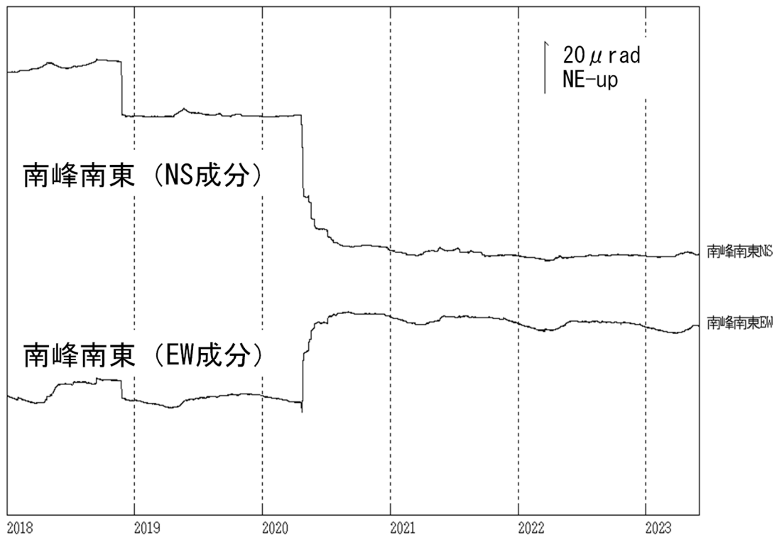
図8 焼岳 南峰南東観測点における傾斜データ（2018年1月1日～2023年5月31日）
