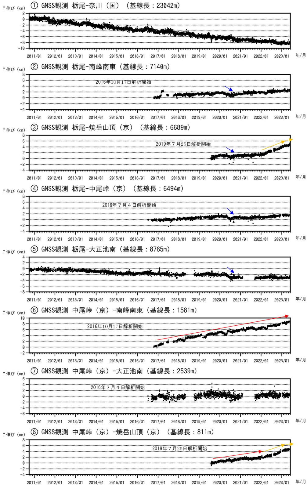
図6 焼岳 GNSS連続観測による基線長変化（2010年10月1日～2023年5月31日）
