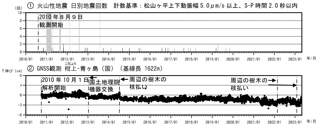
図3 青ヶ島 火山活動経過図（2010年8月9日～2023年4月30日）
