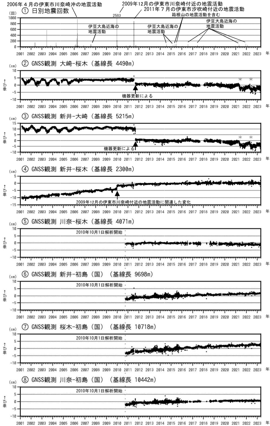
図3 伊豆東部火山群 火山活動経過図（2001年2月1日～2023年4月30日）
