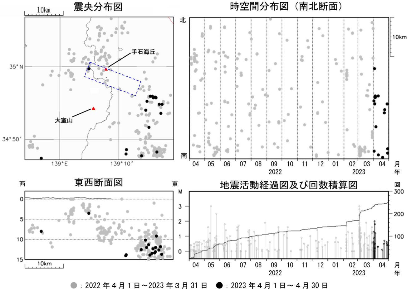
図2 伊豆東部火山群 広域地震観測網による震源分布図（2022年4月1日～2023年4月30日） □の領域は群発地震活動の発生する可能性がある範囲（火口が出現する可能性のある範囲）を示しています。 ( https://www.data.jma.go.jp/vois/data/tokyo/STOCK/level/PDF/level_316.pdf ) 広域地震観測網により震源決定したもので、深さは全て海面以下として決定しています。 M（マグニチュード）は地震の規模を表し、M0.0以上を表示しています。 図中の震源要素は一部暫定値が含まれており、後日変更することがあります。 この図では、関係機関の地震波形を一元的に処理し、地震観測点の標高を考慮する等した手法で得られた震源を用いています。
