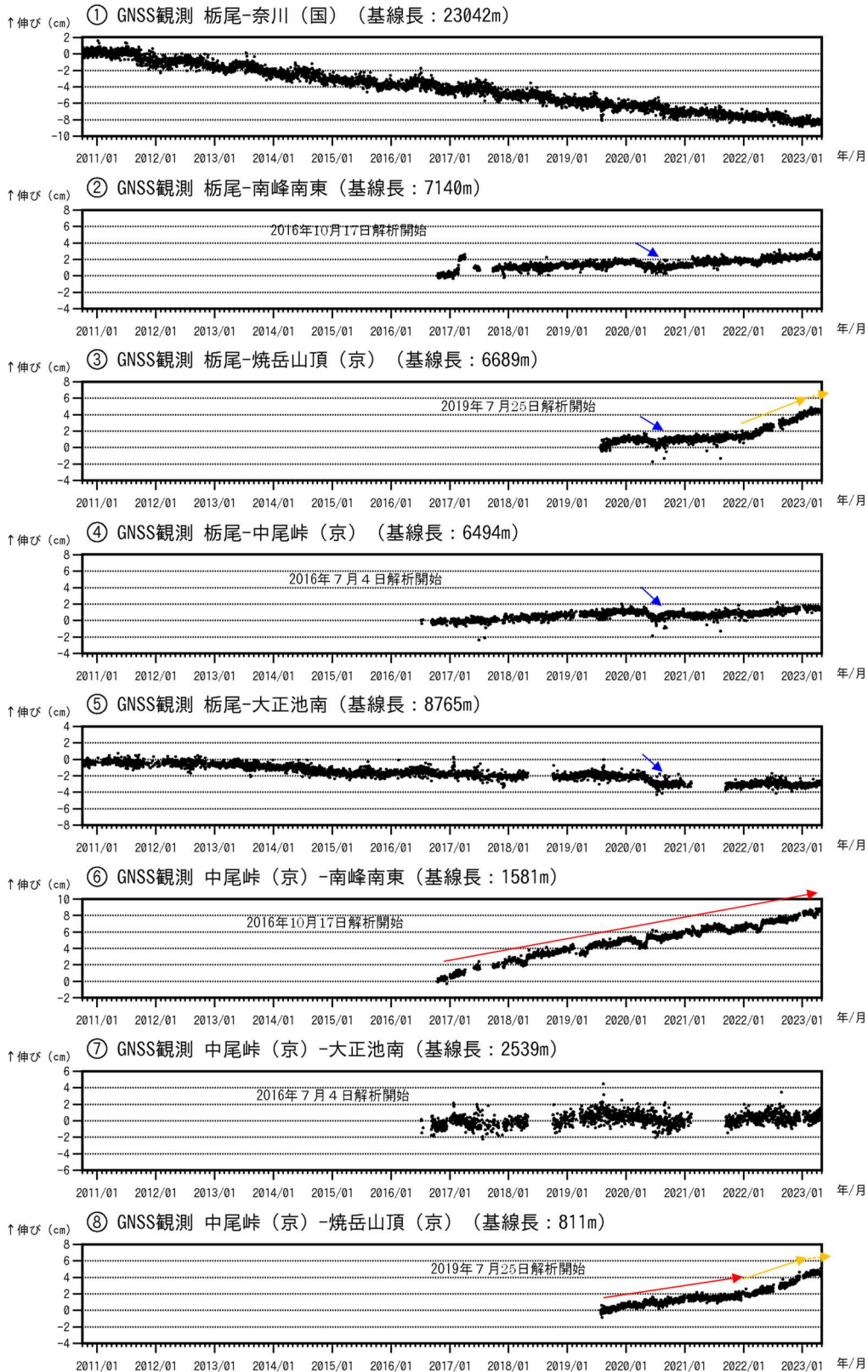
図6 焼岳 GNSS連続観測による基線長変化（2010年10月1日～2023年4月30日）
