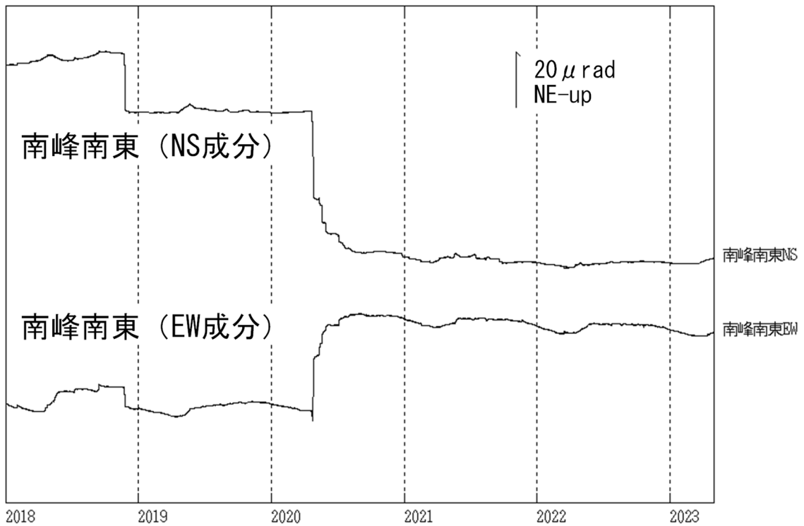
図8 焼岳 南峰南東観測点における傾斜データ（2018年1月1日～2023年4月30日）
