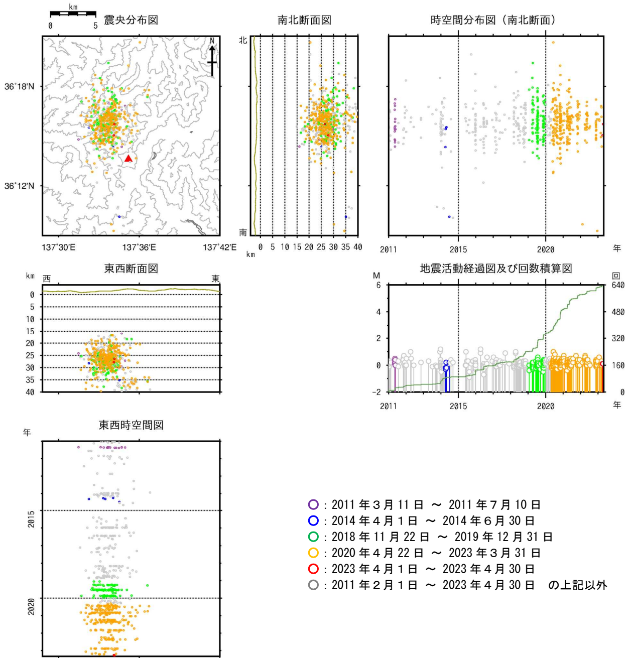
図10 焼岳 広域地震観測網による深部低周波地震の震源分布図（2011年1月1日～2023年4月30日） 広域地震観測網により震源決定したもので、深さは全て海面以下として決定しています。そのため、山頂付近の浅い地震の震源も海面下に決定されています。 M（マグニチュード）は地震の規模を表します。 図中の震源要素は一部暫定値が含まれており、後日変更することがあります。
