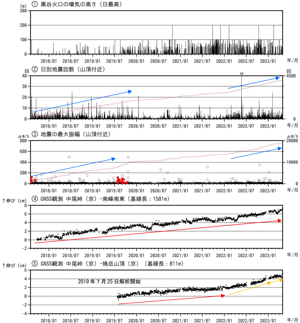
図1 焼岳 火山活動経過図（2017年8月1日～2023年4月30日）
