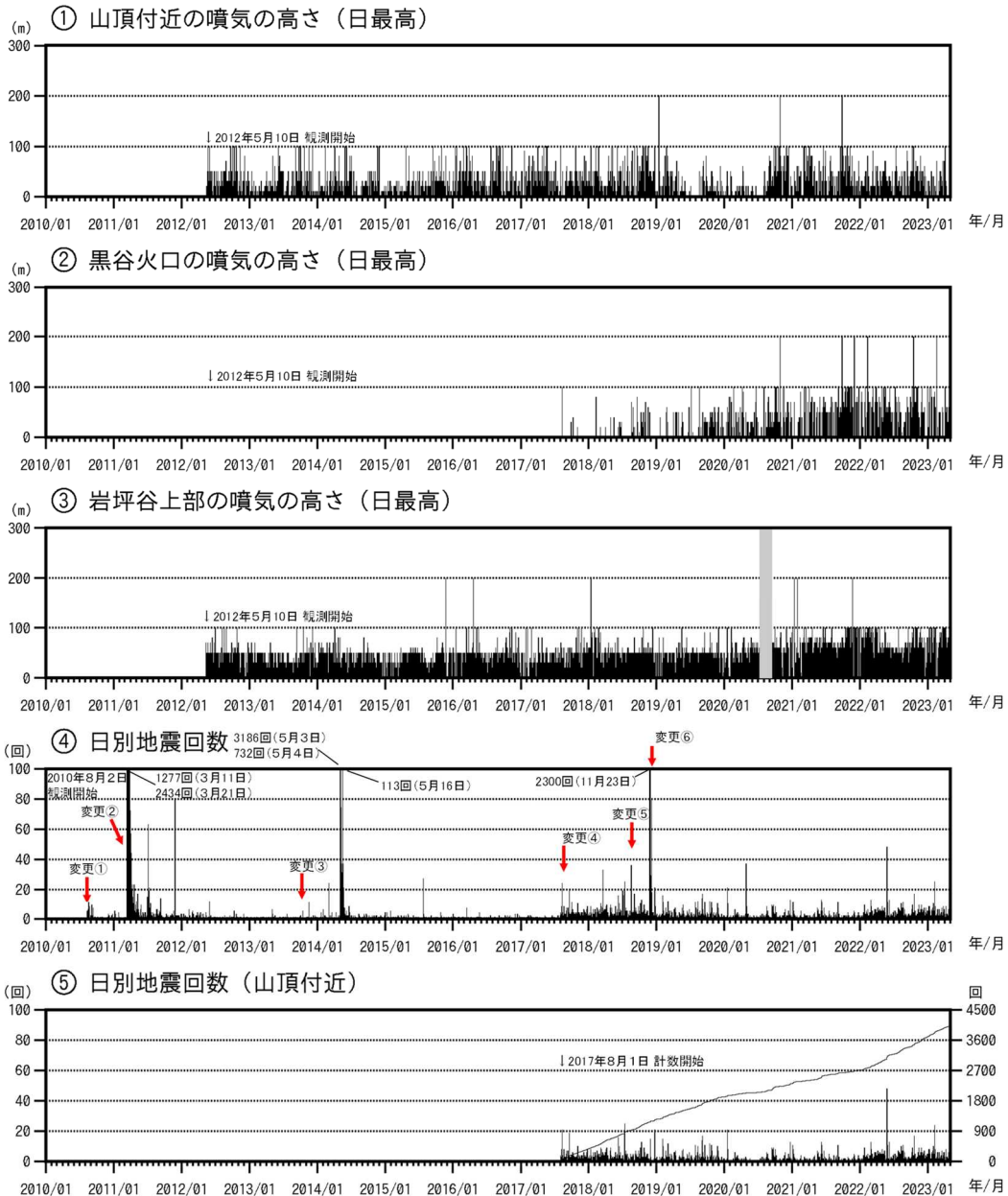
図5 焼岳 噴気の高さと地震回数の推移(2010年8月2日～2023年4月30日)
