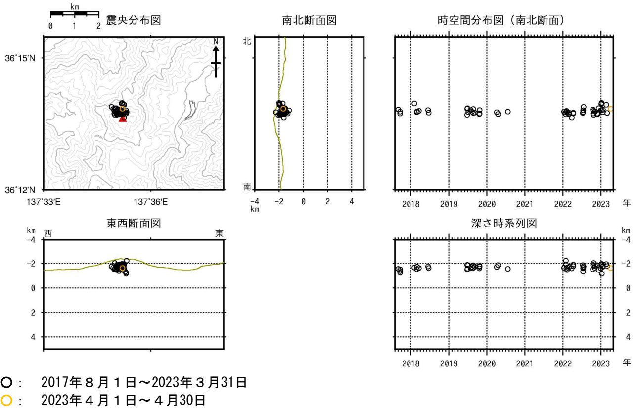
図2 焼岳 山頂付近の地震の震源分布図（2017年8月1日～2023年4月30日）
