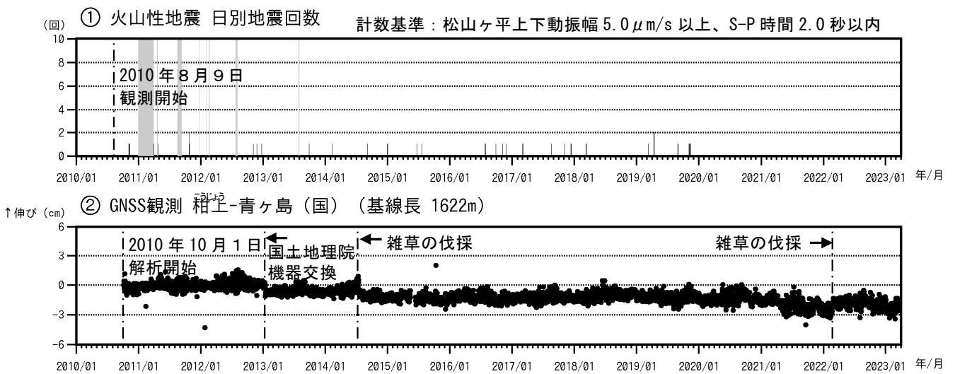
図3 青ヶ島 火山活動経過図（2010年8月9日～2023年3月31日）
