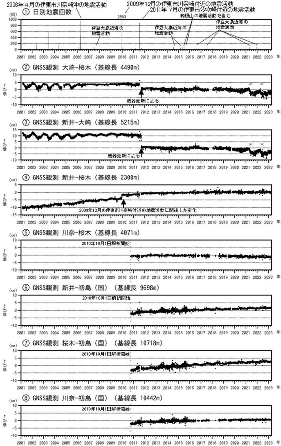
図3 伊豆東部火山群 火山活動経過図 (2001年2月1日~2023年3月31日)
