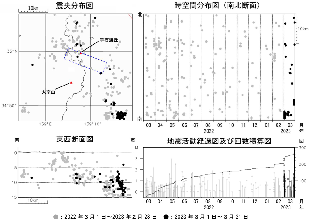
図2 伊豆東部火山群 広域地震観測網による震源分布図（2022年3月1日～2023年3月31日） □の領域は群発地震活動の発生する可能性がある範囲（火口が出現する可能性のある範囲）を示しています。 ( https://www.data.jma.go.jp/vois/data/tokyo/STOCK/level/PDF/level_316.pdf ) 広域地震観測網により震源決定したもので、深さは全て海面以下として決定しています。 M（マグニチュード）は地震の規模を表し、M0.0以上を表示しています。 図中の震源要素は一部暫定値が含まれており、後日変更することがあります。 この図では、関係機関の地震波形を一元的に処理し、地震観測点の標高を考慮する等した手法で得られた震源を用いています。
