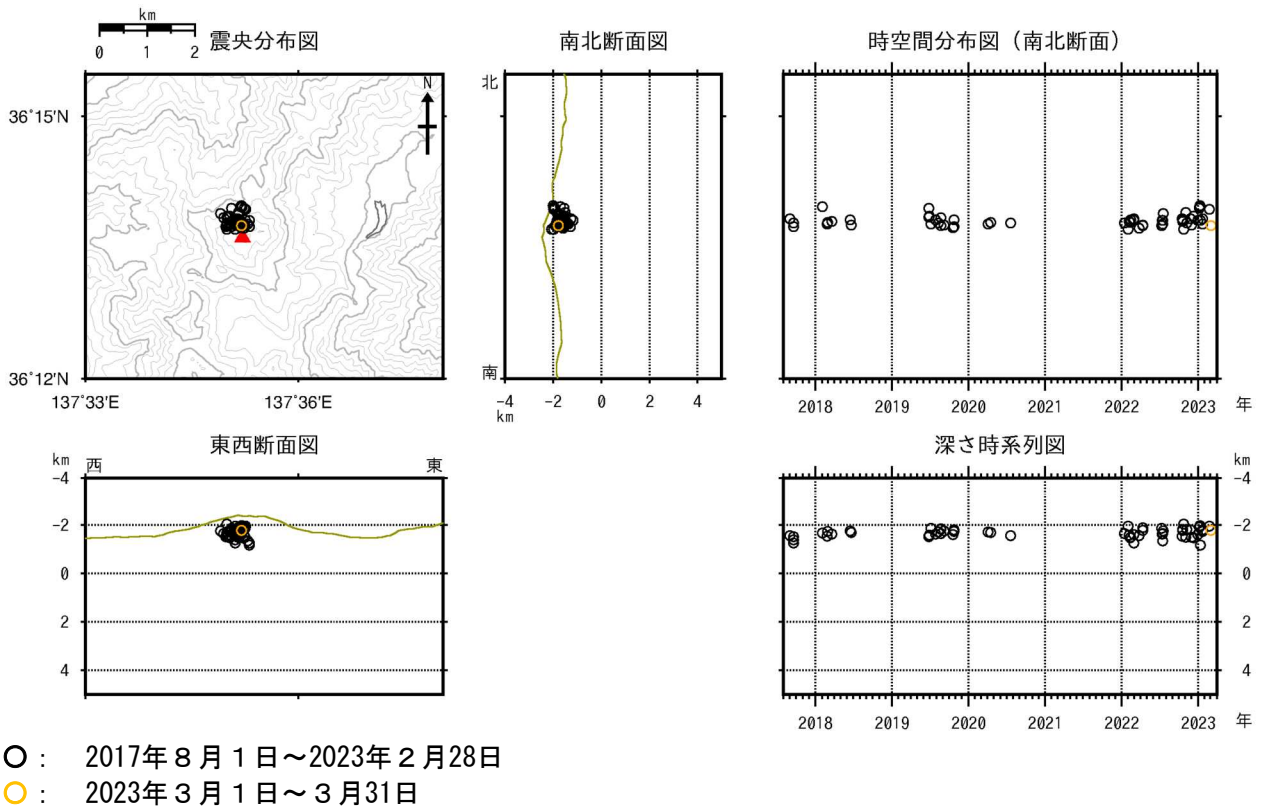
図2 焼岳 山頂付近の地震の震源分布図（2017年8月1日～2023年3月31日）
