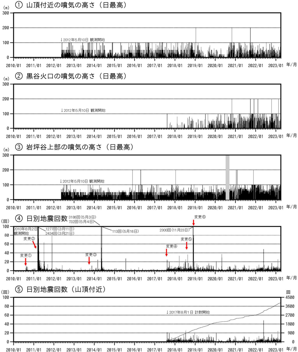
図5 焼岳 噴気の高さと地震回数の推移(2010年8月2日～2023年3月31日)
