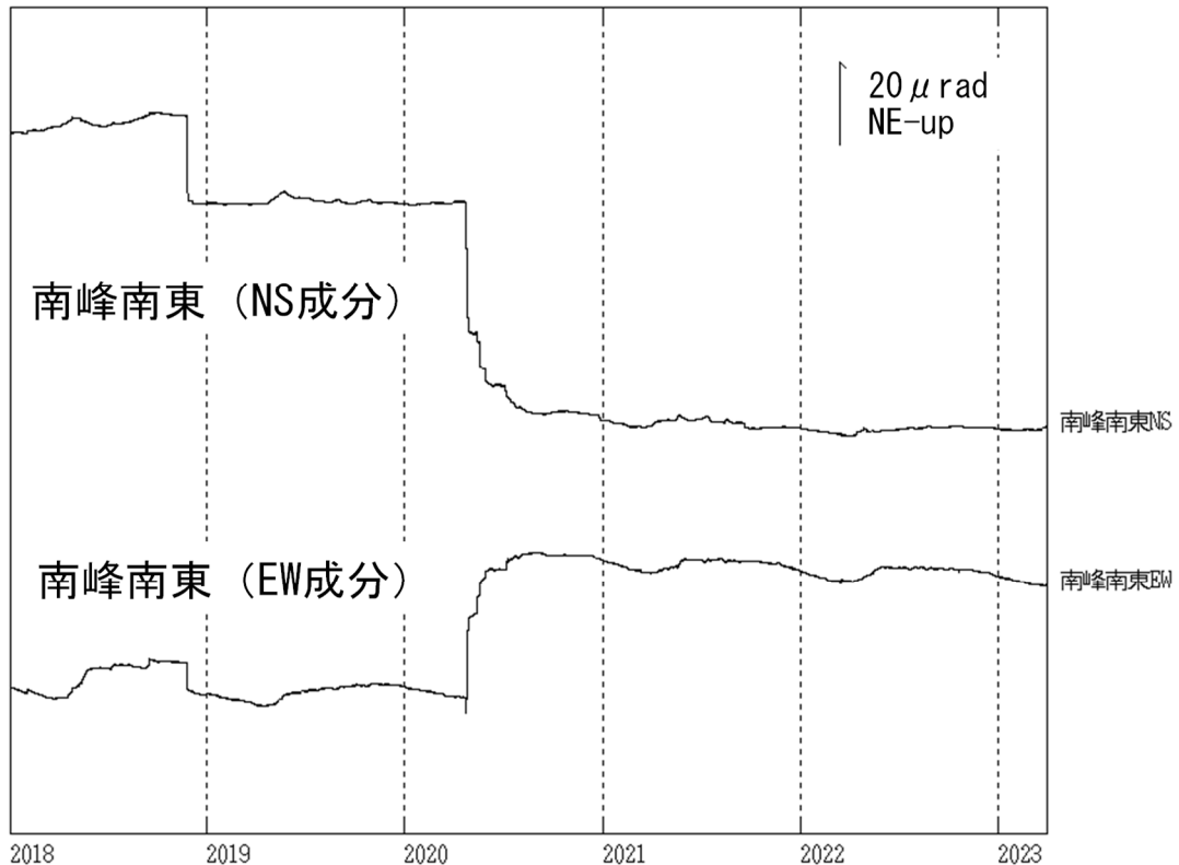
図8 焼岳 南峰南東観測点における傾斜データ（2018年1月1日～2023年3月31日）
