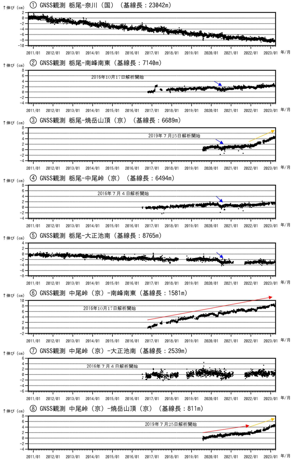
図6 焼岳 GNSS 連続観測による基線長変化 (2010年10月1日~2023年3月31日)
