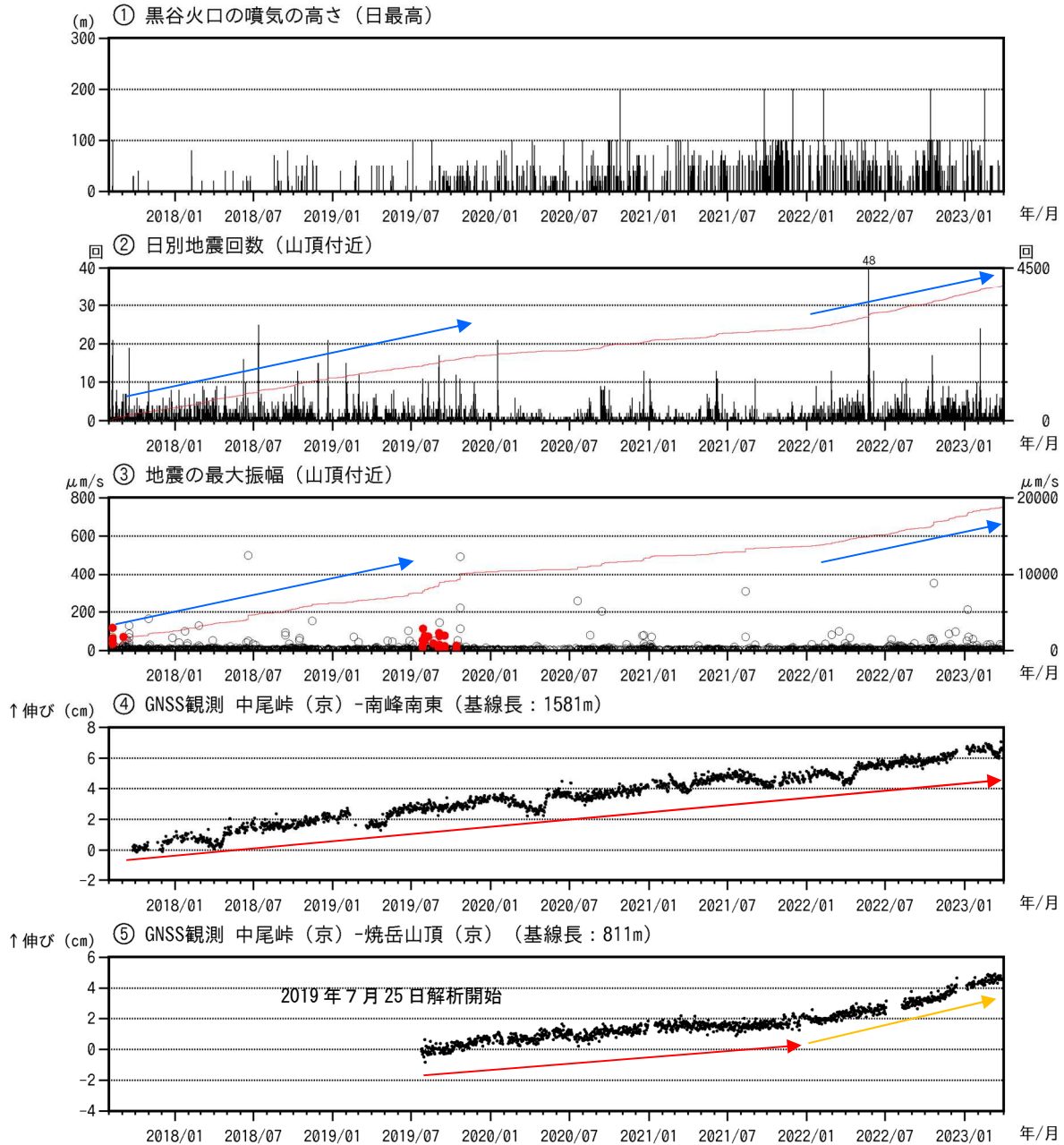
図1 焼岳 火山活動経過図（2017年8月1日～2023年3月31日）
