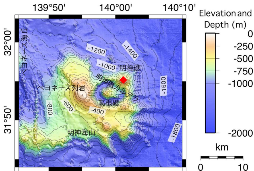
図3 ベヨネース列岩付近の海底地形図と変色水確認地点（◆）
