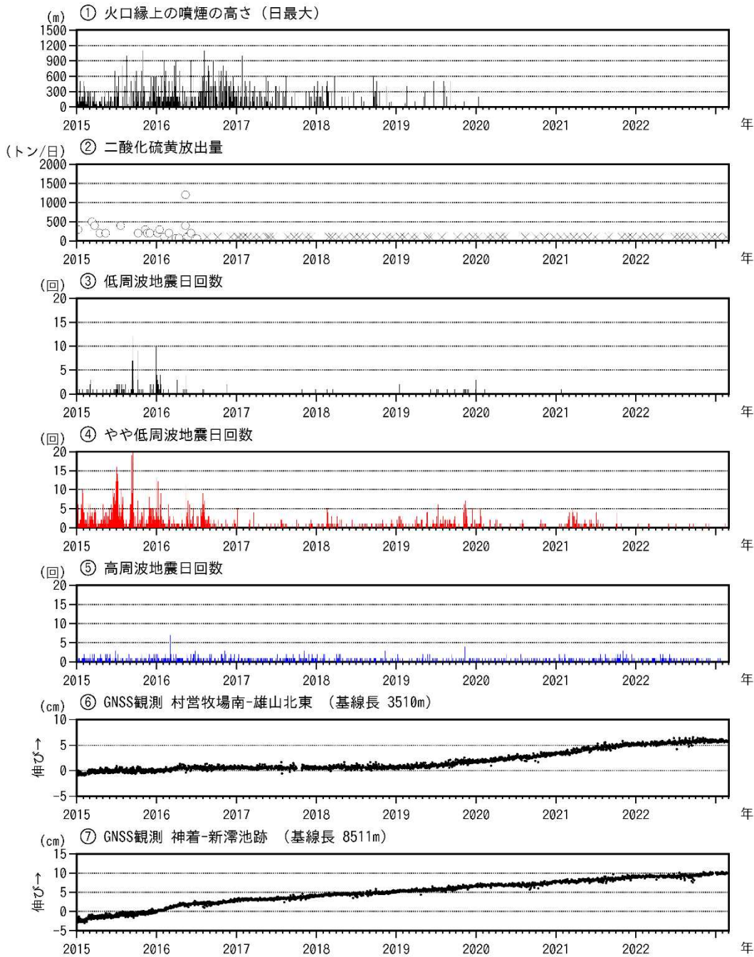
図6 三宅島 火山活動経過図（2015年1月1日～2023年2月28日）
