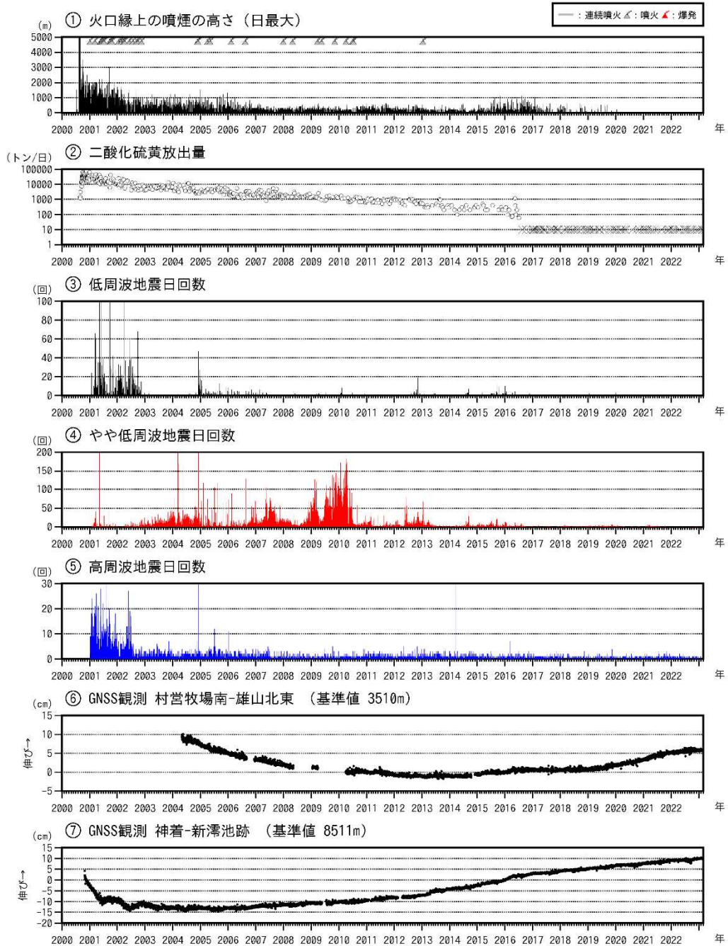
図7 三宅島 長期の火山活動経過図（2000年1月1日～2023年2月28日）
