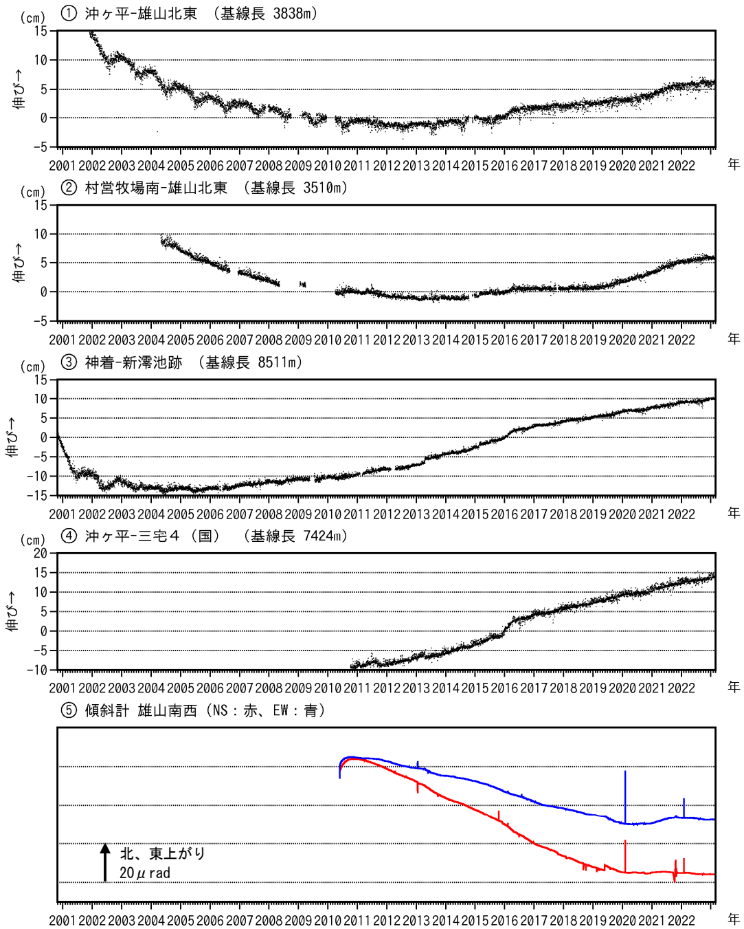
図8 三宅島 GNSS 連続観測及び傾斜計観測結果（2000年10月26日～2023年2月28日）
