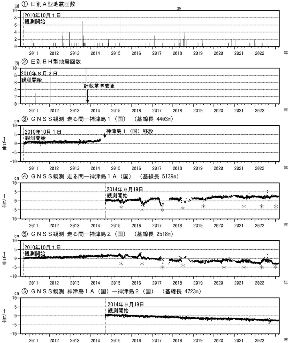
図2 神津島 火山活動経過図(2010年8月2日～2023年2月28日)
