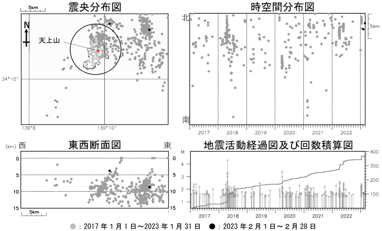
図3 神津島 広域地震観測網による山体・周辺の地震活動（2017年1月1日～2023年2月28日） 広域地震観測網により震源決定したもので、深さは全て海面以下として決定しています。 M（マグニチュード）は地震の規模を表し、M1.4以上の地震を示しています。 図中の震源要素は一部暫定値が含まれており、後日変更することがあります。 計数対象（天上山西から半径約5km、深さ約15km以内）以外の地震が含まれるため、図2-①の日別A型地震回数とは異なります。 震央分布図中の円は火山性地震の回数の計数対象（天上山西から半径5km、深さ15km以内）の範囲を示しています。 この図では、関係機関の地震波形を一元的に処理し、地震観測点の標高を考慮する等した手法で得られた震源を用いています（ただし、2020年8月以前の地震については火山活動評価のための参考震源です）。
